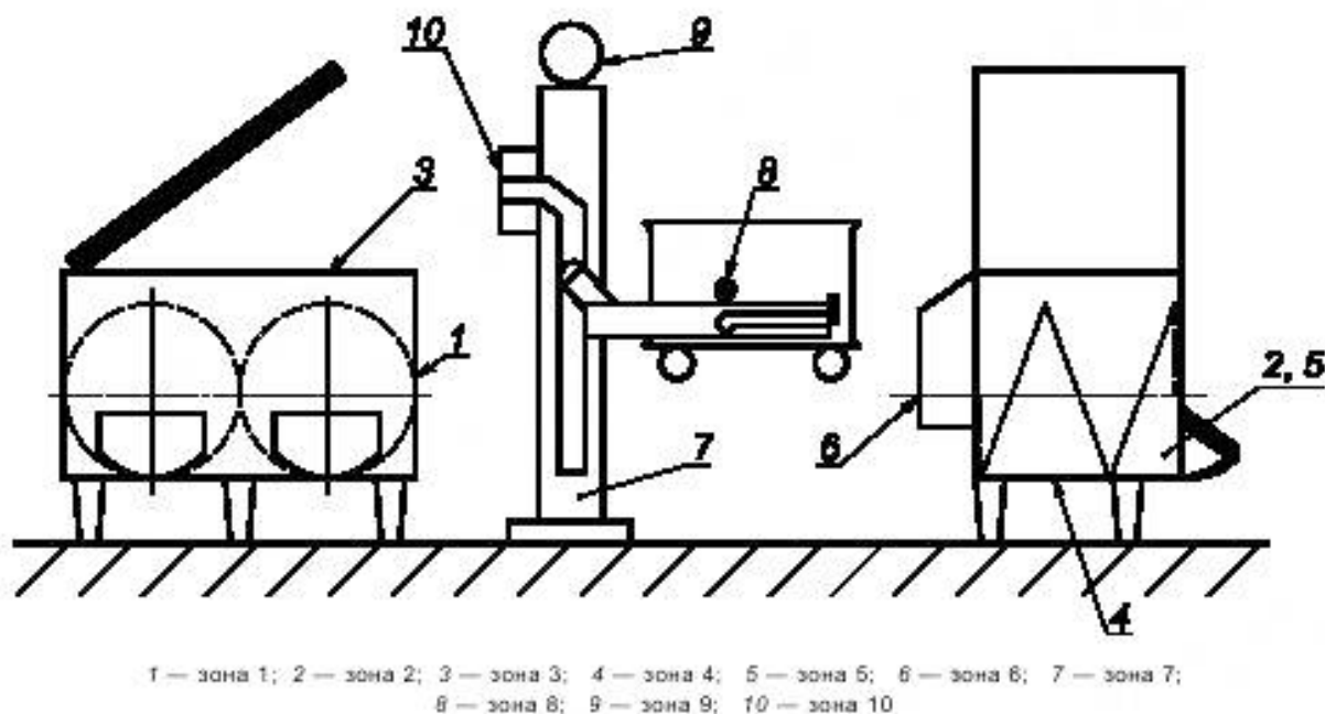
Рисунок 5 — Опасные зоны фаршемешалки
