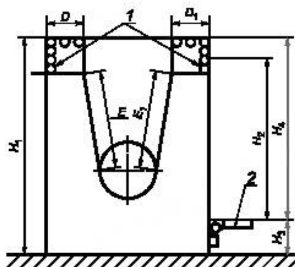
1 — перемещаемое защитное ограждение; 2 — блокирующая ступенька
