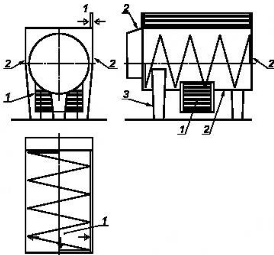
Рисунок 14 — Гигиенические зоны фаршемешалки с выгрузочным люком в донной части
