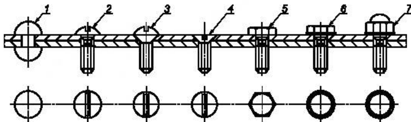
1 — заклепка с полукруглой головкой; 2 — винт с полукруглой головкой; 3 — винт с полукруглой головкой с шлицем; 4 — винт с лоточной головкой с шлицем; 5 — болт с шестигранной головкой; 6 — болт с шестигранной головкой с коническим подголовком; 7 — винт с шестигранной выпуклой головкой
