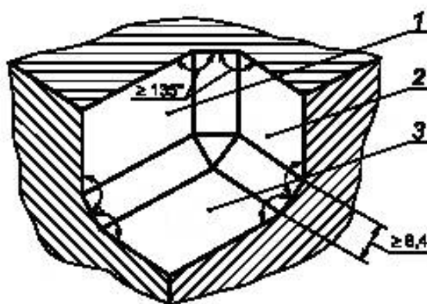
1, 2, 3 — поверхности А, Б, В
