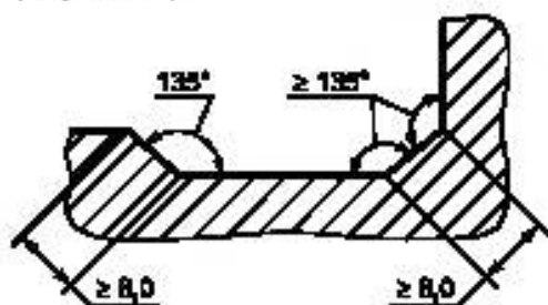
Рисунок А.3 — Углы в пищевой зоне
