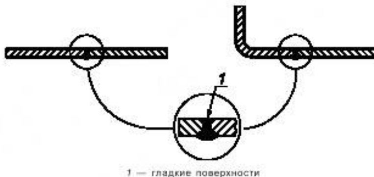
Рисунок А.1 — Гладкие поверхности в пищевой зоне
