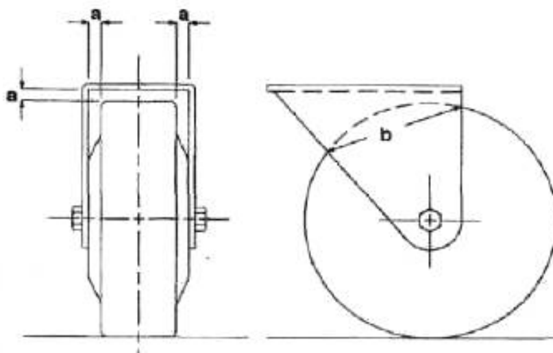
Рисунок А.6 – Пример ролика (колеса) роляного типа, доступного для очистки
