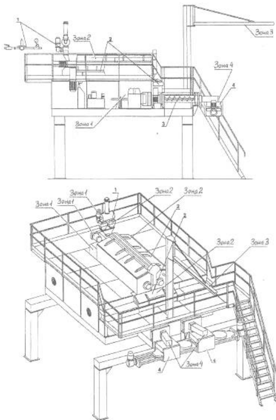
1 – дозирующее устройство; 2 – тестосмеситель; 3 – прессующее устройство; 4 – формующее устройство
