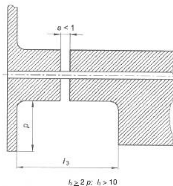
Рисунок А.7 — Шарнирное соединение
