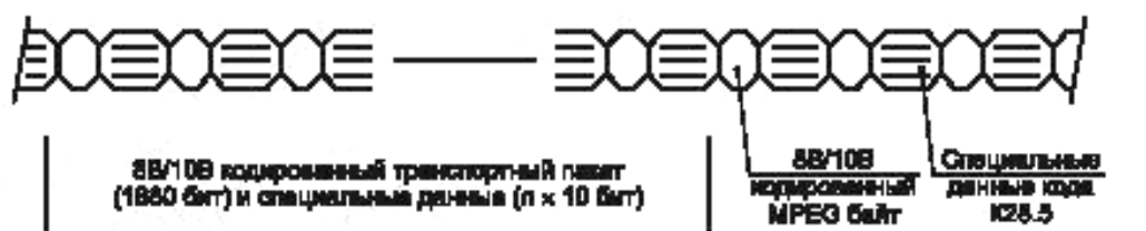
Рисунок 22 — Формат передачи отдельных байт
