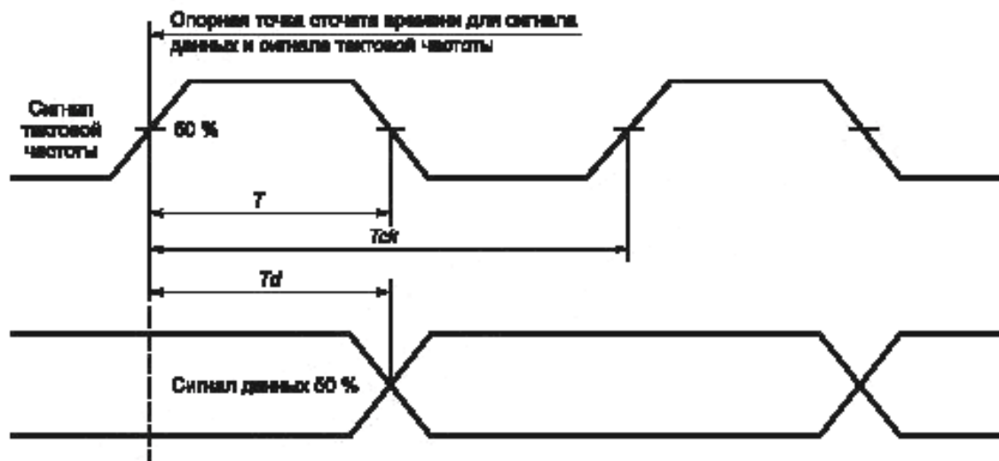
T — длительность импульса синхронизации; T_d — интервал времени передачи данных; T_{ck} — период тактовой частоты; T_{ck} = 2T_d
