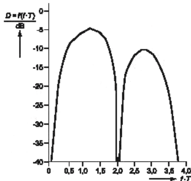
Рисунок 13 — Спектральные плотности инверсного биполярного кода БВН
