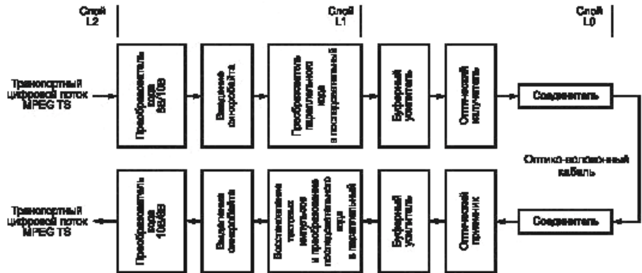
Рисунок 17 — Стекло-волоконная последовательная асинхронная линия передачи
