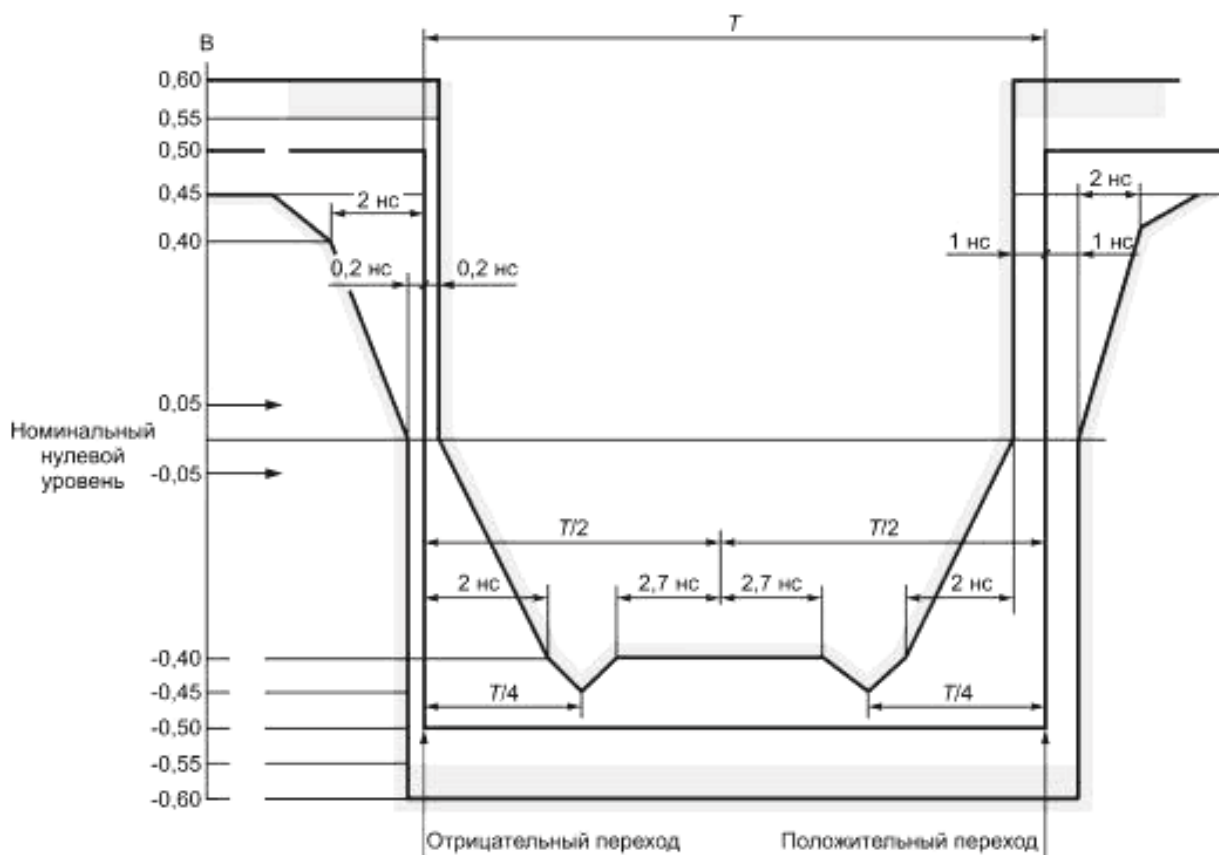
Рисунок 14 — Маска для импульса логического нуля
