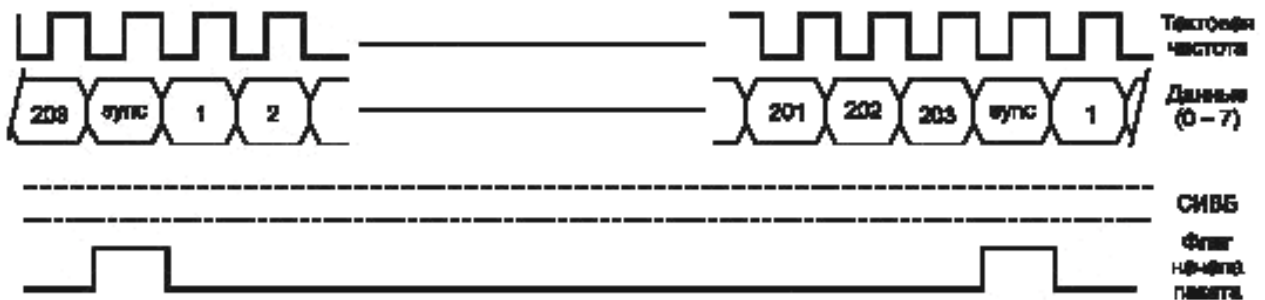
Рисунок 6 — Формат передачи пакетов с кодированием Рида-Соломона (204 байта)
