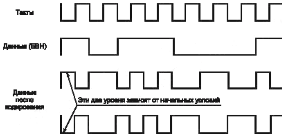
Рисунок 12 — Кодирование инверсным биполярным кодом БВН
