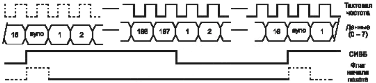
Рисунок 5 — Формат передачи пакетов 204 байта
