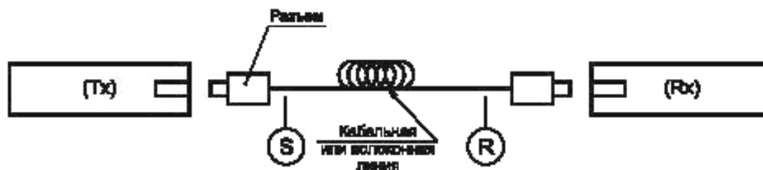
Рисунок 18 — Опорные точки последовательной линии слоя L0
