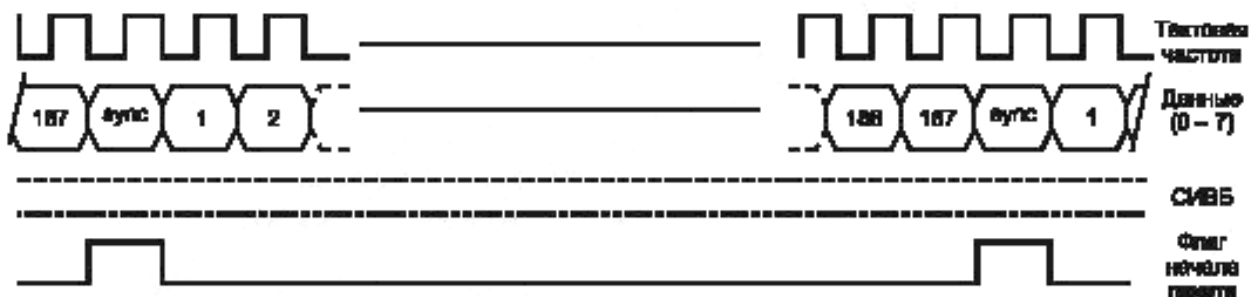
Рисунок 4 — Формат передачи пакетов 188 байт
