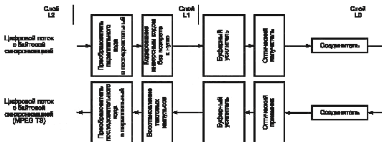
Рисунок 11 — Система передачи с последовательным синхронным интерфейсом при использовании опτικο-волоконного кабеля
