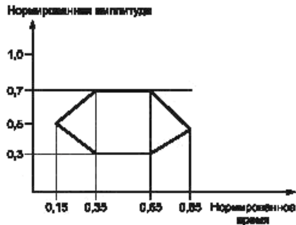
Рисунок 20 — Маска глазовой диаграммы передатчика при измерении джиттера
