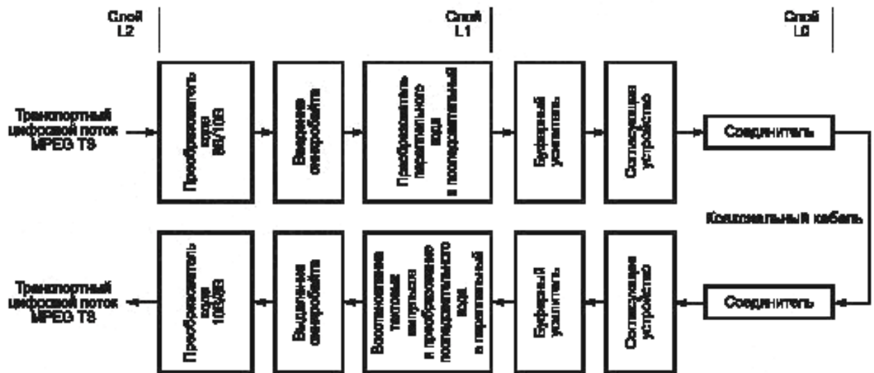
Рисунок 16 — Коаксиальная последовательная асинхронная линия передачи
