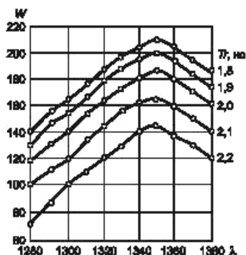
Рисунок 23 — Ширина спектра передатчика
