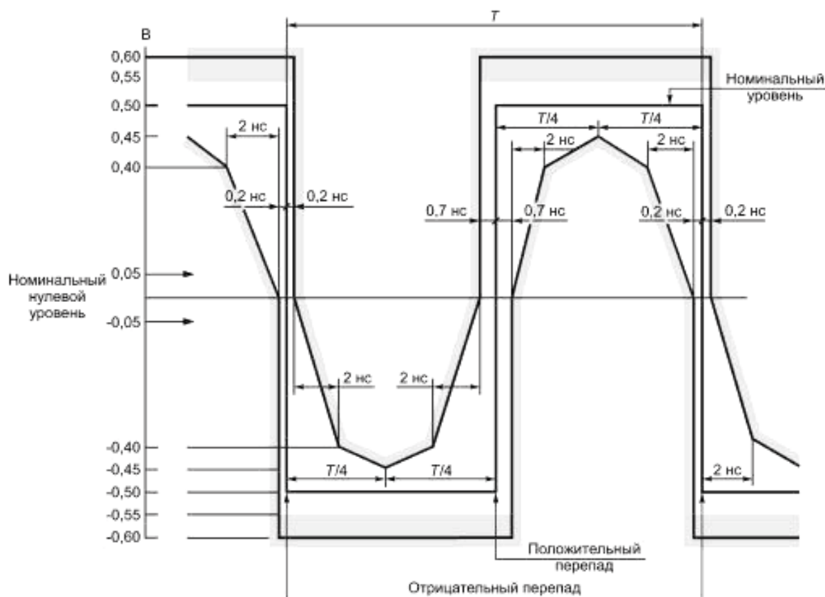
Рисунок 15 — Маска для логической единицы
