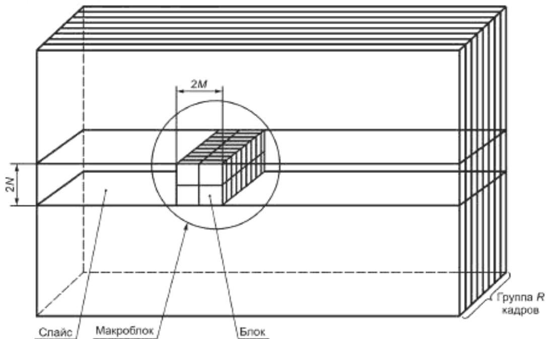
Рисунок Г.1 — Структурные элементы кодирования EVC
