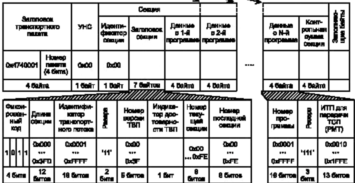
Рисунок 16 — Транспортный пакет с секцией ТВП (PAT)
