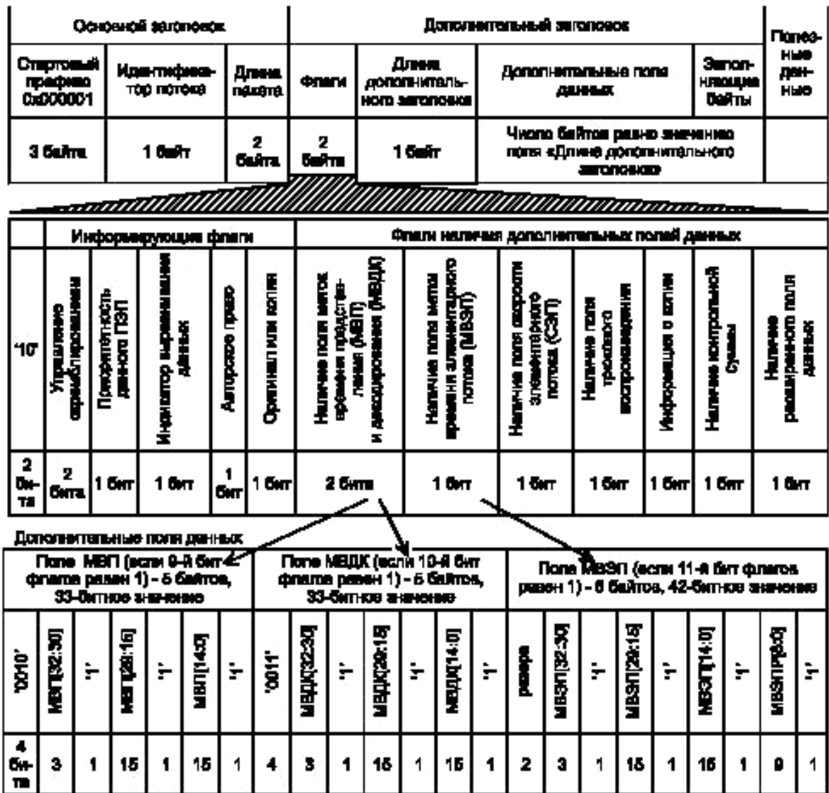
Рисунок 4 — Детализированная структура пакета ПЭП
