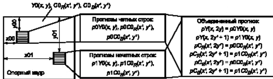
Рисунок А.11 — Формирование полевого прогноза P -макроблока
