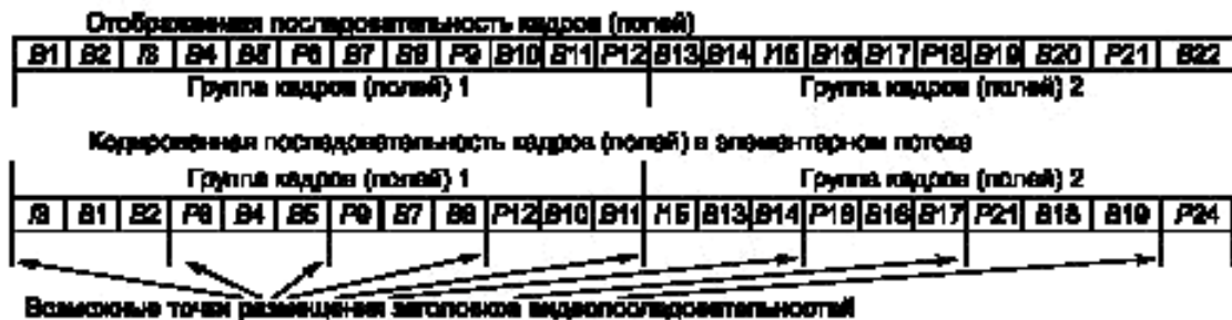
Рисунок А.16 — Отображаемая и кодируемая последовательность кадров
