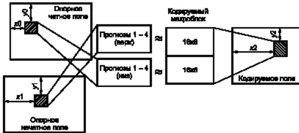
Рисунок А.12 — Формирование прогноза типа «компенсация движения 16x8» для P-поля
