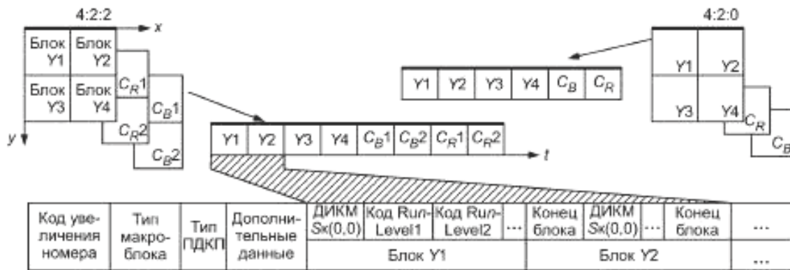
Рисунок А.8 — Результат кодирования I-макроблока
