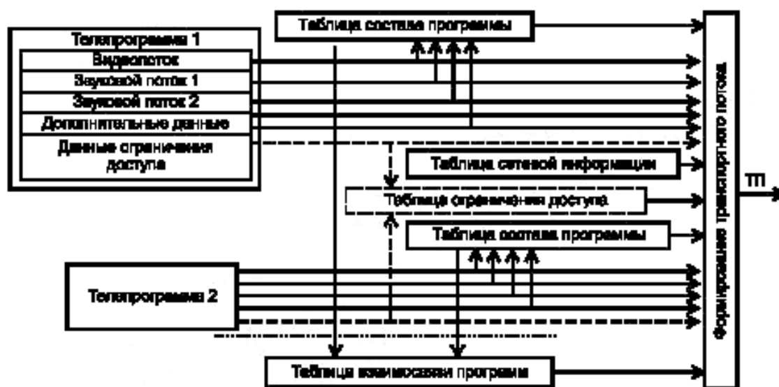
Рисунок 13 — Взаимосвязь элементов ПЗИ и телепрограмм
