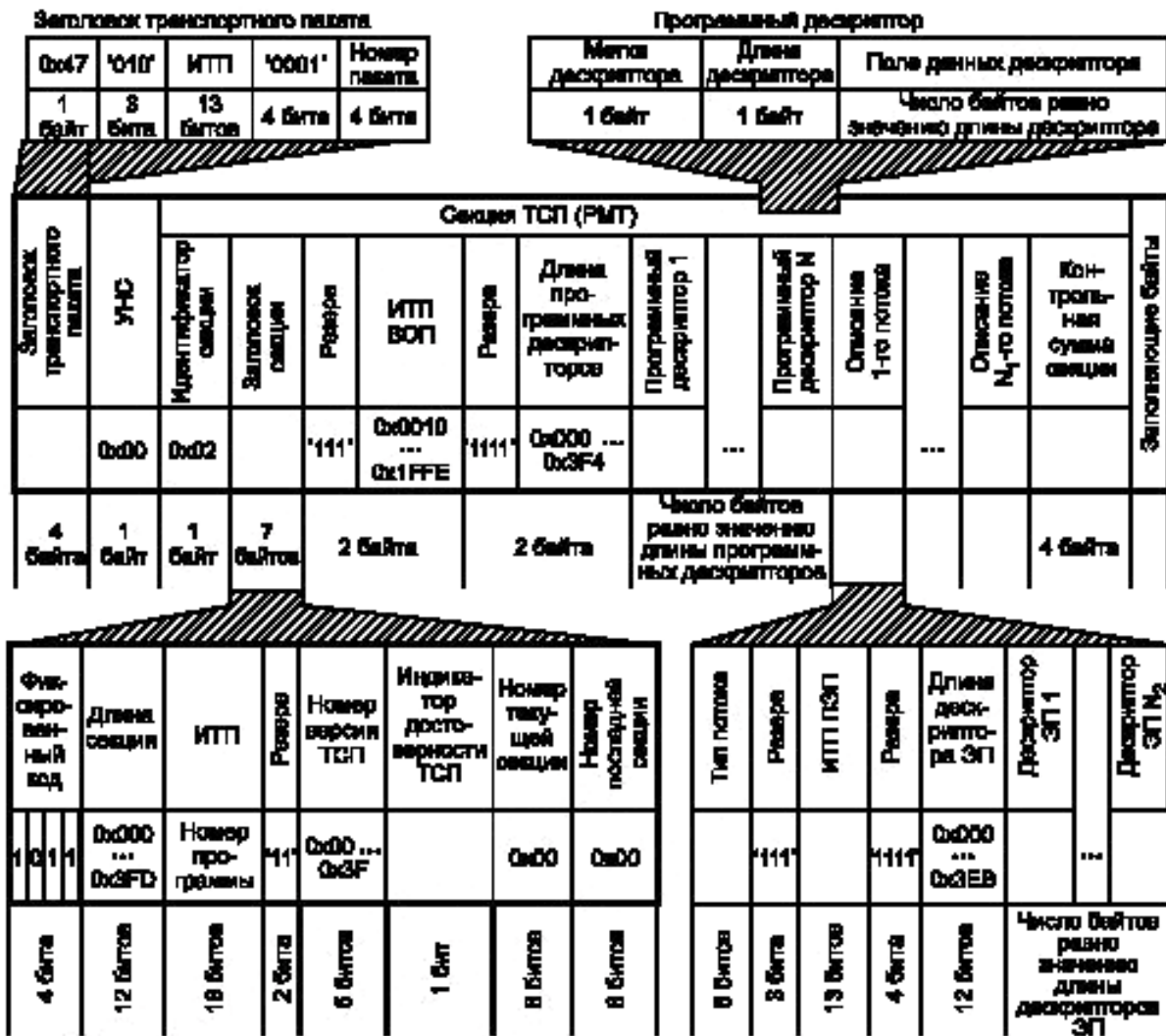
Рисунок 19 — Транспортный пакет с секцией ТСП (PMT)
