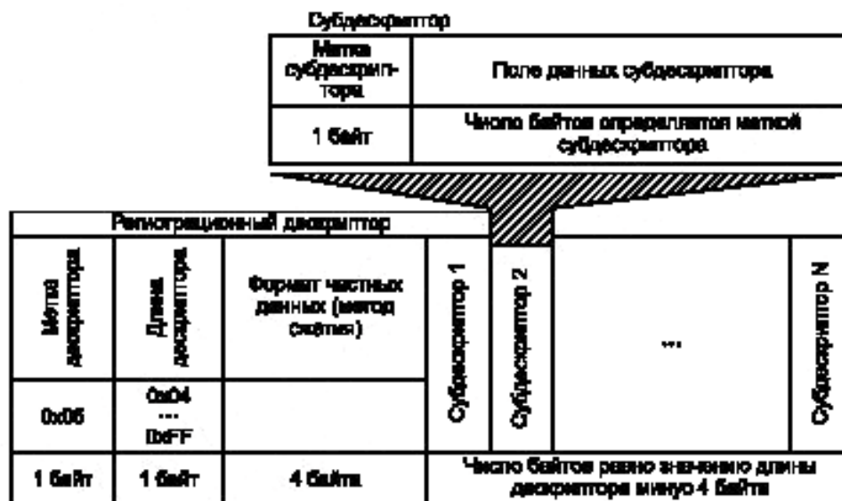
Рисунок 20 — Регистрационный дескриптор, содержащий N субдескрипторов
