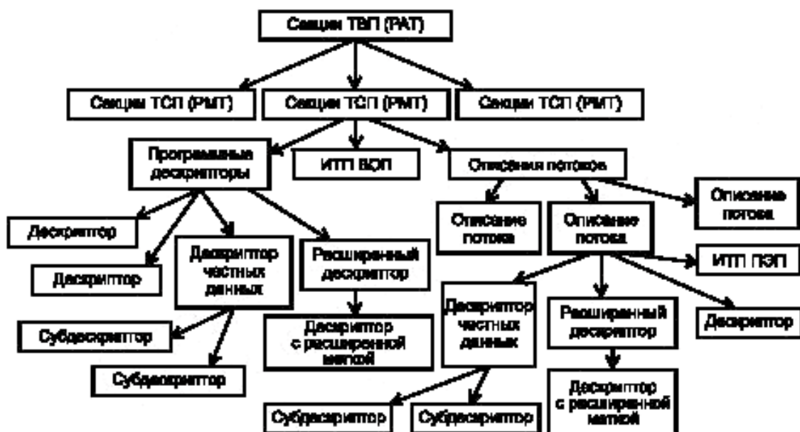
Рисунок 21 — Иерархия элементов служебной информации ТВП (PAT) и ТСП (PMT)
