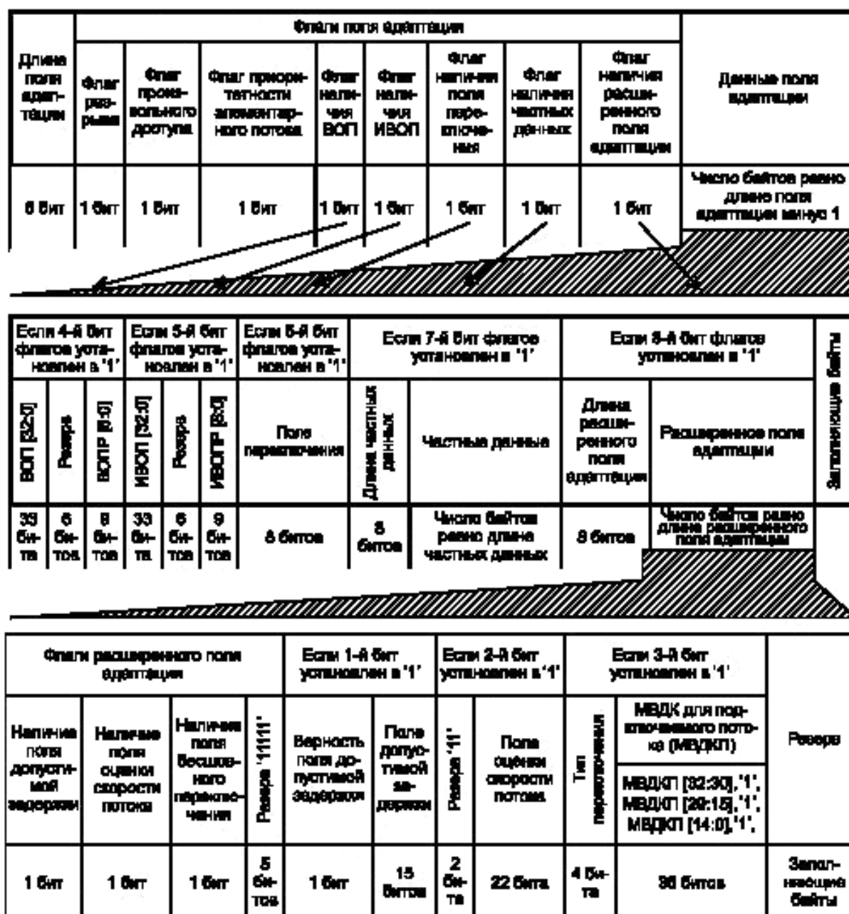
Рисунок 12 — Структура поля адаптации транспортного пакета
