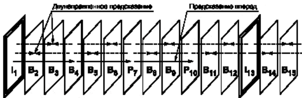
Рисунок A.14 — Виды межкадровых предсказаний
