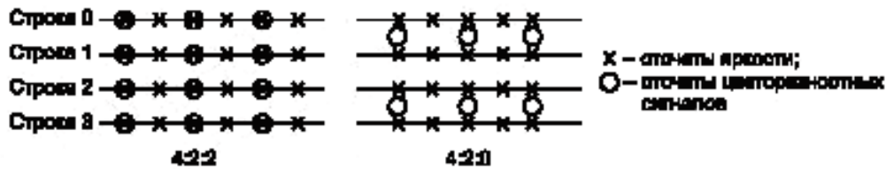
Рисунок А.2 — Форматы субдискретизации цвета 4:2:2 и 4:2:0
