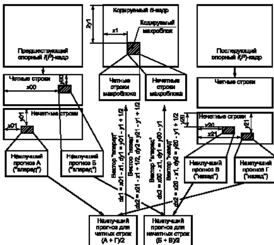
Рисунок А.15 — Формирование полевого прогноза для B-макроблока
