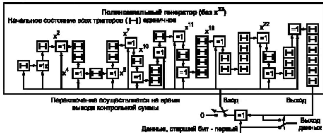
Рисунок 17 — Вычисление контрольной суммы в формирователе ТВП (PAT)
