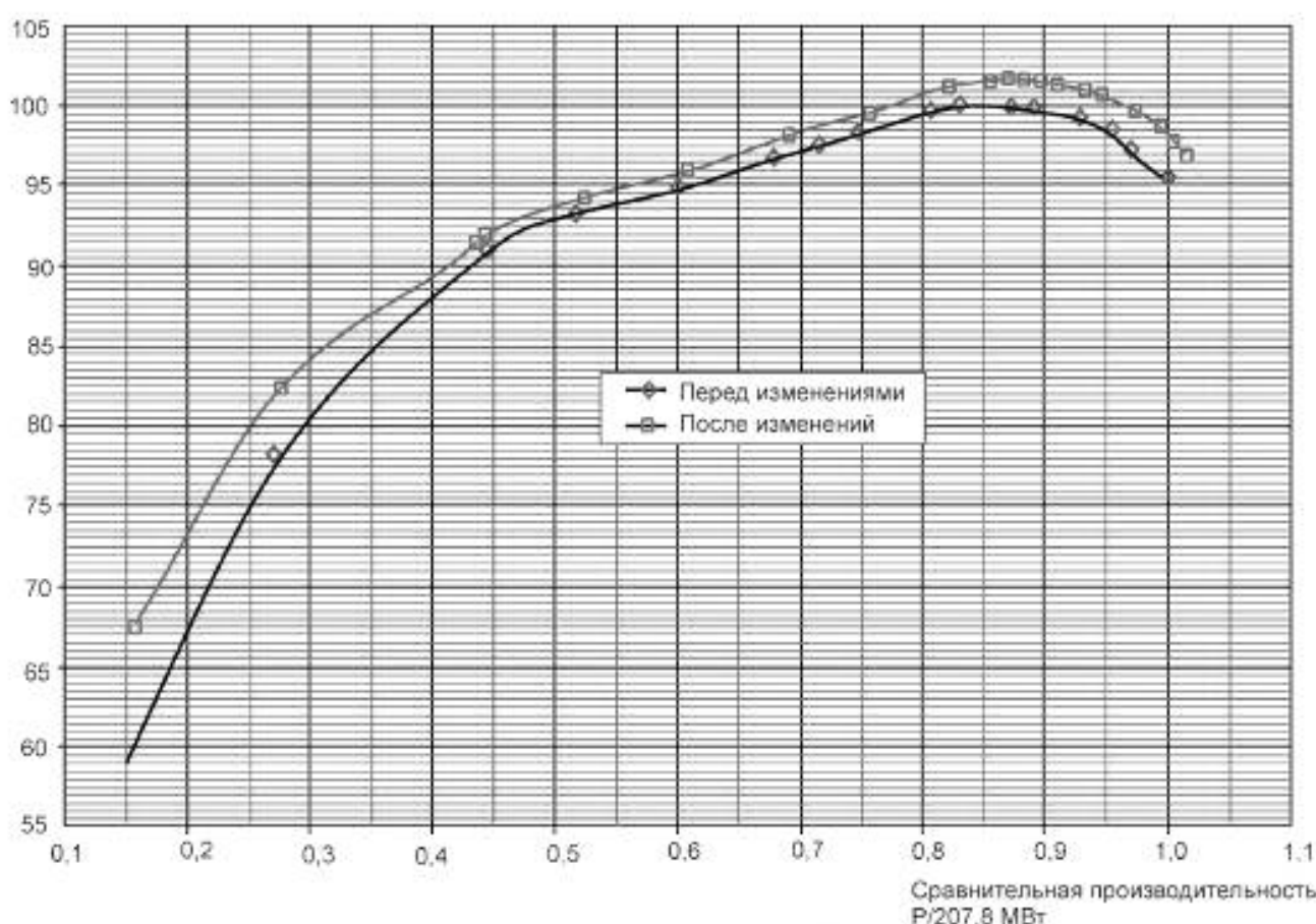
Рисунок 6 — Сравнительный прирост эффективности после изменения лопастей на рабочем колесе LA Grande 3, Квебек, Канада
