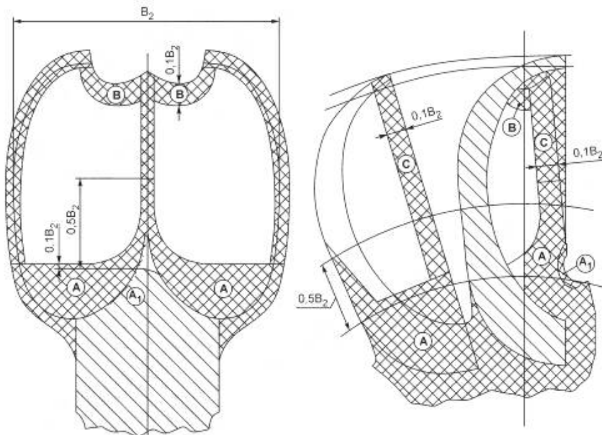
Рисунок 2 — Критические зоны для трещин А и В в лопастях рабочего колеса турбины Пельтона
