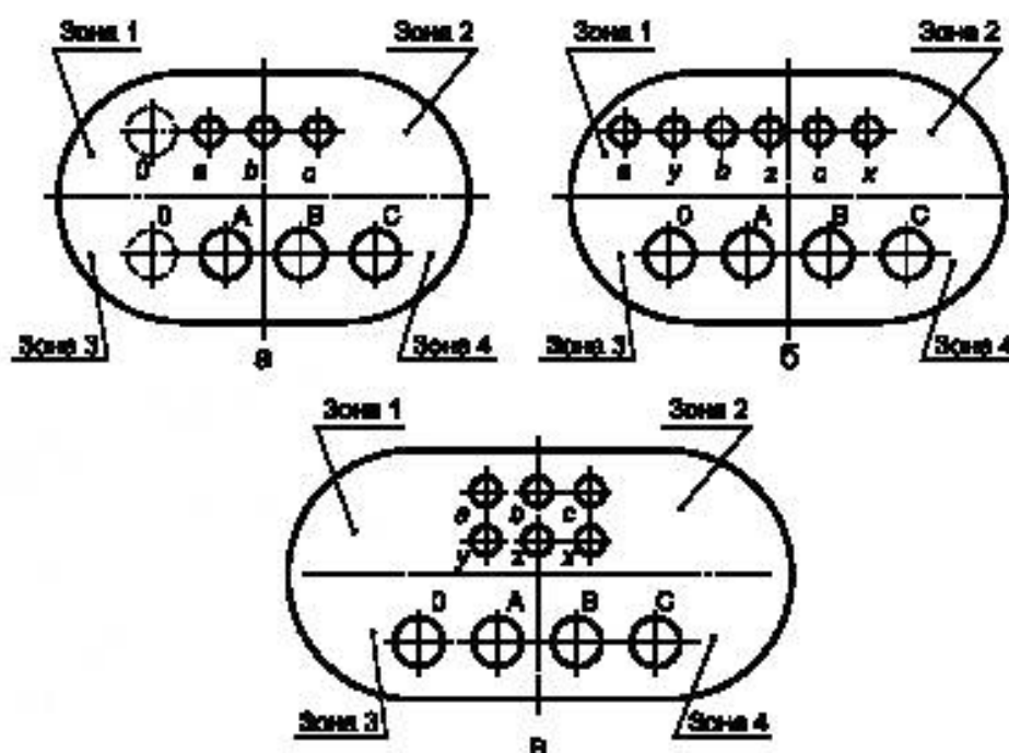
Рисунок 1 — Двухобмоточные трансформаторы
