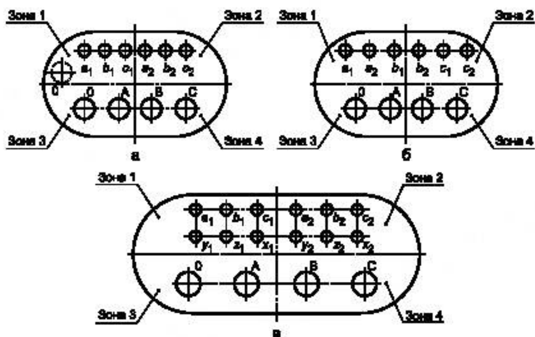
Рисунок 2 — Двухобмоточные трансформаторы с расщепленной обмоткой НН
