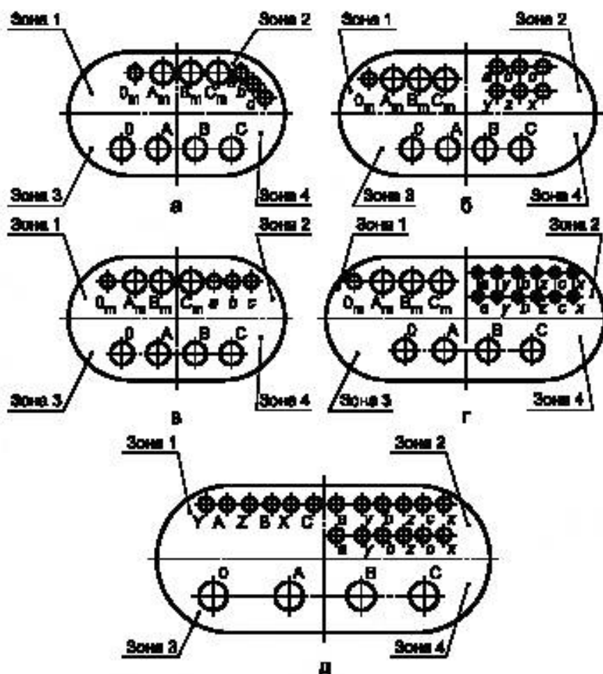
Рисунок 3 — Трехобмоточные трансформаторы
