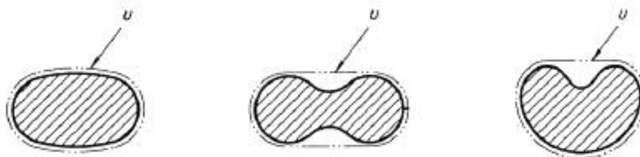
Рисунок 6 – Примеры некруглой вводимой части
