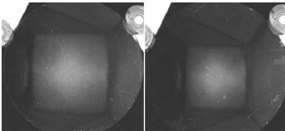
Рисунок Н.2 – Примеры линз, выдержавших испытание («линза проходит»)
