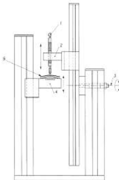
Рисунок J.2 – Пример испытательной установки
