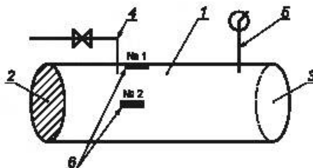
1 — отрезок трубопровода; 2, 3 — герметичные заглушки; 4 — штуцер; 5 — манометр; 6 — зоны измерений (№ 1 и № 2)
