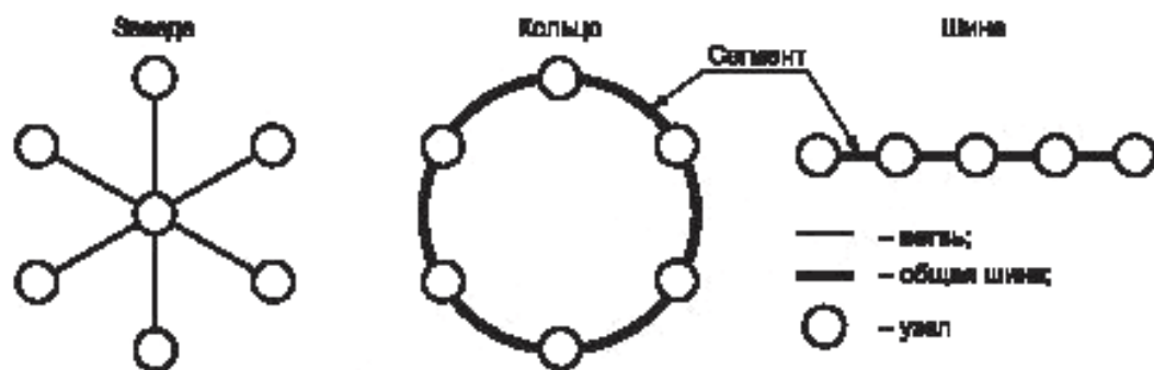
а) Топологии активных сетей
