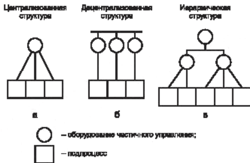
Рисунок А.5 — Примеры структур управления
