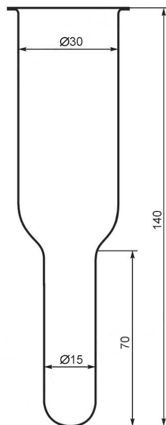
Рисунок 20 — Ампула
