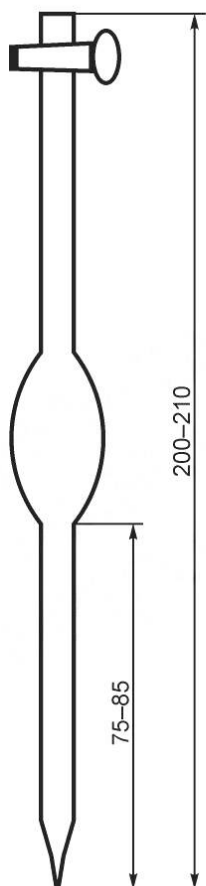
Рисунок 19 — Пипетка для отбора проб
