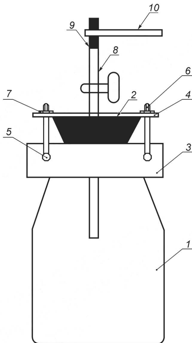
1 — толстостенная склянка вместимостью 250 см 3 ; 2 — резиновая пробка № 22 с отверстием; 3 — полумуфта (хомут) высотой 17 мм; 4 — держатель пробки; 5 — болты для крепления полумуфты болтом и гайкой; 6 — болты для крепления держателя пробки; 7 — гайки для крепления держателя пробки; 8 — стеклянная трубка диаметром 8 мм с краном; 9 — каучуковая трубка диаметром 8 мм; 10 — зажим Мора
