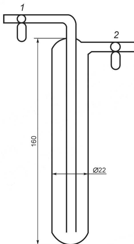
1, 2 — краны или зажимы Гофмана
