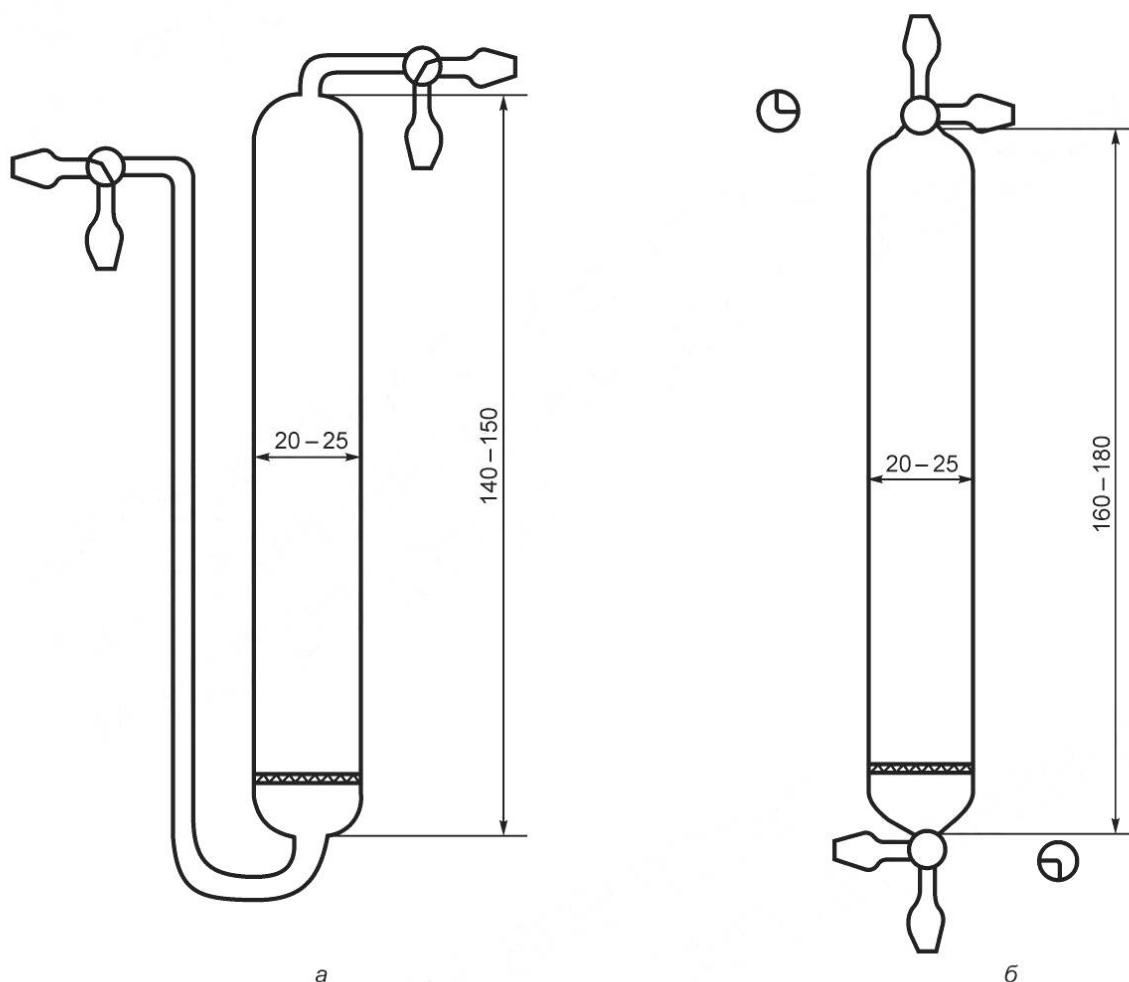
Рисунок 11 — Абсорбционный сосуд
