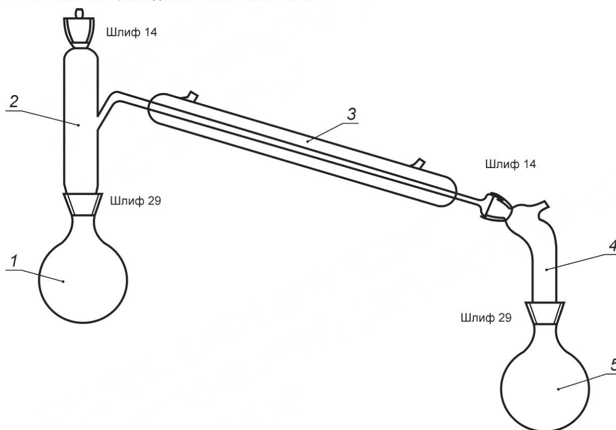
1 — круглодонная колба; 2 — насадка; 3 — холодильник; 4 — алонж; 5 — колба-приемник
