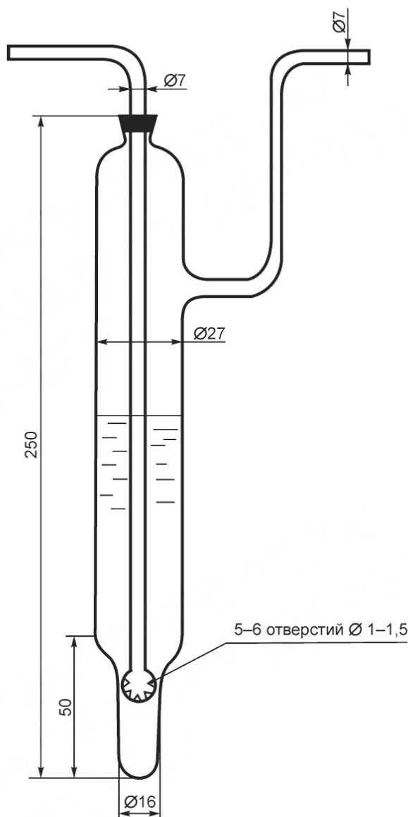
Рисунок 12 — Поглонитель
