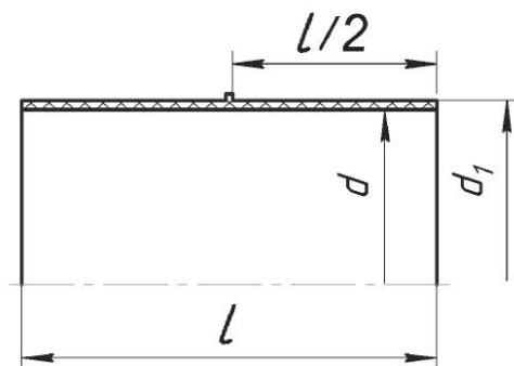
l – длина втулки; d_1 – наружный диаметр; d – внутренний диаметр Рисунок 13 – Основные размеры втулки
