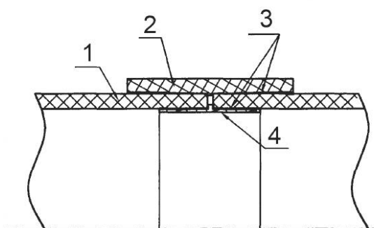
1 – труба; 2 – муфта; 3 – клеевой состав; 4 – втулка
