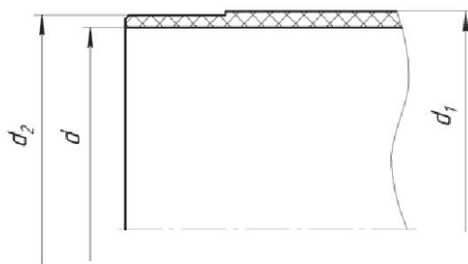
Рисунок 2 – Ниппель под соединение «К» без утолщения
