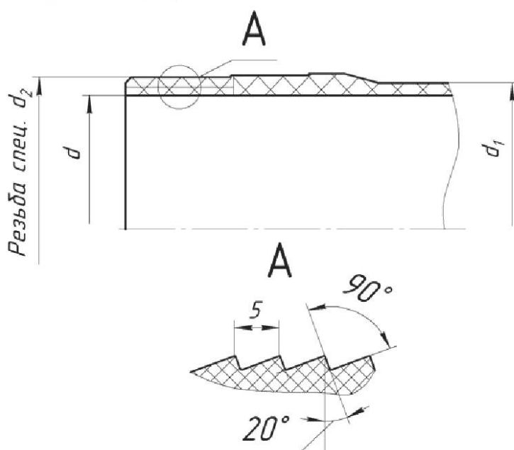
Рисунок 2 – Ниппель под соединение «К» без утолщения
