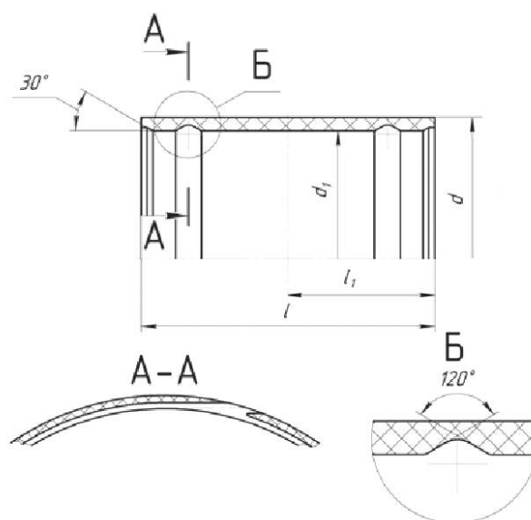
d – наружный диаметр муфты; d_1 – внутренний диаметр муфты; l – длина муфты; l_1 – глубина соединения
