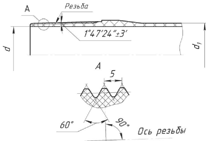
d – внутренний диаметр трубы; d_1 – наружный диаметр трубы Рисунок 5 – Резьбовая концевая часть под соединение «РКН»
