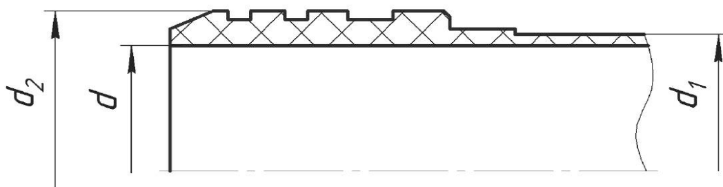
Рисунок 3 – Ниппель под соединение «КРС»
