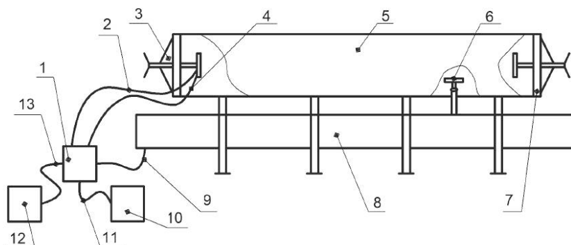
1 – гидропульт; 2 – рукав высокого давления; 3 – опора неподвижная с узлом зажима; 4 – рукав низкого давления; 5 – бронекамера; 6 – люнет опорный; 7 – опора подвижная с узлом зажима; 8 – бак; 9 – рукав циркуляционный; 10 – насос низкого давления; 11 – рукав низкого давления; 12 – насос высокого давления; 13 – рукав высокого давления
