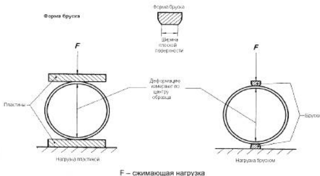
Рисунок 1 – Схема нагружения образца
