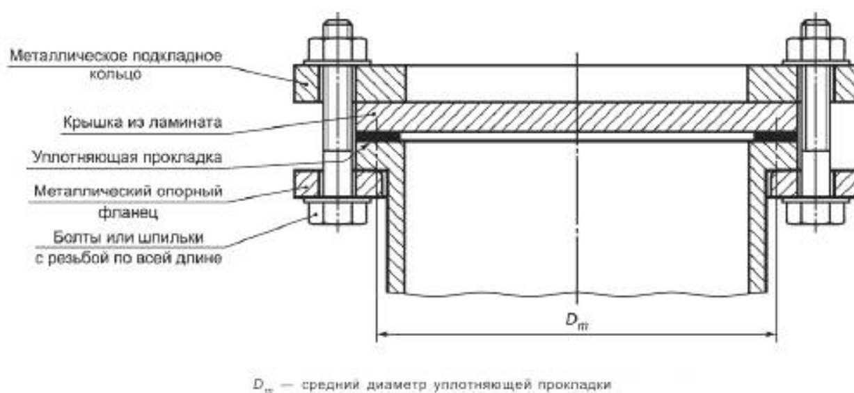
Рисунок Ж.8 — Общий вид глухого фланца: уплотняющая прокладка внутри окружности центров отверстий под болты
