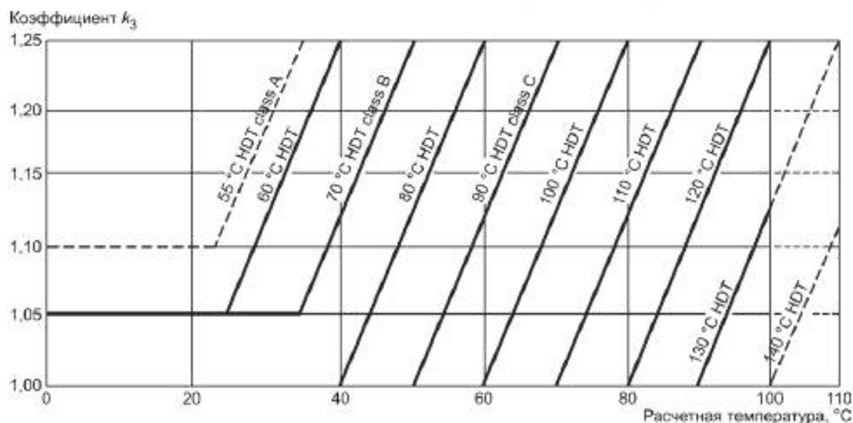
Рисунок А.1 — Коэффициент, соответствующий температуре
