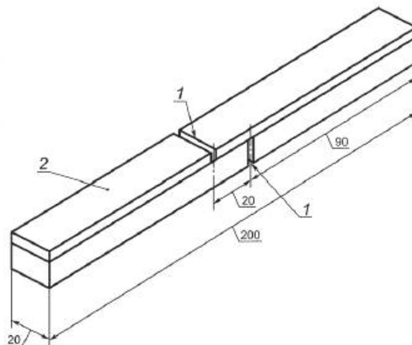
1 — надпил; 2 — термопластичный футеровочный слой
