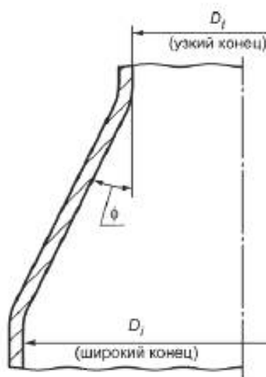
Рисунок Ж.6 — Коническое днище с изгибами
