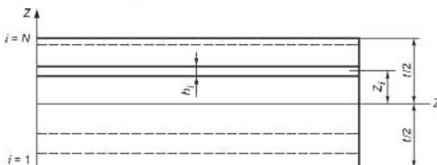
Рисунок П.1 — l слой балки из ламината
