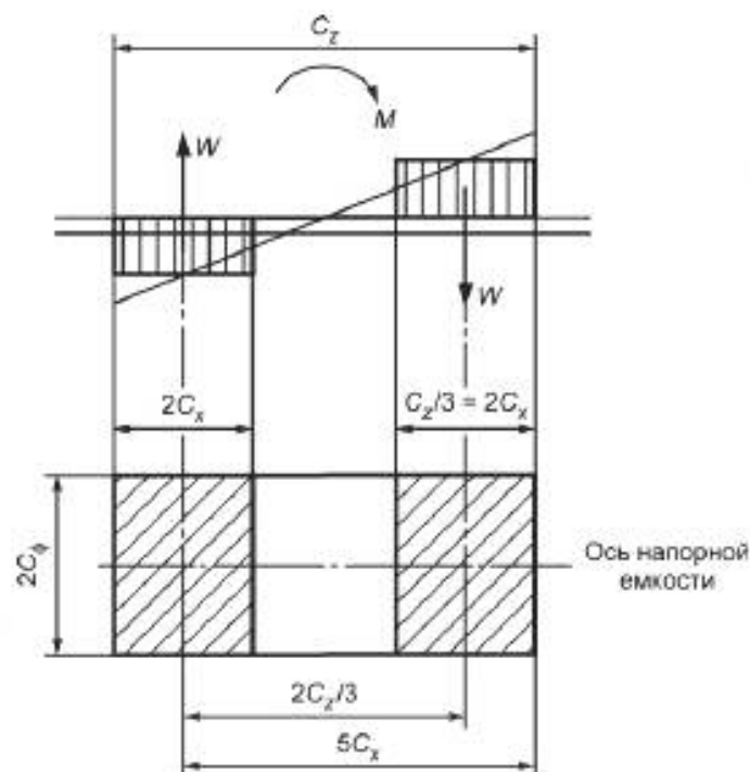
Рисунок У.23 — Продольный момент
