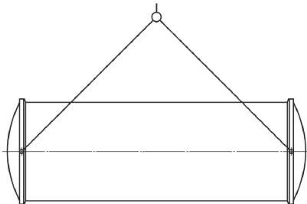
Рисунок 9.1 — Подъем емкости с использованием цепф в горизонтальном положении
