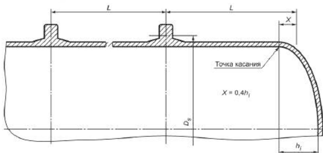
Рисунок В.2 — Цилиндр с ребрами жесткости
