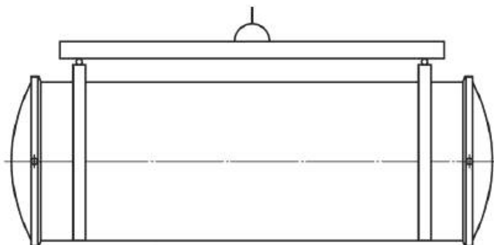
Рисунок 9.2 — Подъем емкости с использованием ремённых чалок в горизонтальном положении
