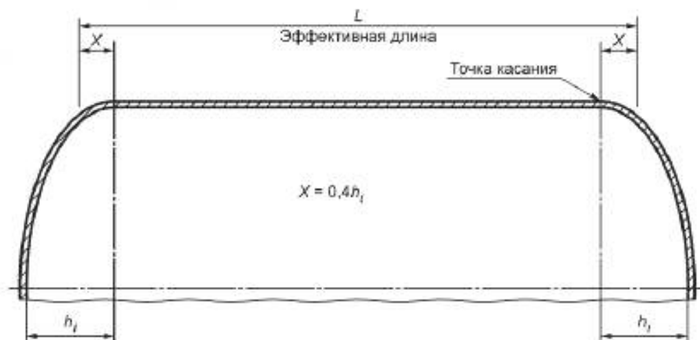
Рисунок В.1 — Цилиндр без ребер жесткости
