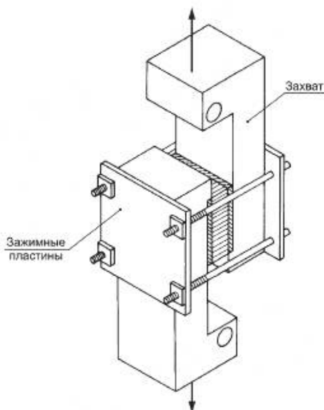
Рисунок 8.3 — Установка образца в захватах
