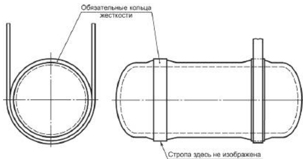
Рисунок М.8 — Стропы
