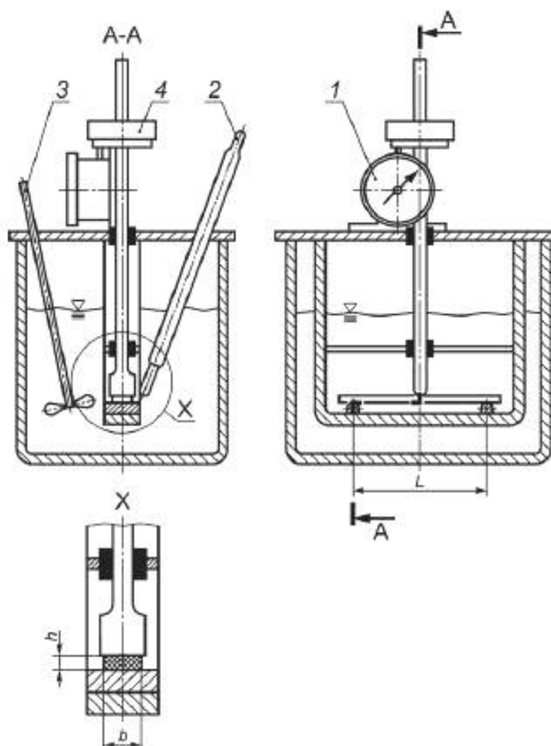
1 — прибор с круговой шкалой; 2 — термометр; 3 — мешалка; 4 — нагрузка; b — ширина испытуемого образца
