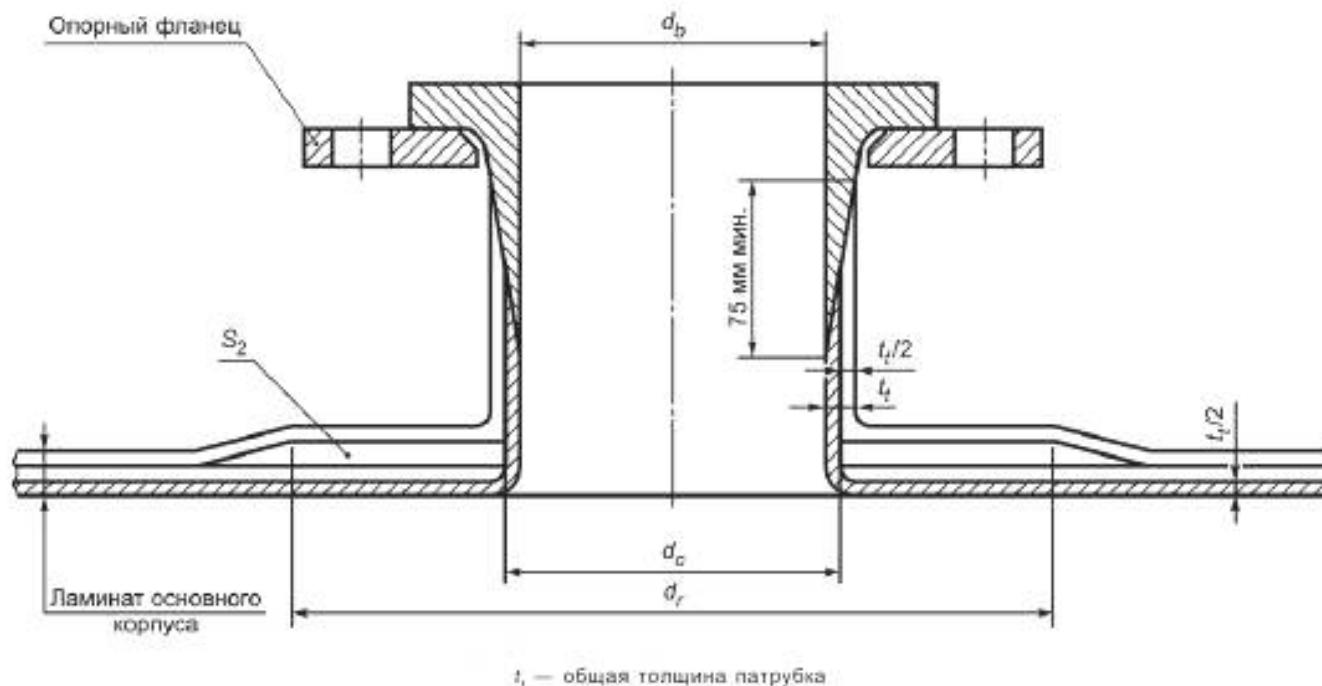
Рисунок К.4 — Схематическое изображение типовых патрубков: установленный заподлицо патрубок без термопластичной футеровки или с термопластичной футеровкой (не изображено)
