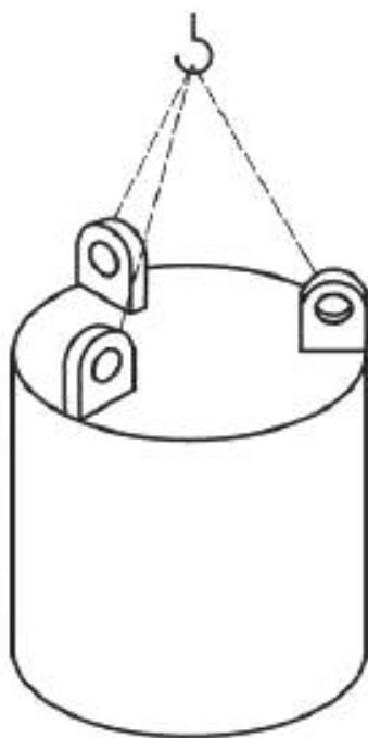
Рисунок X.4 — Равноудаленные радиальные проушины
