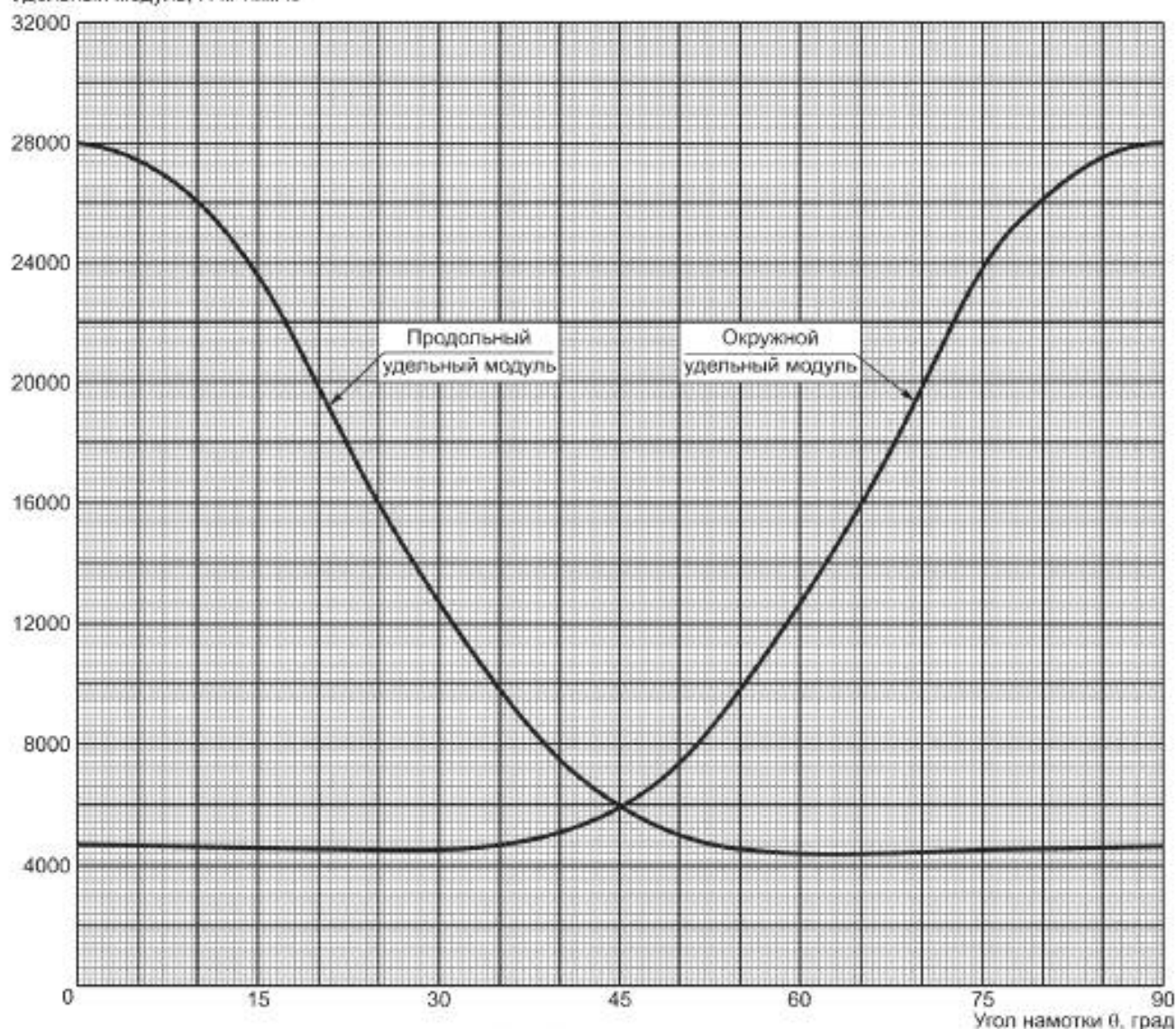
Рисунок А.3 — Зависимость удельного модуля от угла намотки
