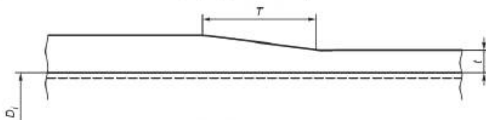
T — длина плавного перехода; l — толщина ламината; D_i — внутренний диаметр корпуса
