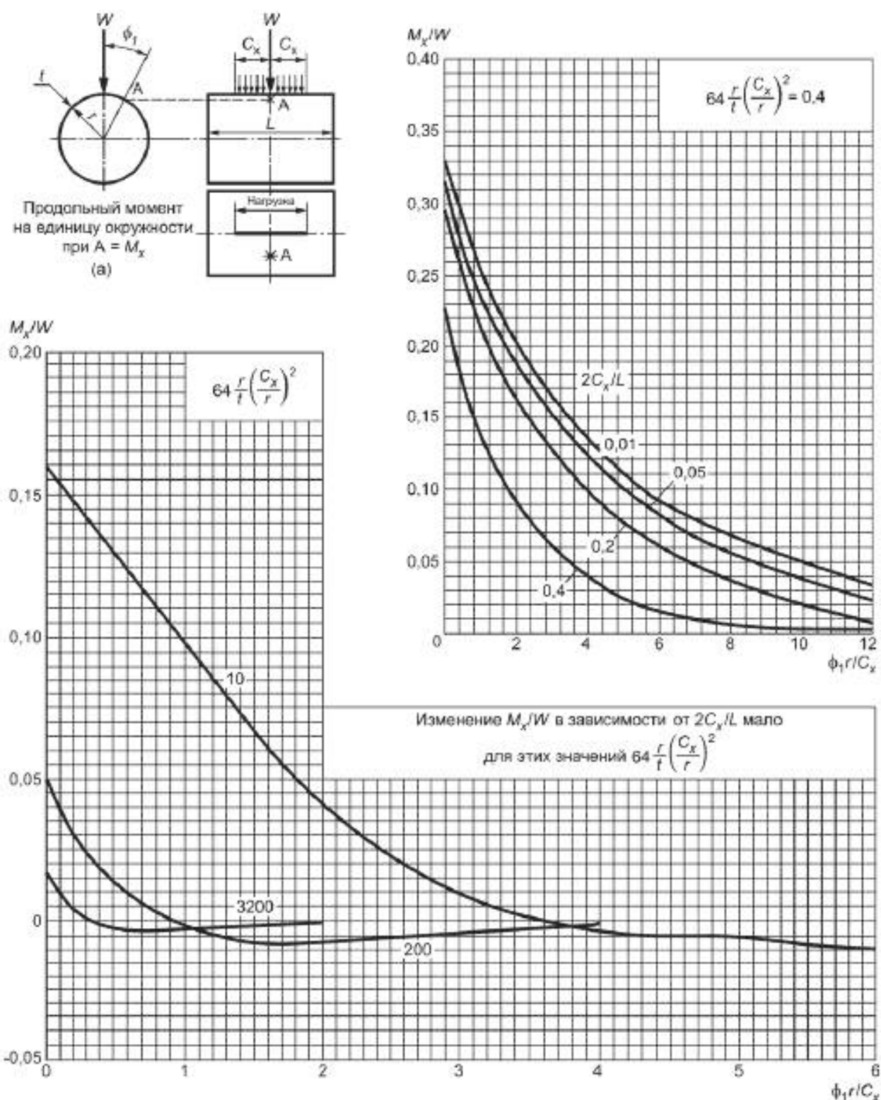
Рисунок Y.11 — Продольный момент, вызванный изменением радиальной линейной нагрузки по окружности (см. Y.2.2.3.2)
