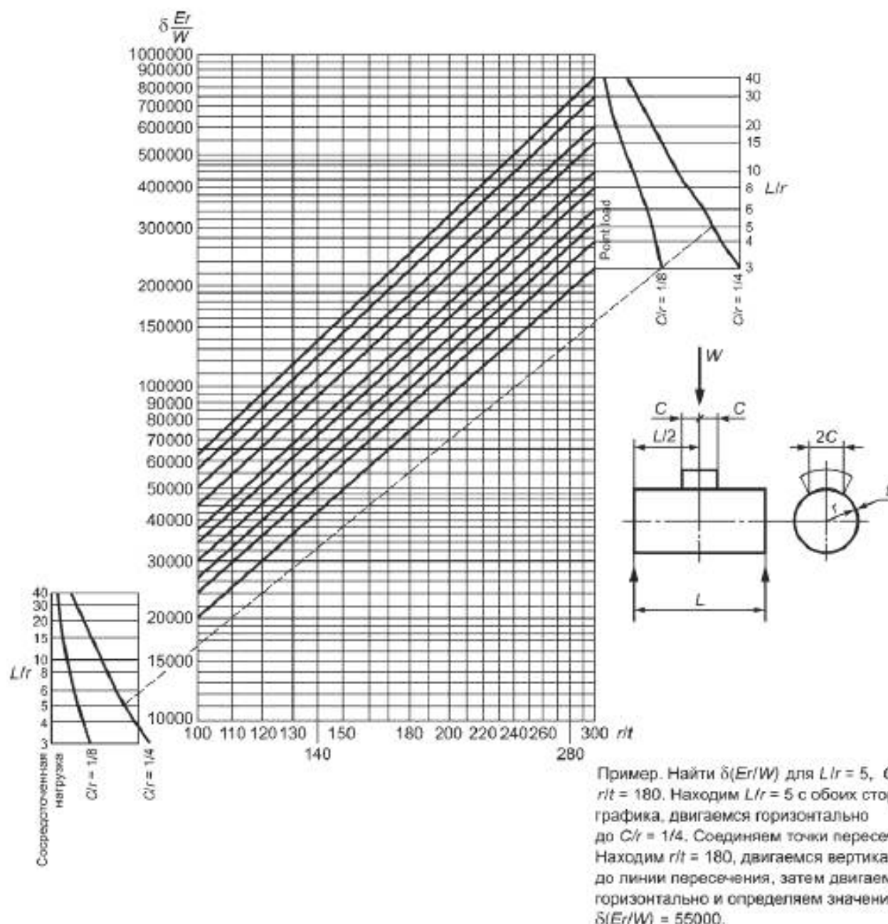
Рисунок У.20 — Максимальная радиальная деформация цилиндрического корпуса, на который воздействует радиальная нагрузка W , равномерно распределенная по квадрату 2C \times 2C
