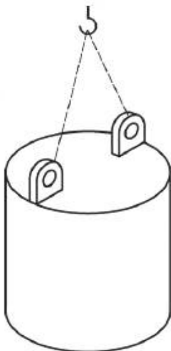
Рисунок X.3 — Проушины в плоскости диаметра
