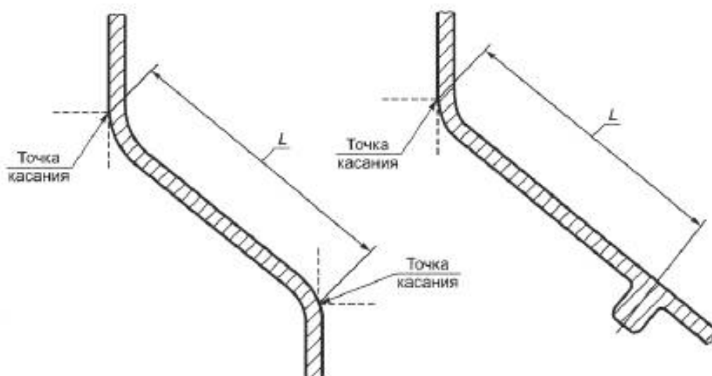
Рисунок В.3 — Конические секции
