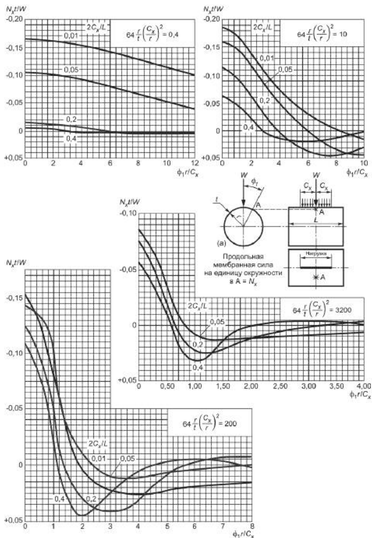
Рисунок Y.13 — Продольные мембранные силы, вызванные изменением радиальной линейной нагрузки по окружности (см. Y.2.2.3.2)
