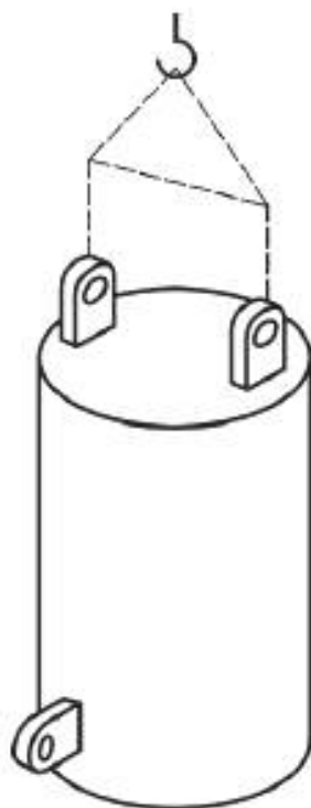
Рисунок X.2 — Параллельные проушины
