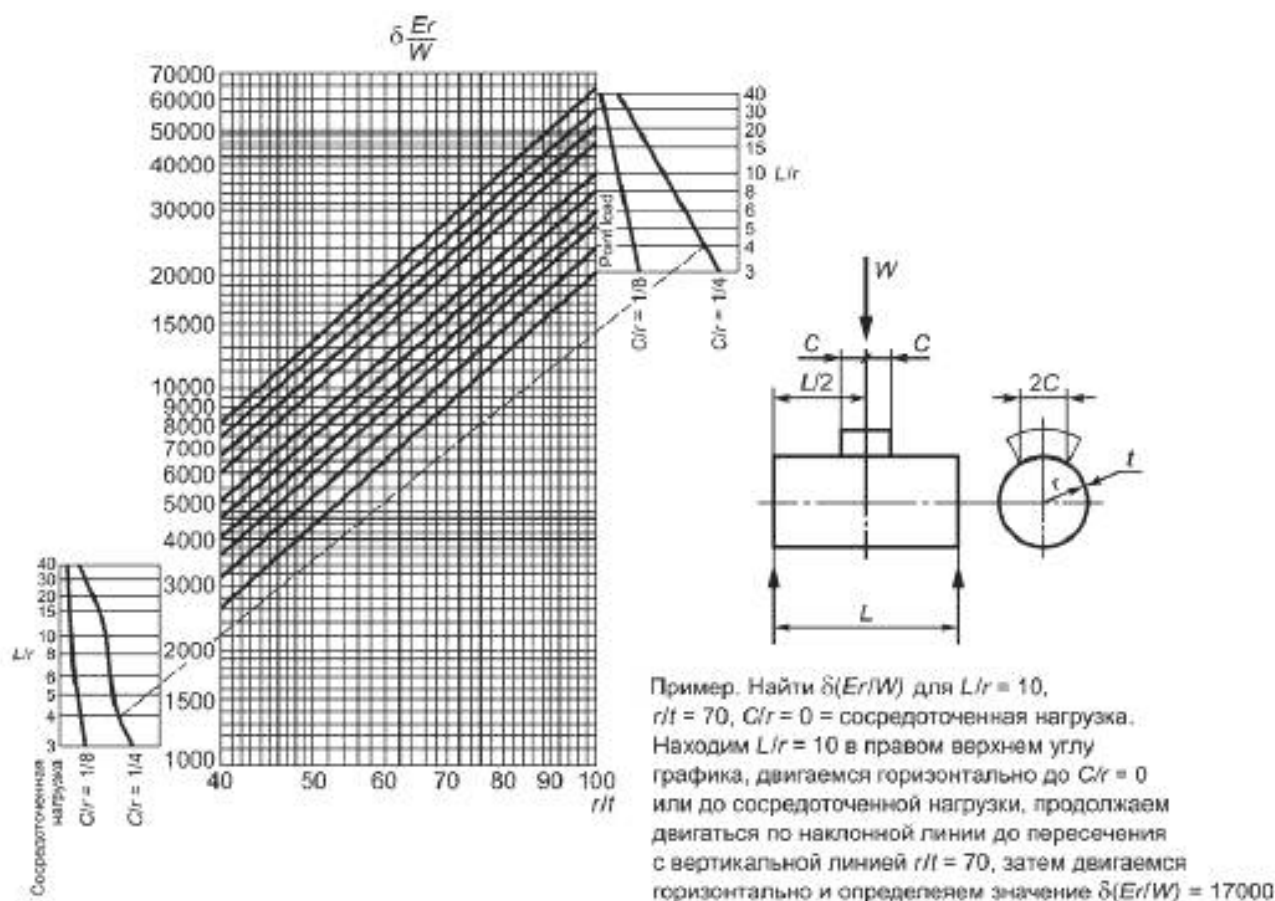
Рисунок У.19 — Максимальная радиальная деформация цилиндрического корпуса, на который действует радиальная нагрузка W , равномерно распределенная по квадрату 2C \cdot 2C
