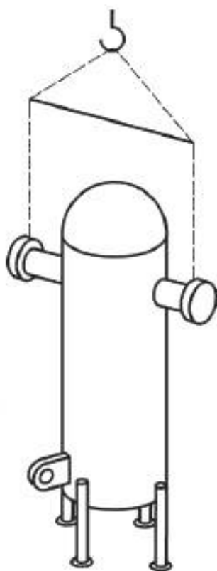
Рисунок X.1 — Цапфы и проушина
