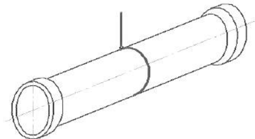
Рисунок 10.3 — Подъем царги в горизонтальном положении одинарной строповкой
