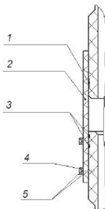
1 — уплотнитель; 2 — компенсатор; 3 — уплотнительная прокладка; 4 — болт; 5 — шайба
