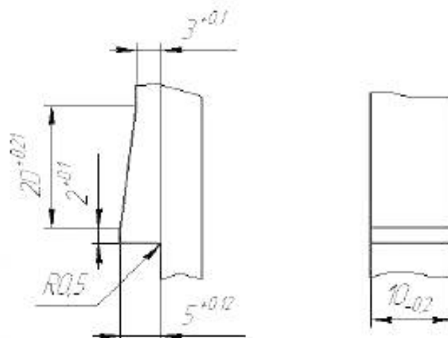
Рисунок Б.3 — Режущая кромка подвижного ножа
