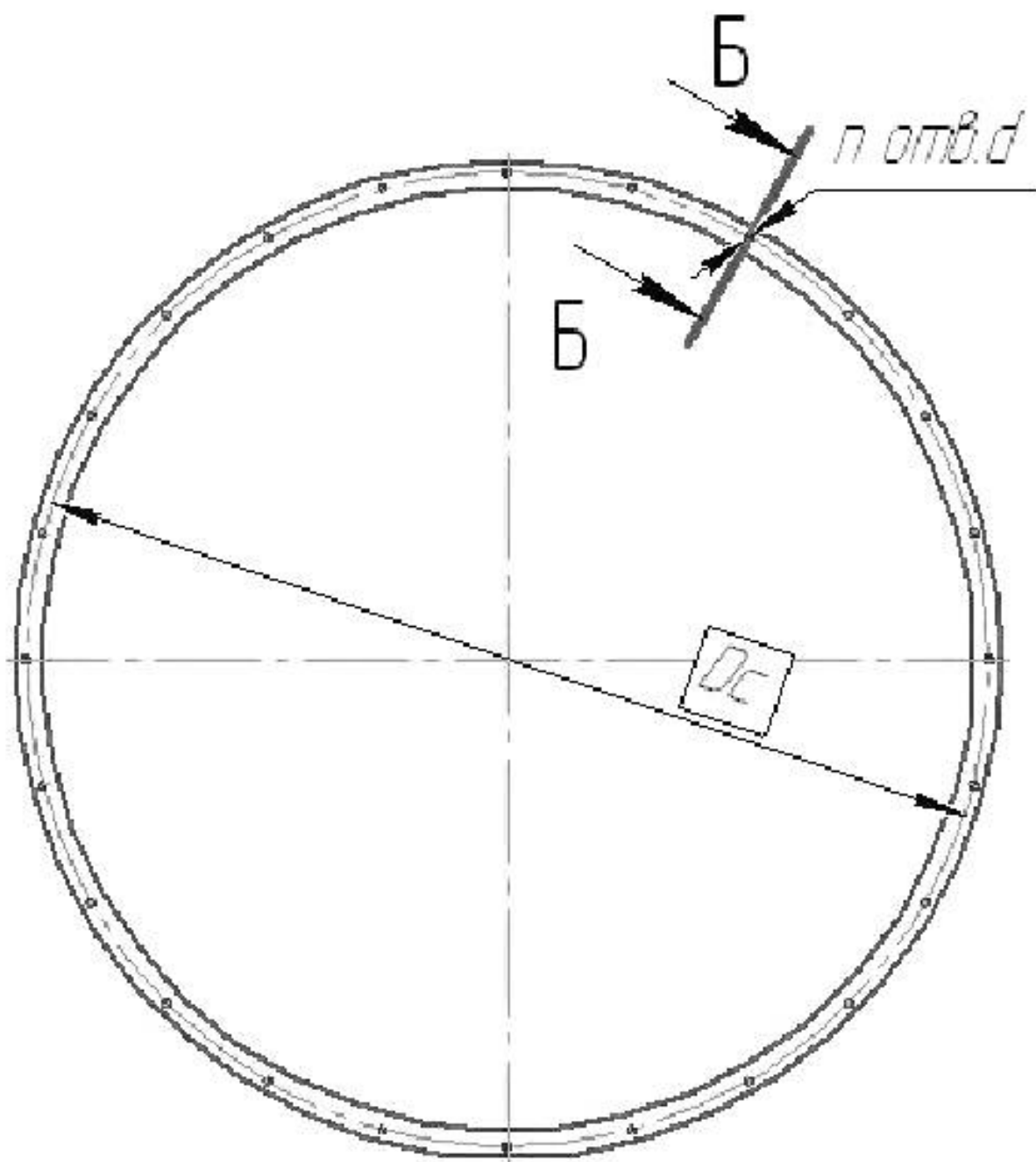
Рисунок А.10 — Расположение монтажных стыковочных отверстий на верхнем торце царг типа Ц, ЦО, ЦР, ЦВК для штифто-шпилечного соединения
