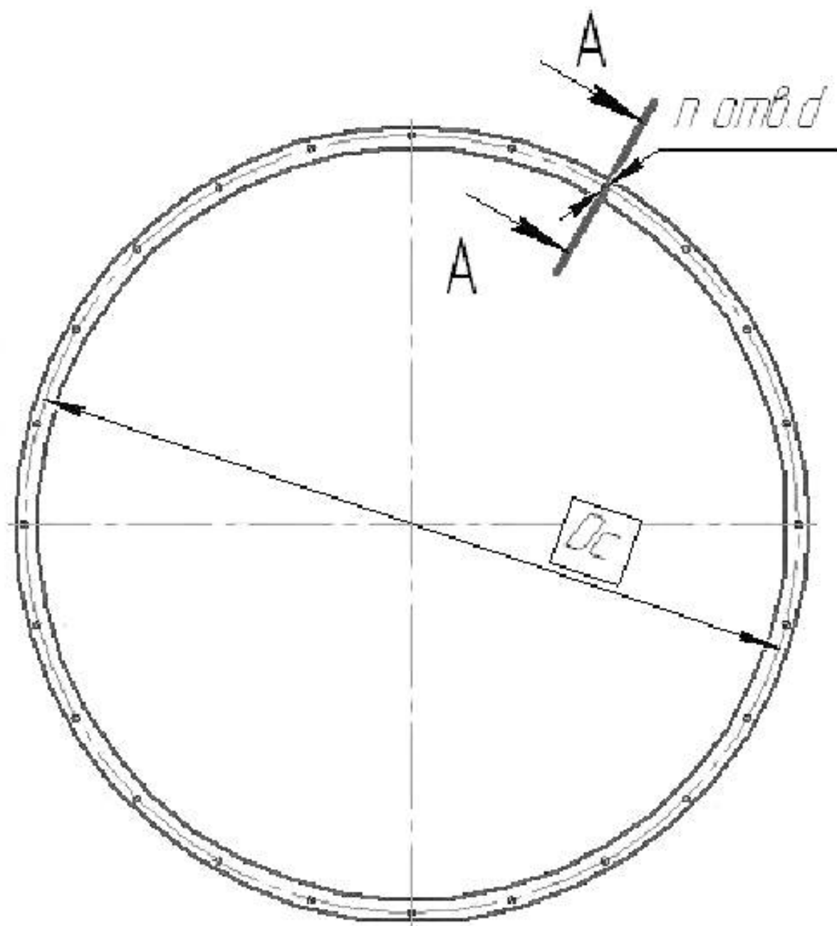
Рисунок А.11 — Расположение монтажных стыковочных отверстий на нижнем торце цагг типа Ц, ЦВ, ЦО, ЦР, ЦНК, ЦНКО для шпилечного и штифто-шпилечного соединений
