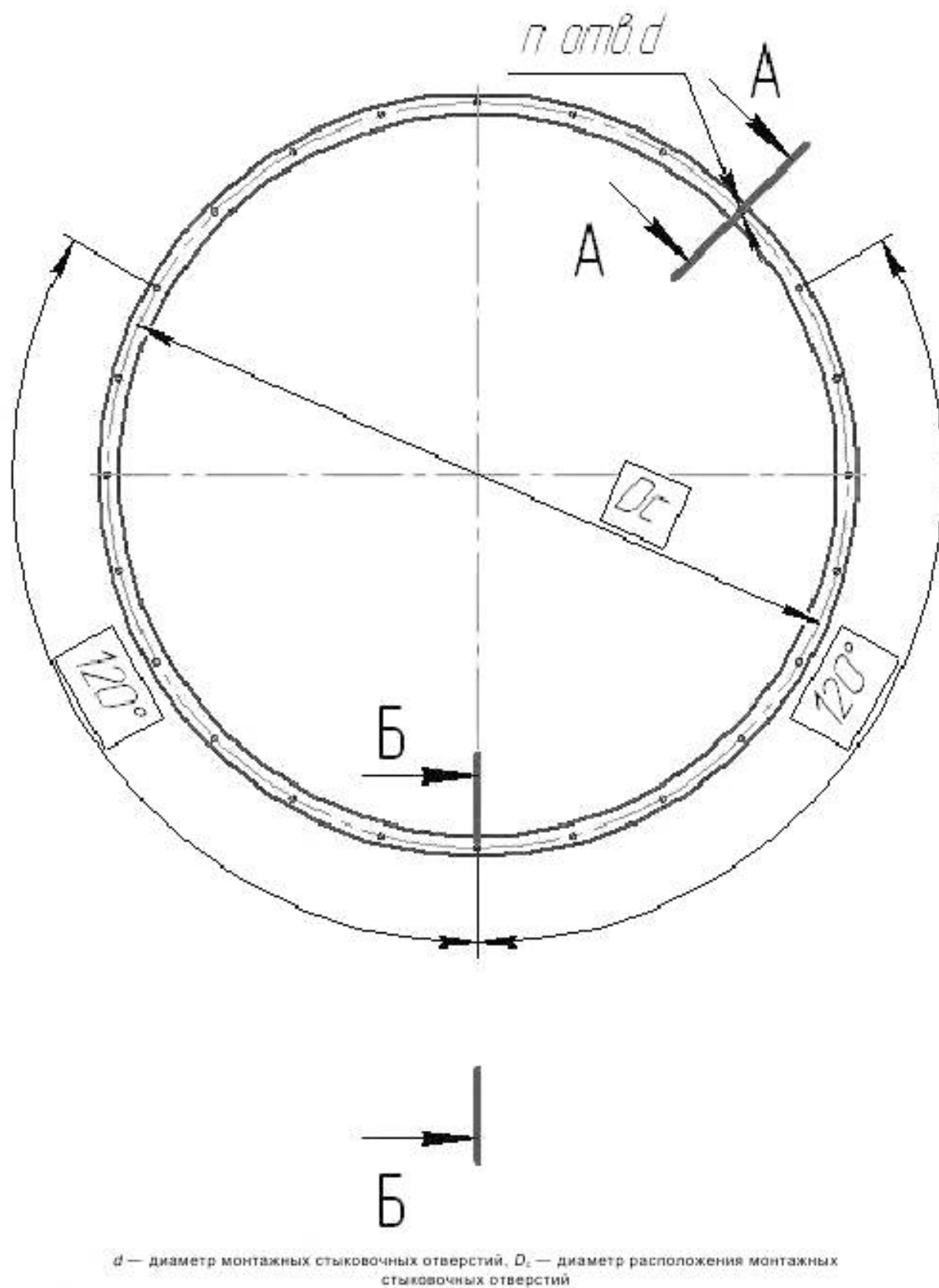
Рисунок А.9 — Расположение монтажных стыковочных отверстий на верхнем торце царг типа Ц, ЦО, ЦР, ЦВК для шпильчатого соединения
