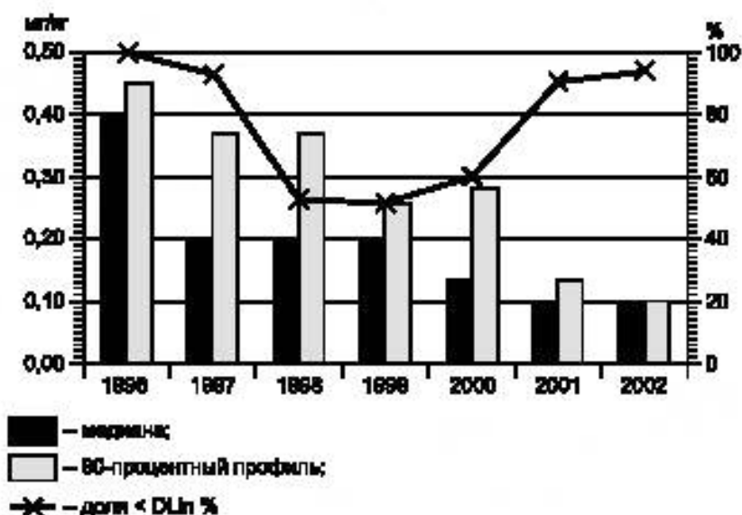
Рисунок Ж.1 — Изменения концентрации ртути в ВРГ
