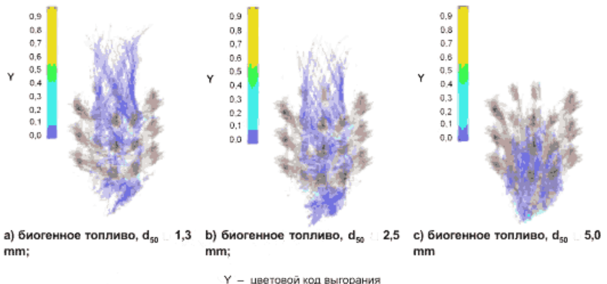
Рисунок 6 — Симуляция выгорания TBT в котле
