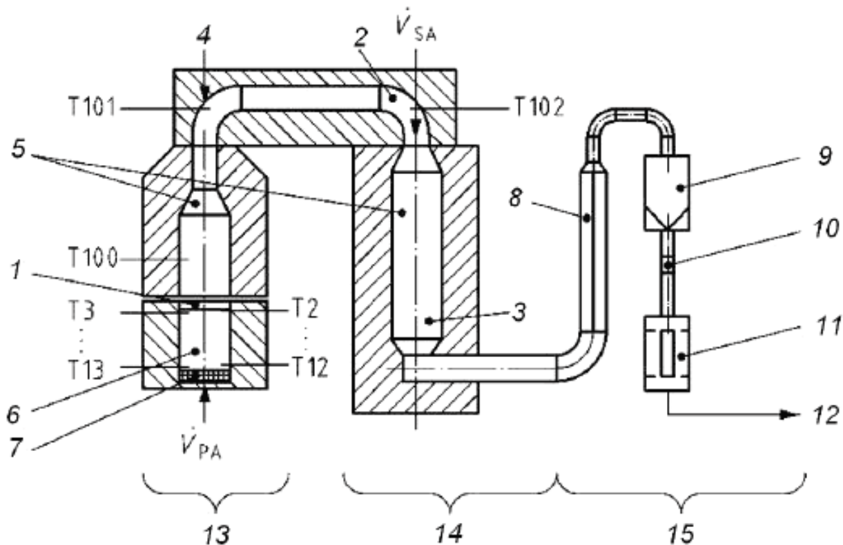
1 – газовая проба 1; 2 – газовая проба 2; 3 – газовая проба 3; 4 – камера; 5 – электрообогрев ( T_{\max} = 1100 \text{ }^{\circ}\text{C} ); 6 – стационарный слой (объем 10 л); 7 – запись массы пробы; 8 – теплообменник; 9 – камера фильтра; 10 – расходомер; 11 – адсорбер Коула; 12 – вентилятор; 13 – камера сжигания; 14 – камера догорания; 15 – очистка дымовых газов
