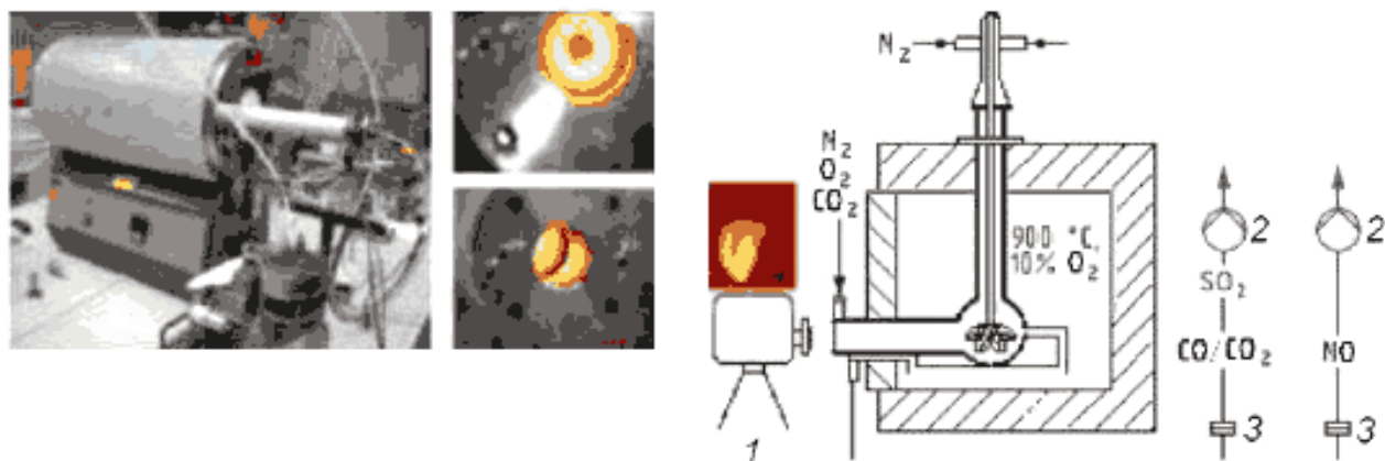
1 – камера высокого разрешения; 2 – насос; 3 – фильтр
