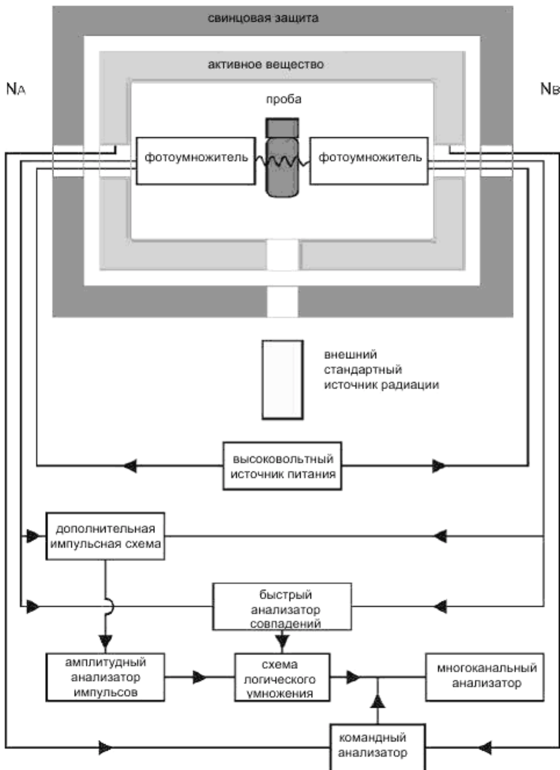
Рисунок А.1 – Жидкостный сцинтилляционный счетчик
