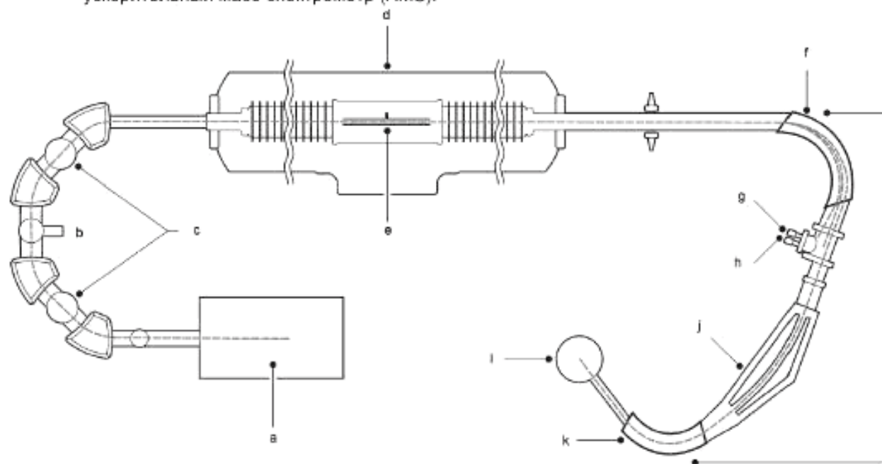
a – источник ионов на 59 проб; b – прерыватель; c – рекомбинатор; d – тандемный ускоритель; e – защищенный канал; f – магнит 110 °C; g – приемник C12; h – приемник C13; i – высокоэнергетический масс-спектрометр; j – электростатический детектор 33 °C; k – магнит 90 °C; l – ионизационная камера
