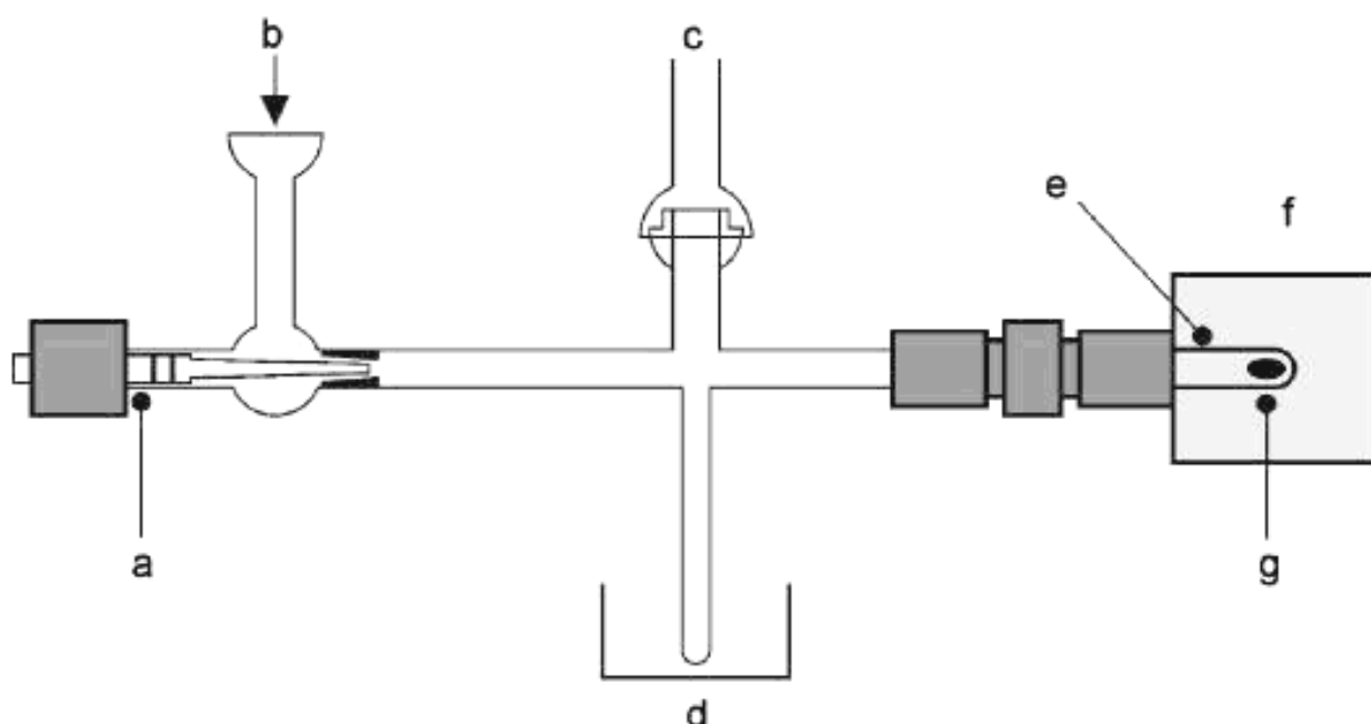
а – ампула с пробой в виде CO 2 ; б – H 2 ; с – датчик давления; d – электронный охлаждающий элемент (-18 ° для улавливания H 2 O); е – кварцевая трубка; f – графитовая печь (600 °C); g – порошок Fe
