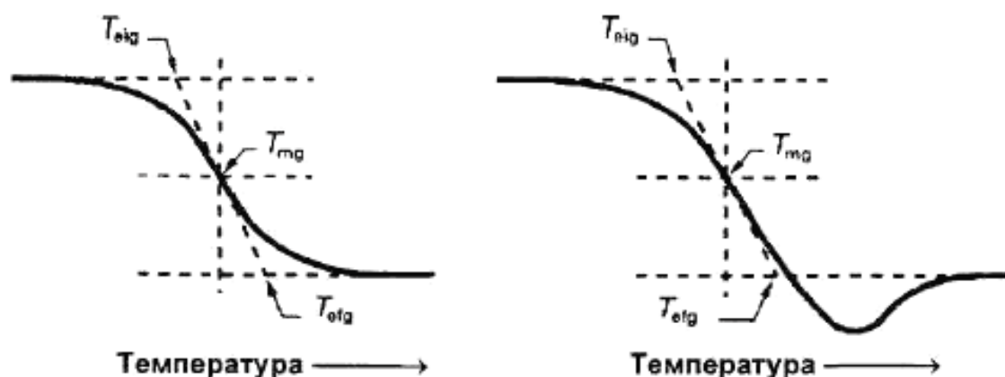
Рисунок 1 – Пример определения температуры стеклования по кривой ДСК
