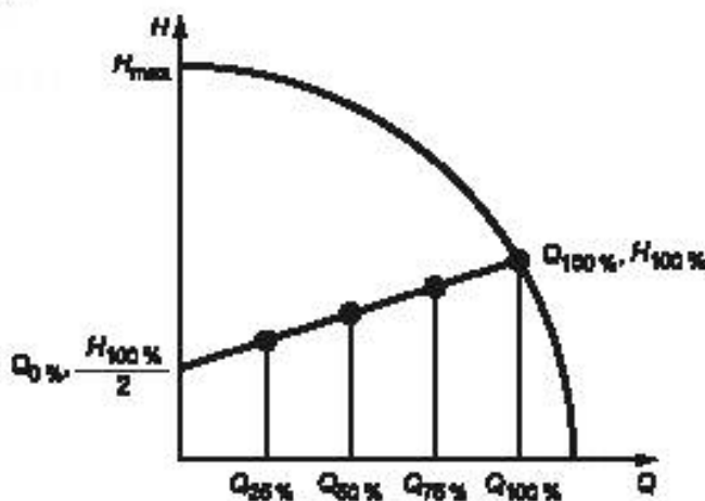
Рисунок 1 — Опорный график производительности циркуляционного насоса
