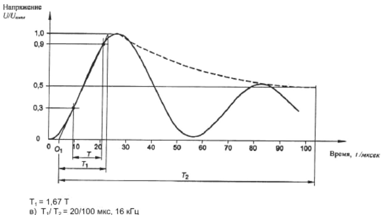
Рисунок 2 – Колебательный грозовой импульс
