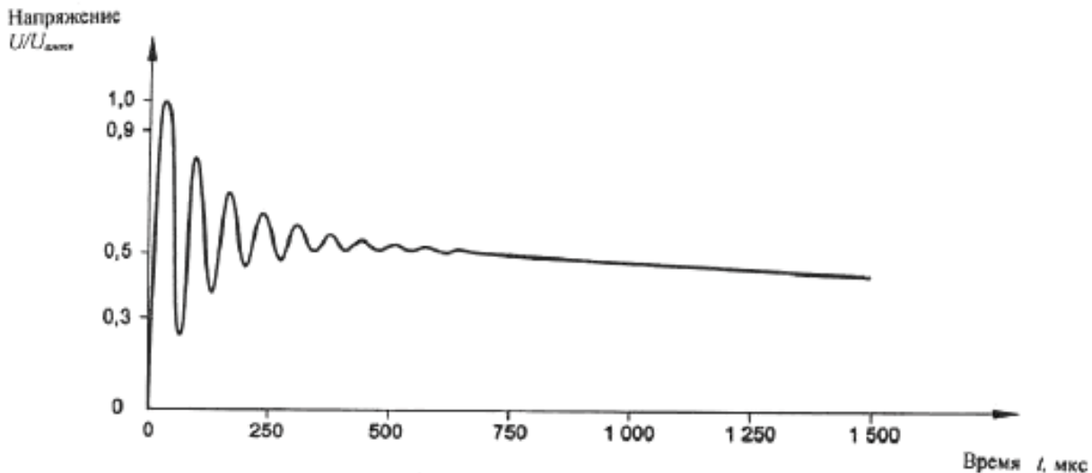
а) T_p / T_2 = 20 / 1\,000 мкс, 15 кГц
