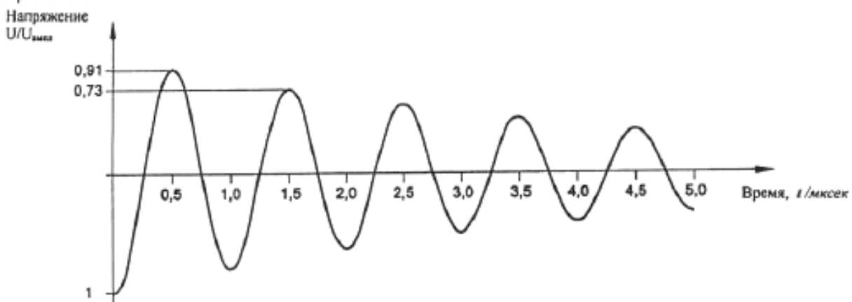
Рисунок 5 - Затухающее переменное напряжение ( f_r = 1 кГц, D_r = 0,2 )
