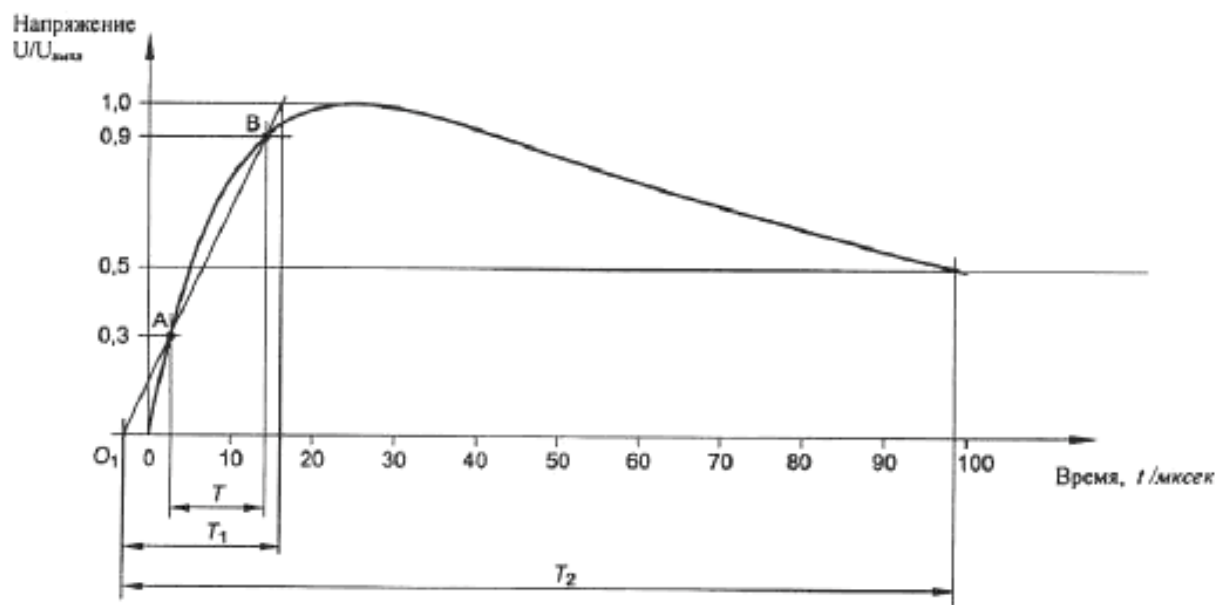
Рисунок 1 – Аперриодический грозовой импульс
