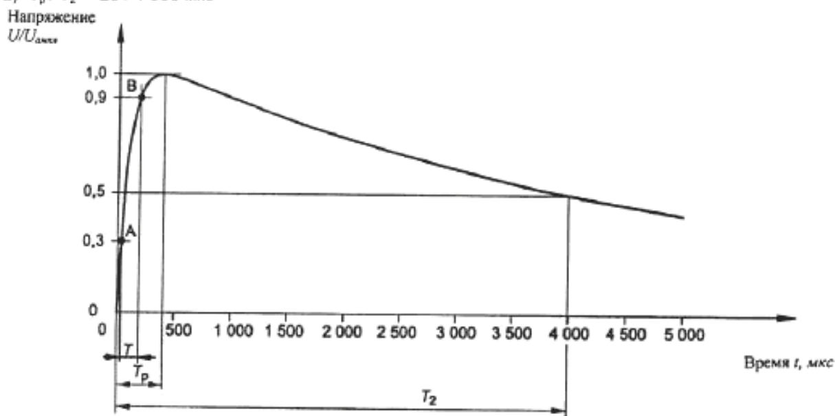
Рисунок 3 - Аперiodический коммутационный импульс
