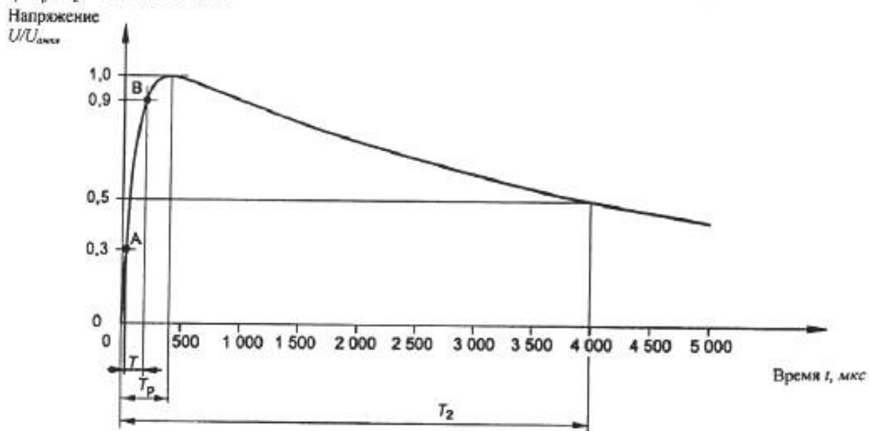
Рисунок 3 - Апериодический коммутационный импульс
