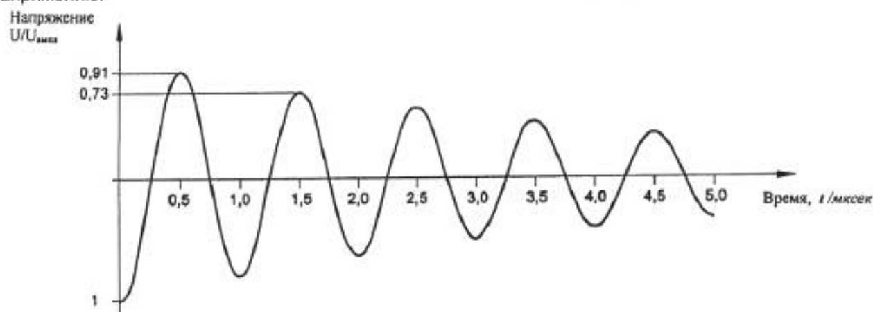
Рисунок 5 - Затухающее переменное напряжение ( f_c = 1 кГц, D_f = 0,2 )
