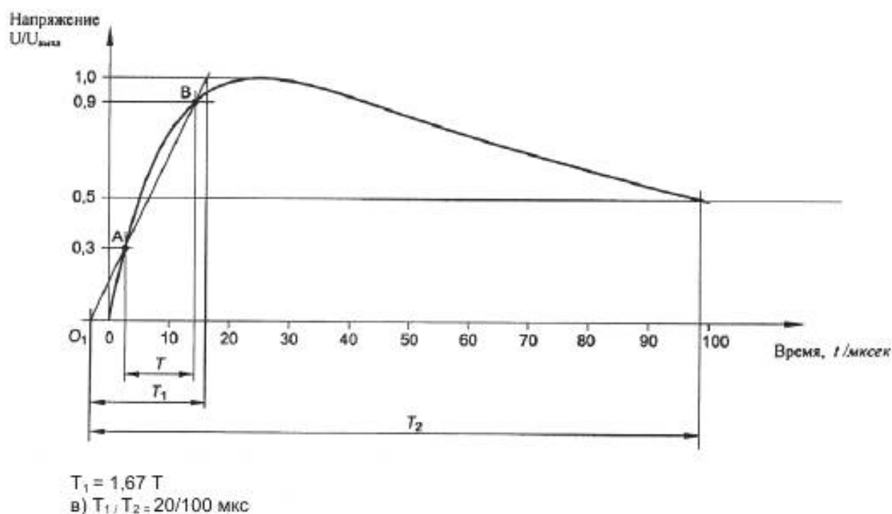
Рисунок 1 – Апериодический грозовой импульс
