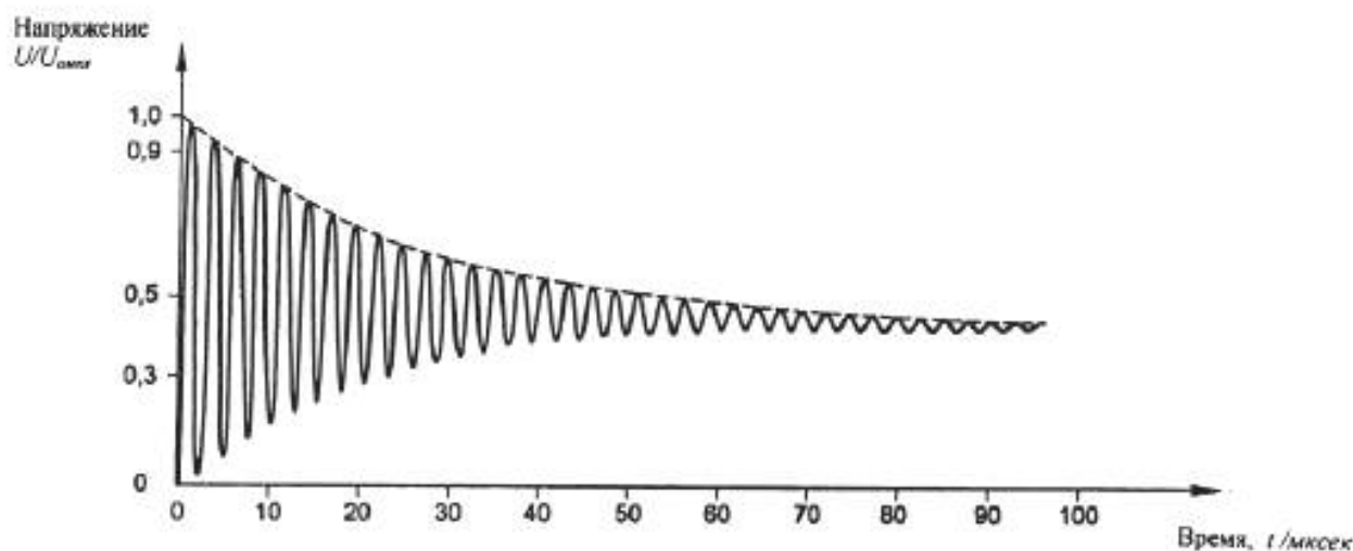
а) T_1/T_2 = 0,8/50 мкс, 370 кГц
