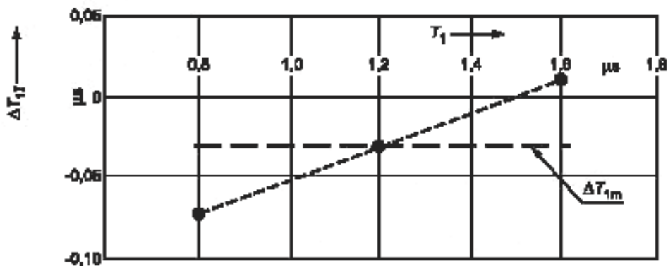
Рисунок Б.2 — Отклонение времени нарастания фронта (длительности переднего фронта) \Delta T_{11} измерительной системы X по отношению к эталонной измерительной системе N и их среднее значение \Delta T_{1m} в диапазоне T_1 = 0,8 \dots 1,6 \text{ мкс}
