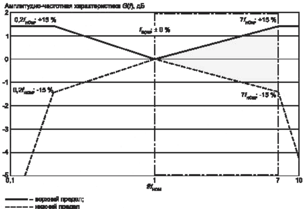
Рисунок 6 — Приемлемая нормализованная амплитудно-частотная характеристика измерительной системы (затемненная область), предназначенная для измерения одной из основных частот f_{\text{ном}} (испытанная в диапазоне 1—7 f_{\text{ном}} )
