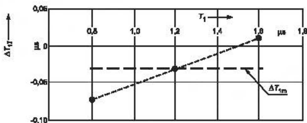
Рисунок Б.2 — Отклонение времени нарастания фронта (длительности переднего фронта) \Delta T_1 , измерительной системы X по отношению к эталонной измерительной системе N и их среднее значение \Delta T_{1m} в диапазоне T_1 = 0,8 \dots 1,6 \text{ мкс}
