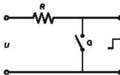
Рисунок В.3,д — Типовая схема цепи ступенчатого генератора
