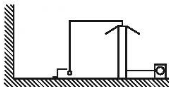
Рисунок В.3,б — Предпочтительная схема цепи для больших делителей
