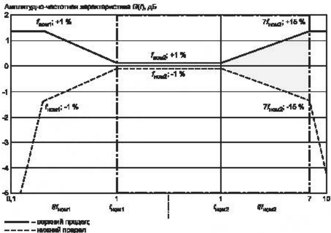
Рисунок 7 — Приемлемая нормализованная амплитудно-частотная характеристика измерительной системы (затененная область), предназначенная для диапазона основных частот от f_{ном1} до f_{ном2} (испытанная в диапазоне f_{ном1}—7f_{ном2} )
