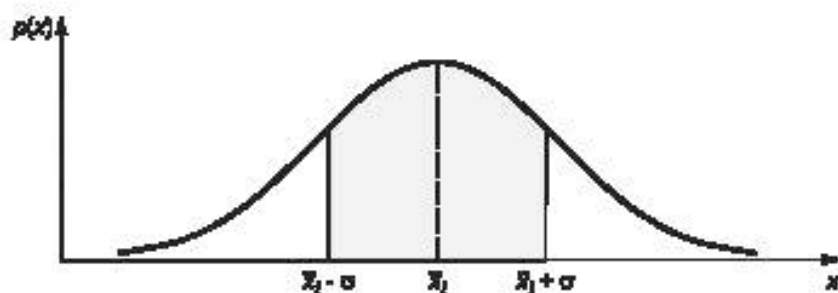
Рисунок А.1 — Плотность нормального распределения вероятности p(x)
