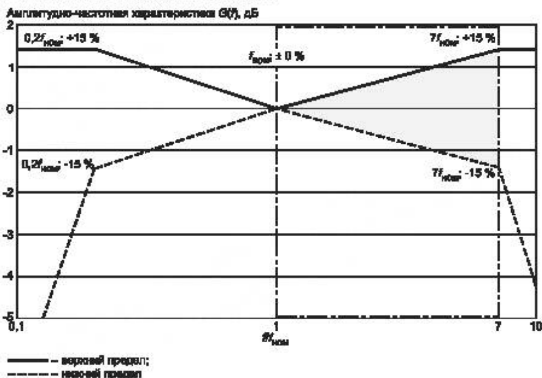
Рисунок 6 — Приемлемая нормализованная амплитудно-частотная характеристика измерительной системы (затененная область), предназначенной для измерения одной из основных частот f_{ном} (испытанная в диапазоне 1—7 f_{ном} )
