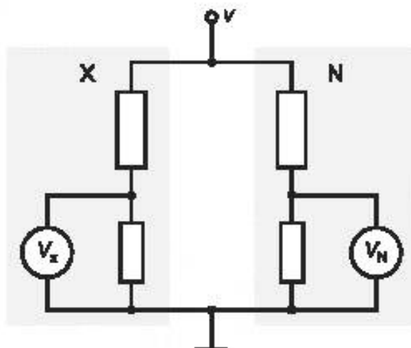
Рисунок Б.1 — Сличение испытуемой системы X с эталонной системой N
