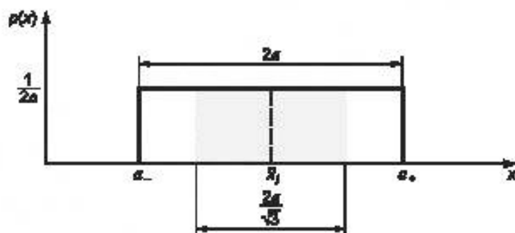
Рисунок А.2 — Плотность равномерного распределения вероятности p(x)
