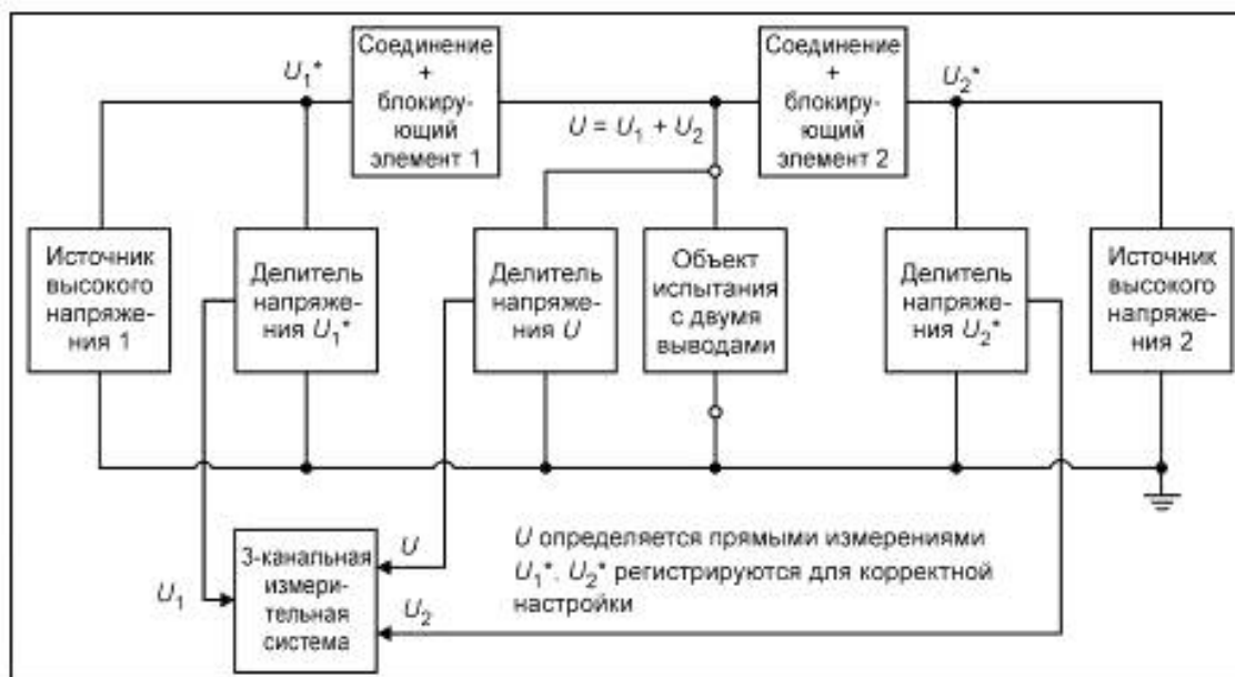
Рисунок 21 — Структурная схема испытаний наложенным напряжением
