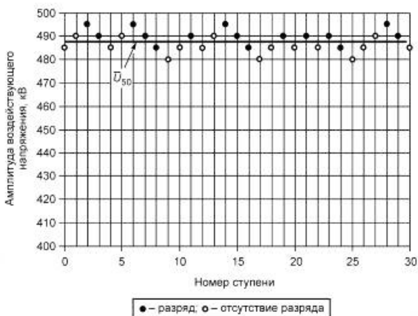
Рисунок А.3 — Результаты испытаний изоляции методом «авверх-вниз» (метод А.2.2)
