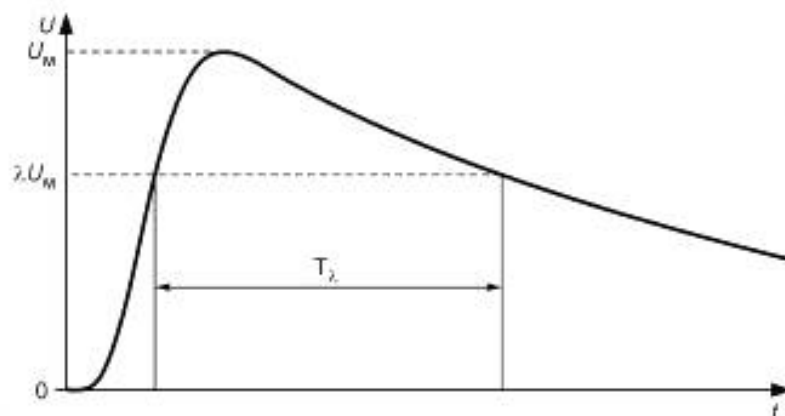
Рисунок 9 — Интервал времени импульсного напряжения
