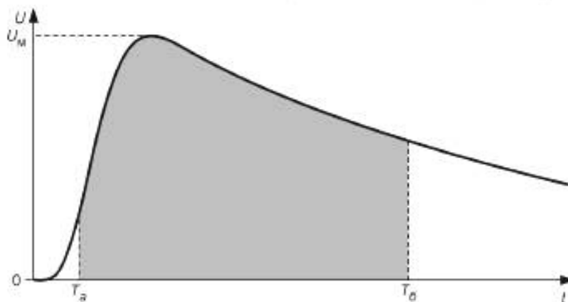
Рисунок 10 — Интеграл импульсного напряжения
