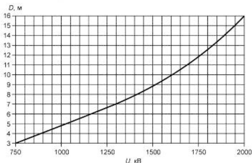
Рисунок 1 — Рекомендуемое наименьшее расстояние D от находящихся под напряжением или заземленных посторонних предметов до высоковольтного электрода испытываемого объекта при испытании кратковременным переменным напряжением или напряжением коммутационного импульса положительной полярности с амплитудным (максимальным) значением U
