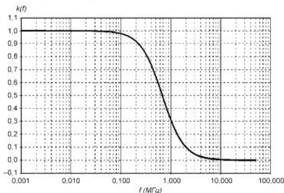
Рисунок 7 — Функция испытательного напряжения
