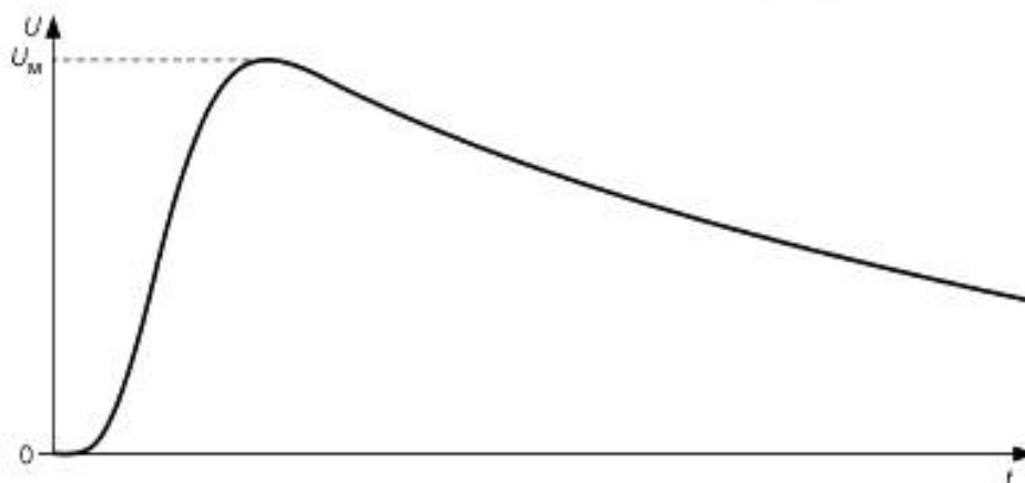
Рисунок 6 — Полный грозовой импульс напряжения
