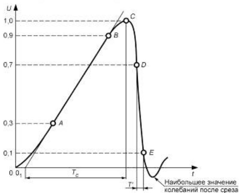
Рисунок 11 — Грозовой импульс, срезанный на фронте
