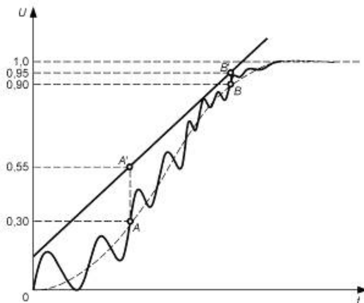
Рисунок 14 — Допустимые колебания на фронте импульса
