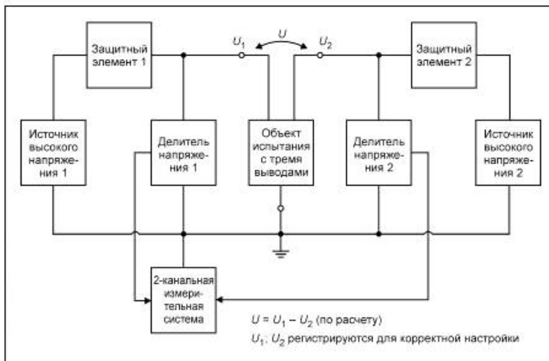
Рисунок 18 — Структурная схема испытаний комбинированным напряжением
