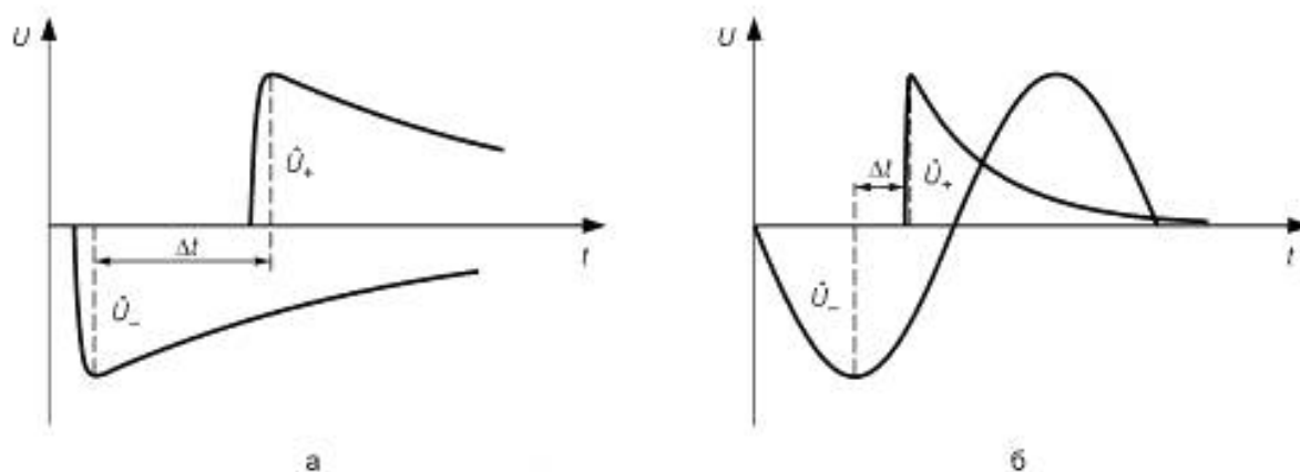
Рисунок 20 — Определение задержки по времени \Delta t
