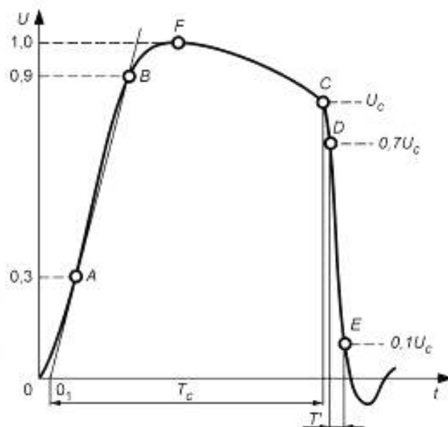
Рисунок 12 — Грозовой импульс, срезанный на спаде импульса
