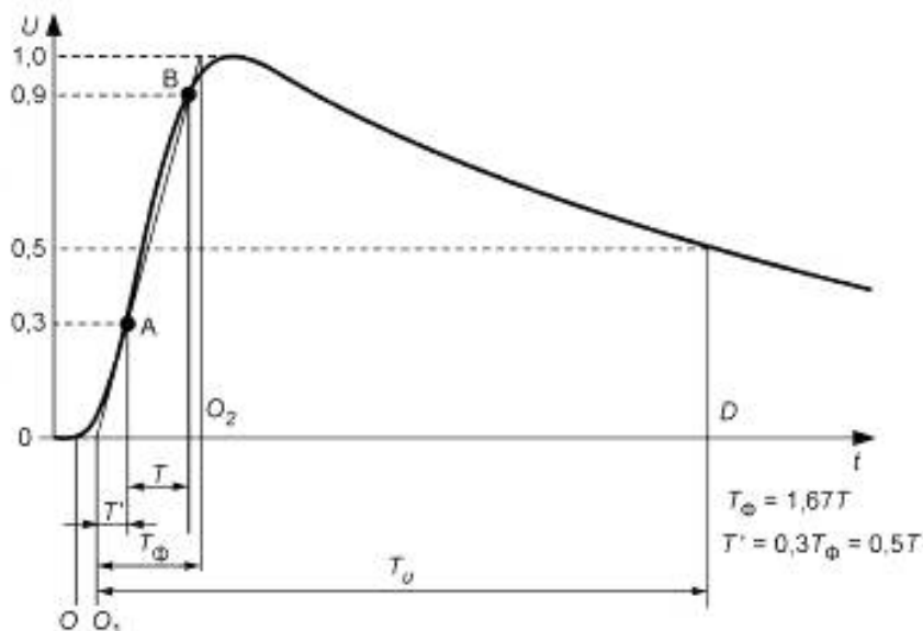
Рисунок 8 — Временные параметры напряжения полного грозового импульса
