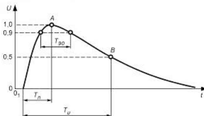
Рисунок 16 — Апериодический коммутационный импульс
