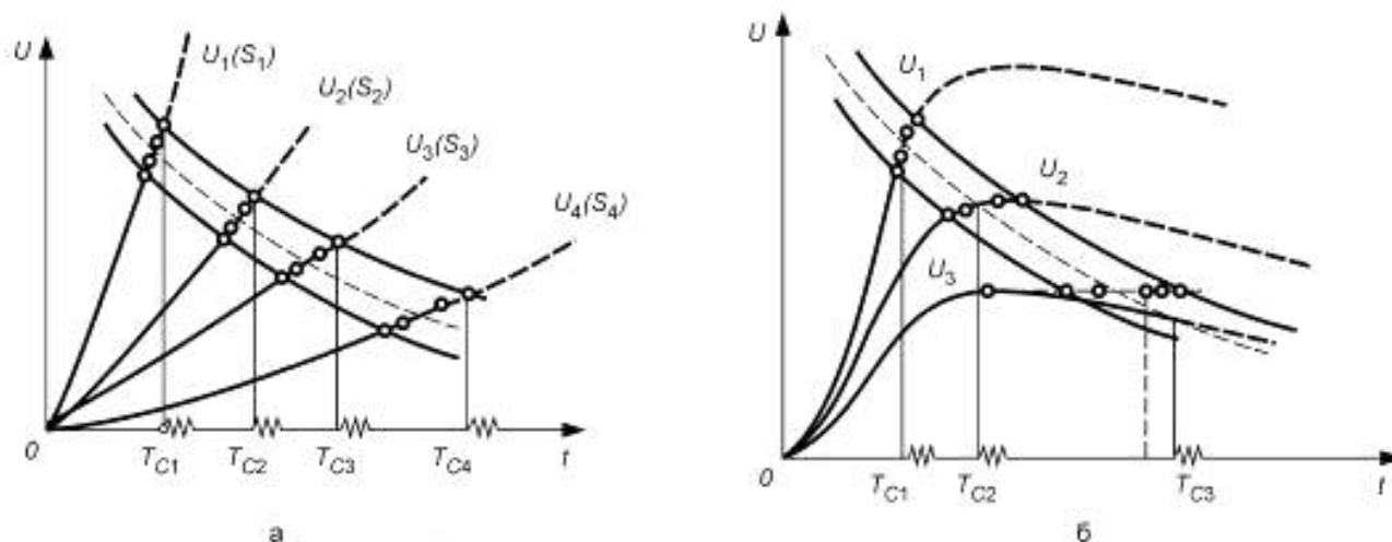
Рисунок 15 — Вольт-секундные характеристики изоляции
