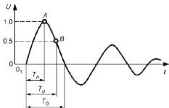
Рисунок 17 — Колебательный коммутационный импульс
