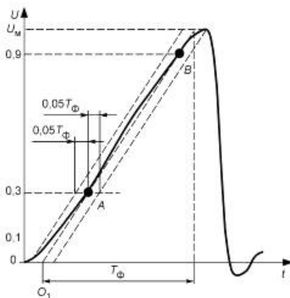
Рисунок 13 — Линейно нарастающий импульс, срезанный на фронте
