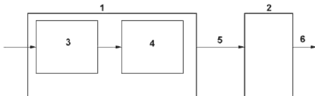
1 – EPSD; 2 – центральная группа; 3 – электронный датчик давления; 4 – преобразователь сигнала; 5 – интерфейс; 6 – разъем
