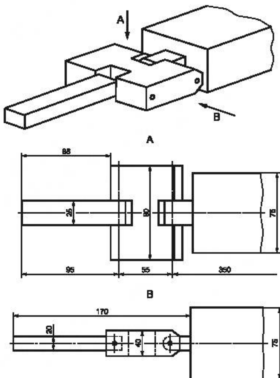
Рисунок 101 — Тестовый палец
