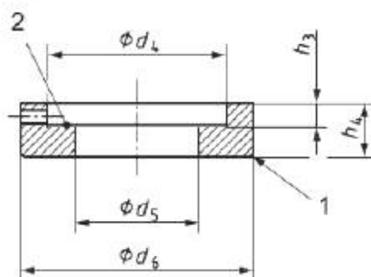
Рисунок А.2 – Промежуточное кольцо, тип А
