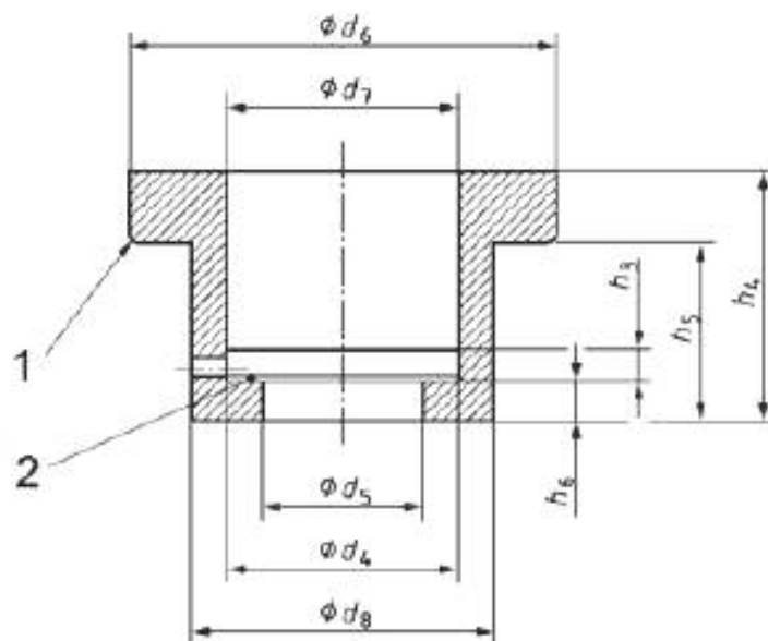
Рисунок А.3 – Промежуточное кольцо, тип В
