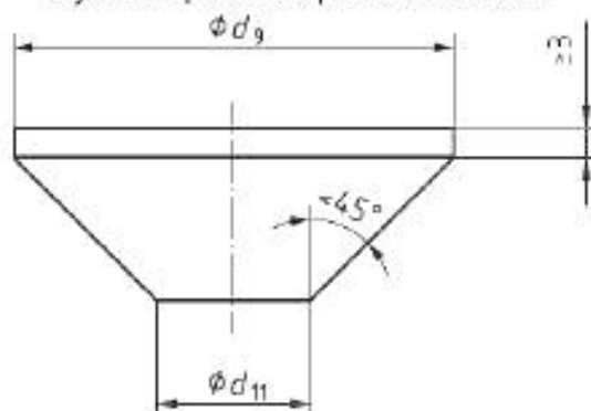
Рисунок А.4 – Нагрузочные опоры
