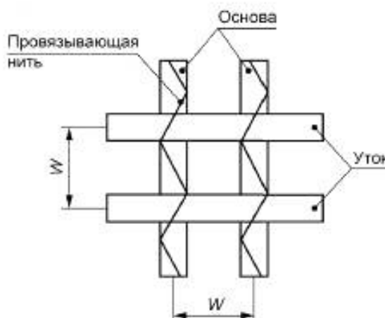
Рисунок 1 — Ячейка стеклосетки с перевивочным плетением
