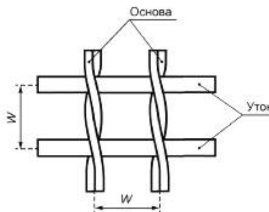
Рисунок 1 — Ячейка стеклосетки с перевивочным плетением
