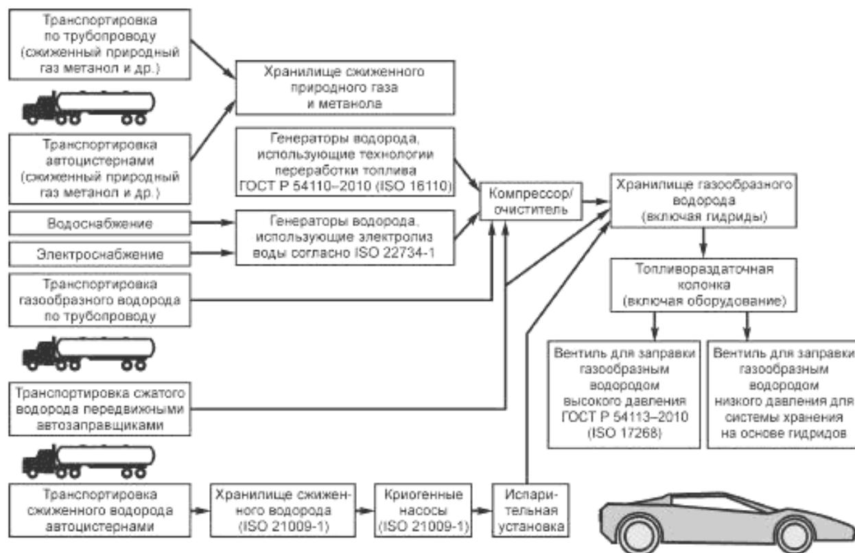
Рисунок 1 — Газообразный водород — заправочная станция
