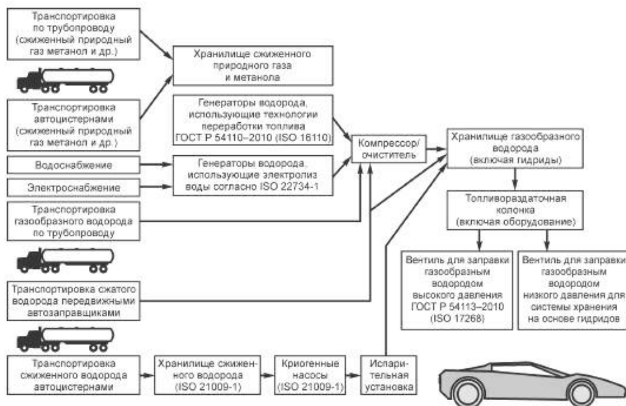
Рисунок 1 — Газообразный водород — заправочная станция
