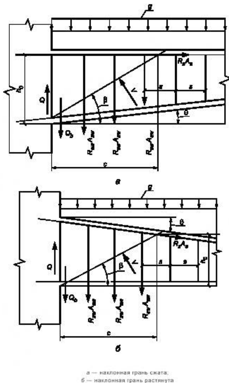
Рисунок 6 — Схема усилий в сечении, наклонном к продольной оси железобетонного элемента, с наклонной гранью при расчете его по прочности на действие поперечной силы
