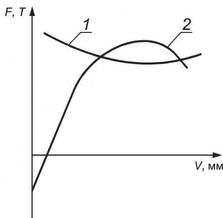
1 — усилие трения; 2 — гидравлическое усилие
