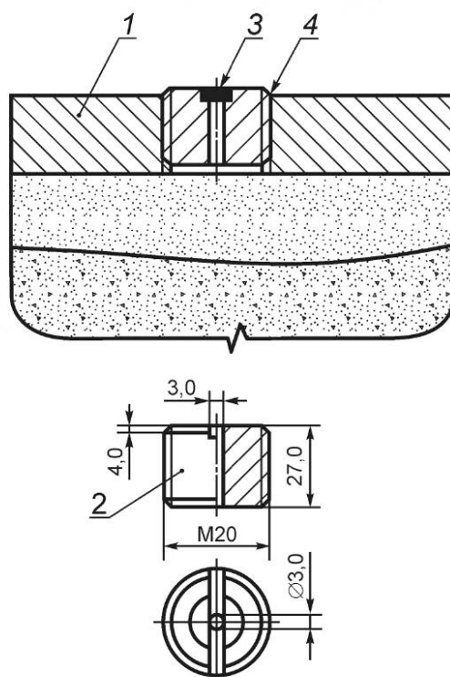
Рисунок В.4.12— Исполнительная схема выявления гидравлической связи
