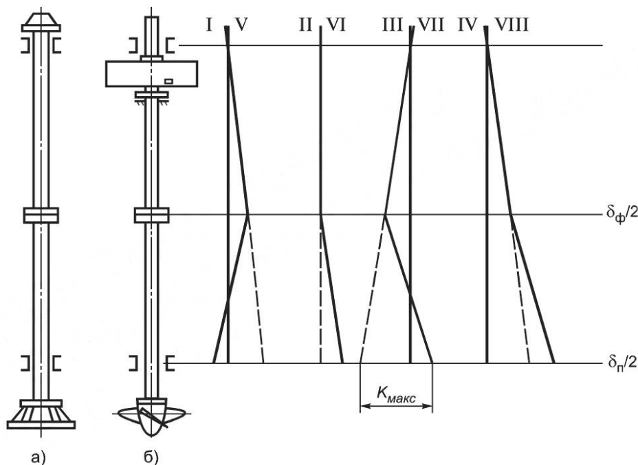
а) гидрогенератор подвесного типа; б) гидрогенератор зонтичного типа
