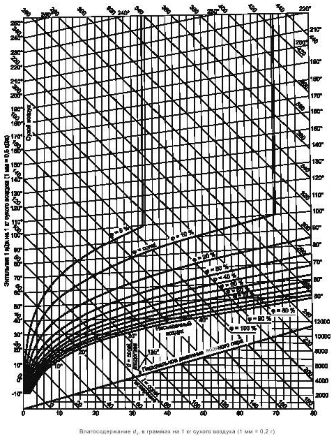
Рисунок И.2 — t - d диаграмма влажного воздуха при 745 мм рт. ст. на 1 кг содержащегося в нем сухого воздуха (для температуры до 250 °C)
