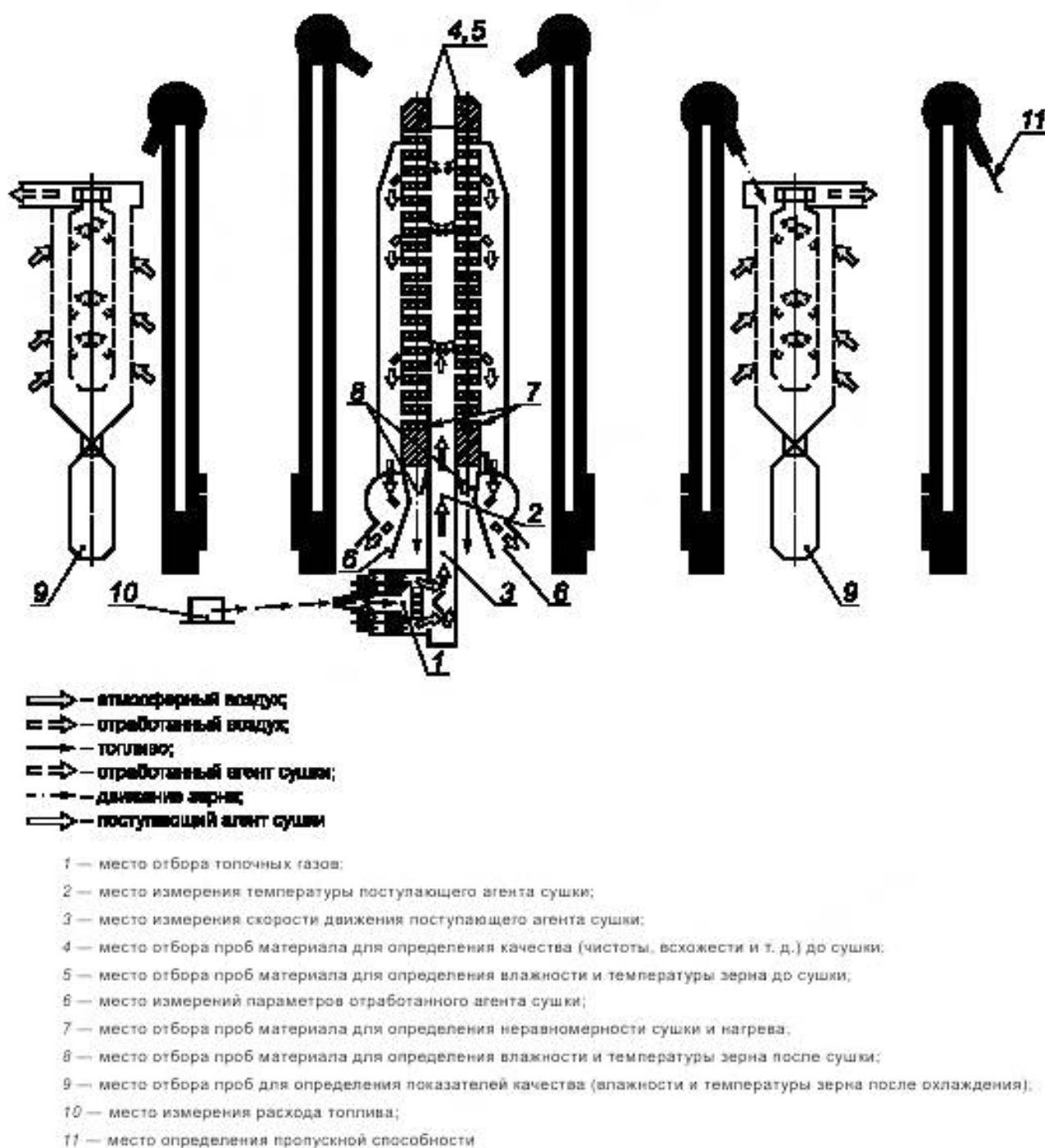
Рисунок В.1 — Схема мест измерений и отбора проб при испытании сушилок шахтного типа
