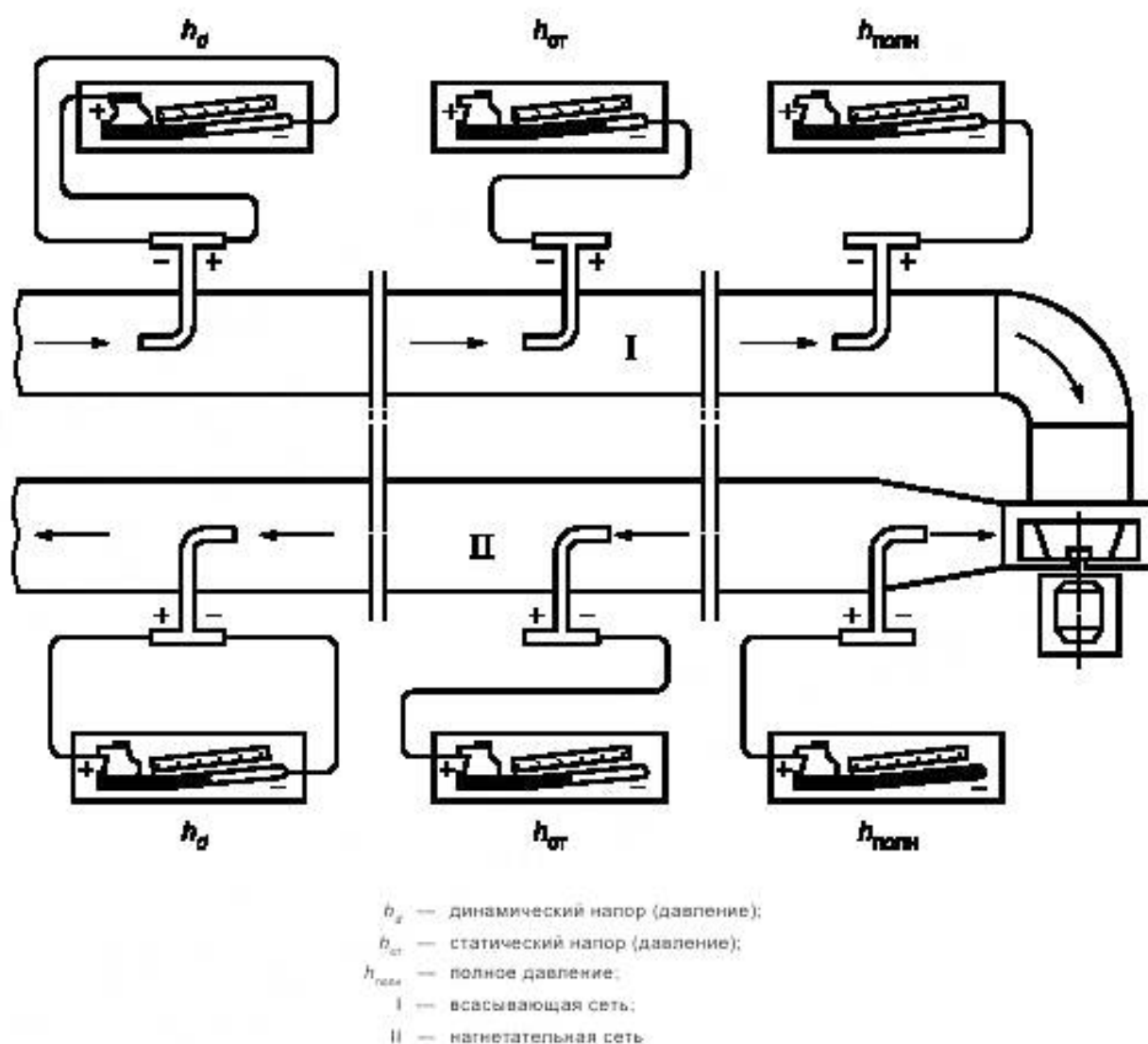
Рисунок 1 — Схема присоединения микроманометра к пневмометрической трубке
