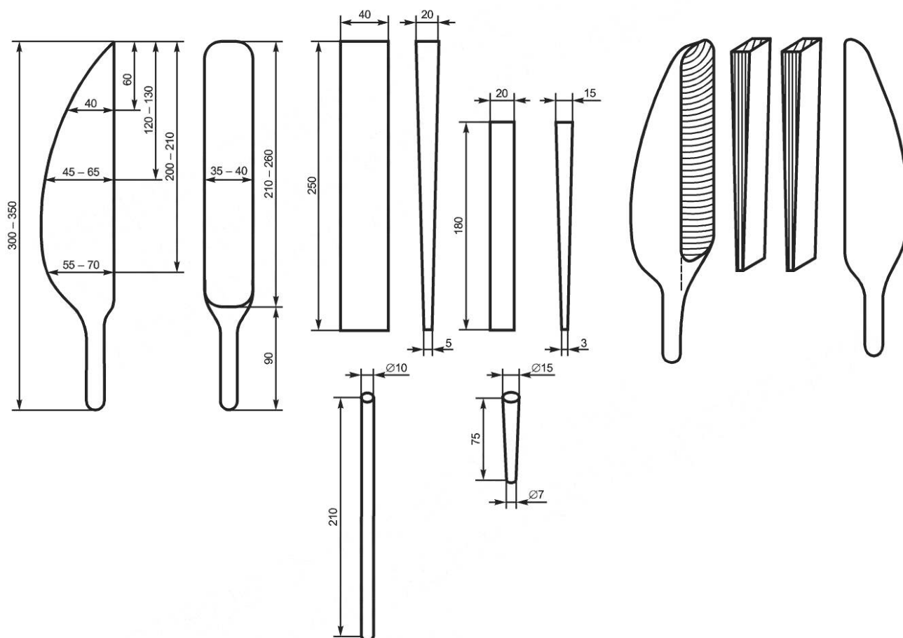
Рисунок Б.1 — Правилка для шкурок соболя
