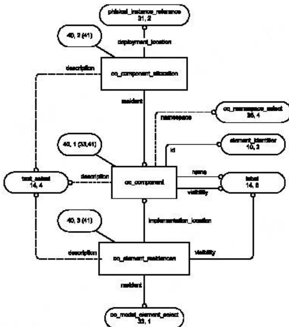
Рисунок Е.41 — Диаграмма ссылочной модели приложения на уровне сущности в нотации EXPRESS-G (40 из 41)
