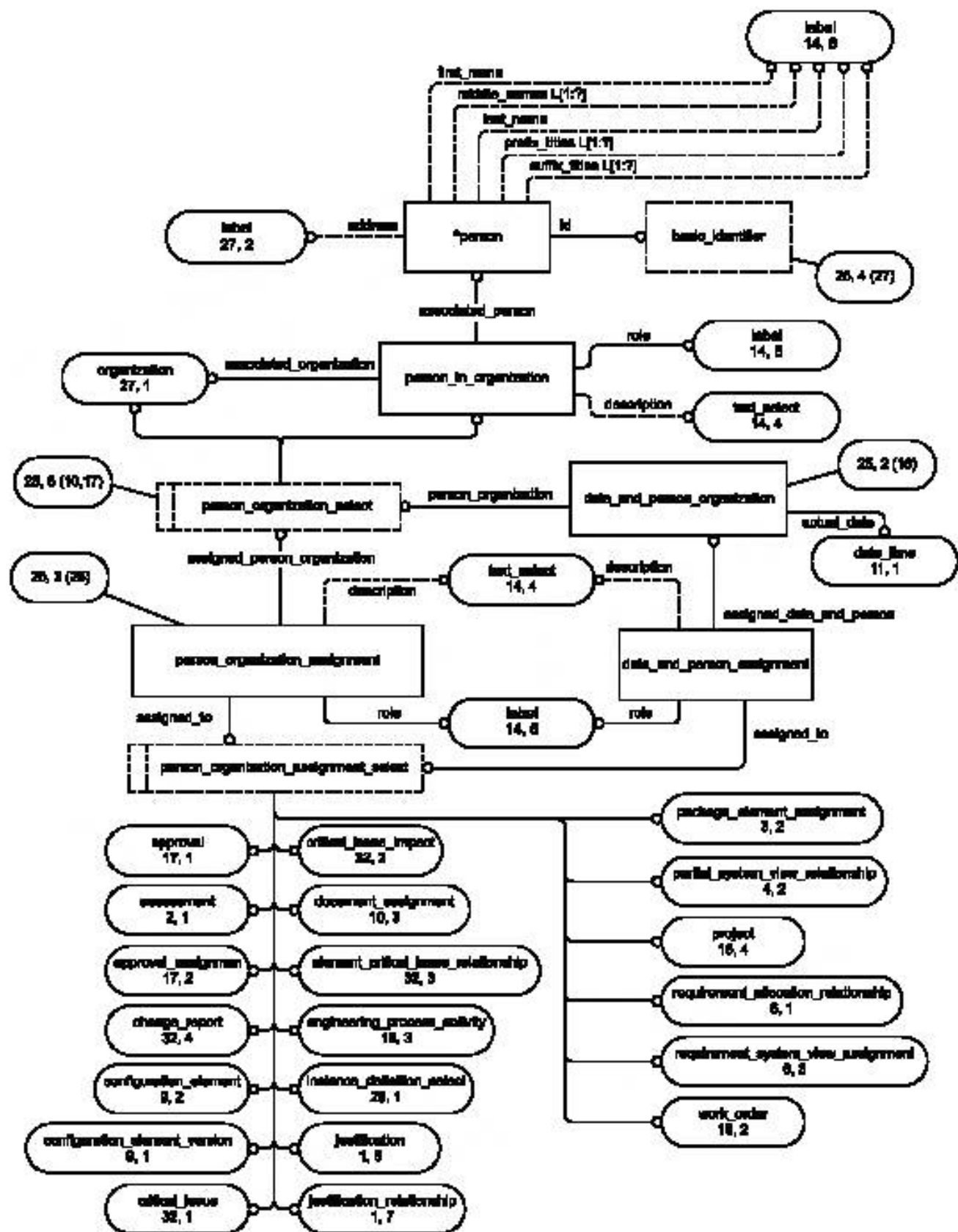
Рисунок E.26 — Диаграмма ссылочной модели приложения на уровне сущности в нотации EXPRESS-G (25 из 41)
