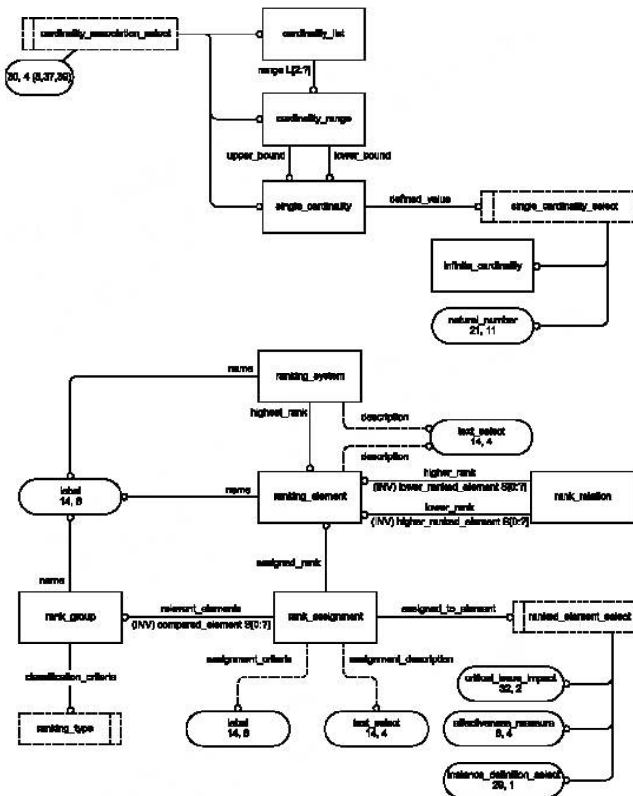
Рисунок E.31 — Диаграмма ссылочной модели приложения на уровне сущности в нотации EXPRESS-G (30 из 41)
