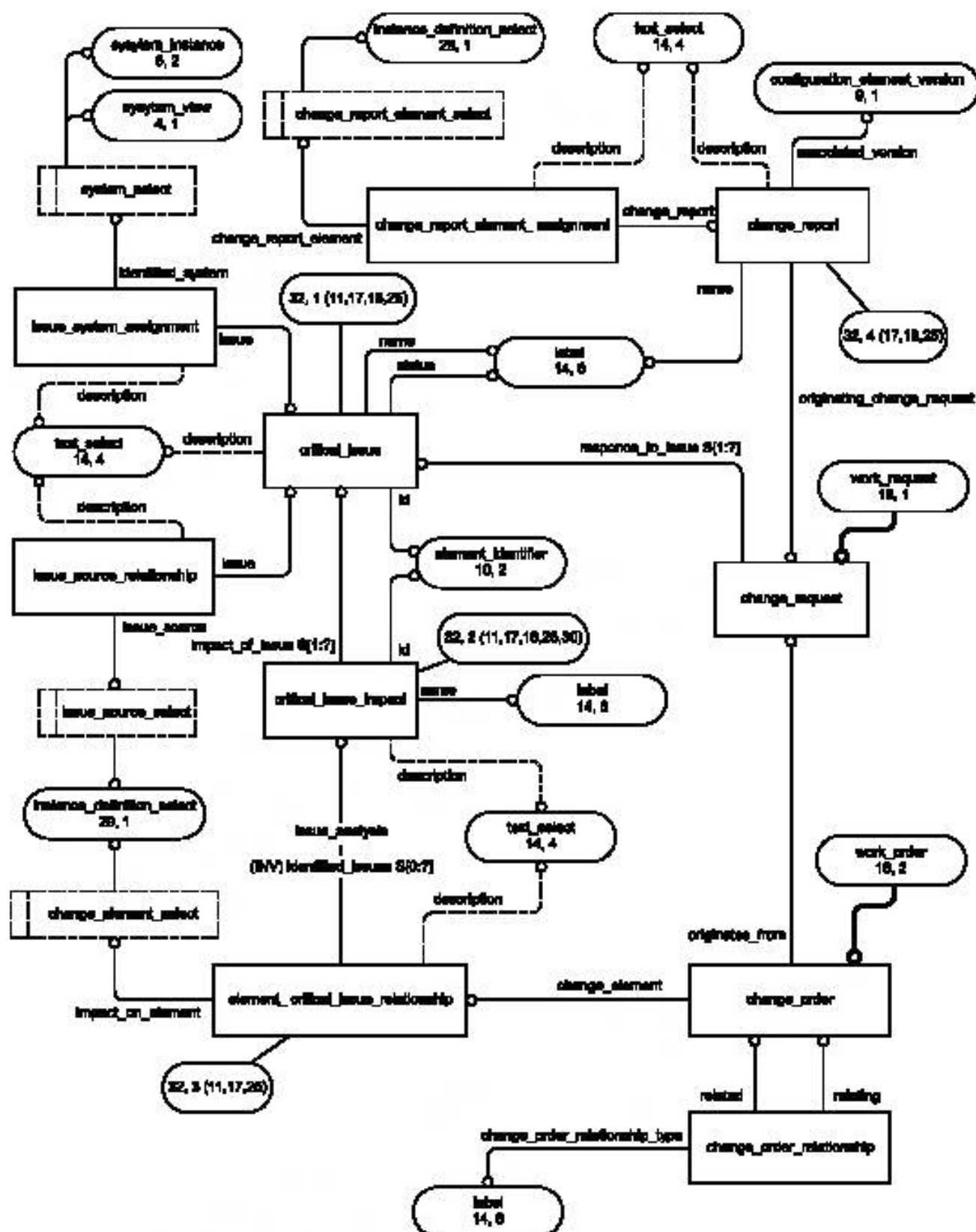
Рисунок E.33 — Диаграмма ссылочной модели приложения на уровне сущности в нотации EXPRESS-G (32 из 41)
