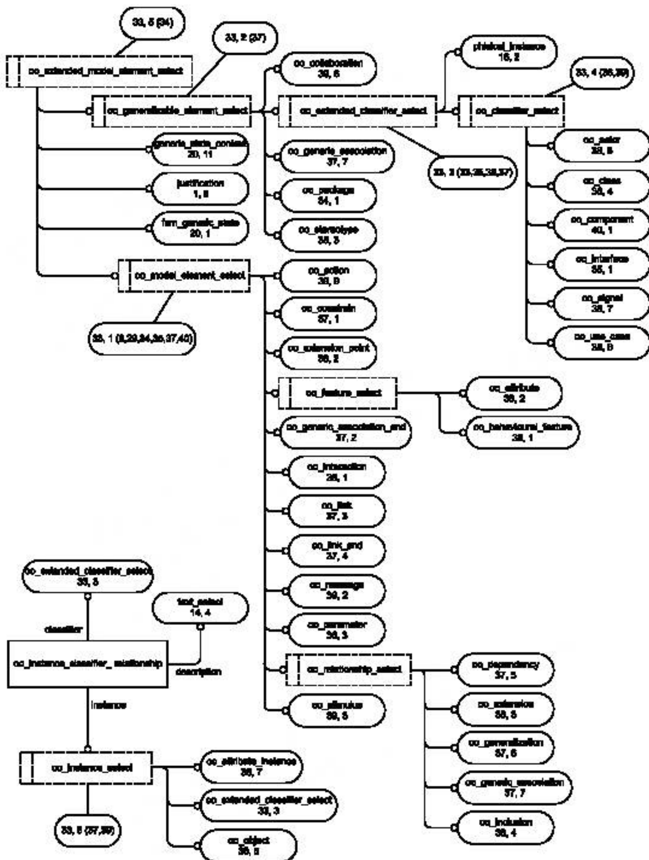
Рисунок Е.34 — Диаграмма ссылочной модели приложения на уровне сущности в нотации EXPRESS-G (33 из 41)
