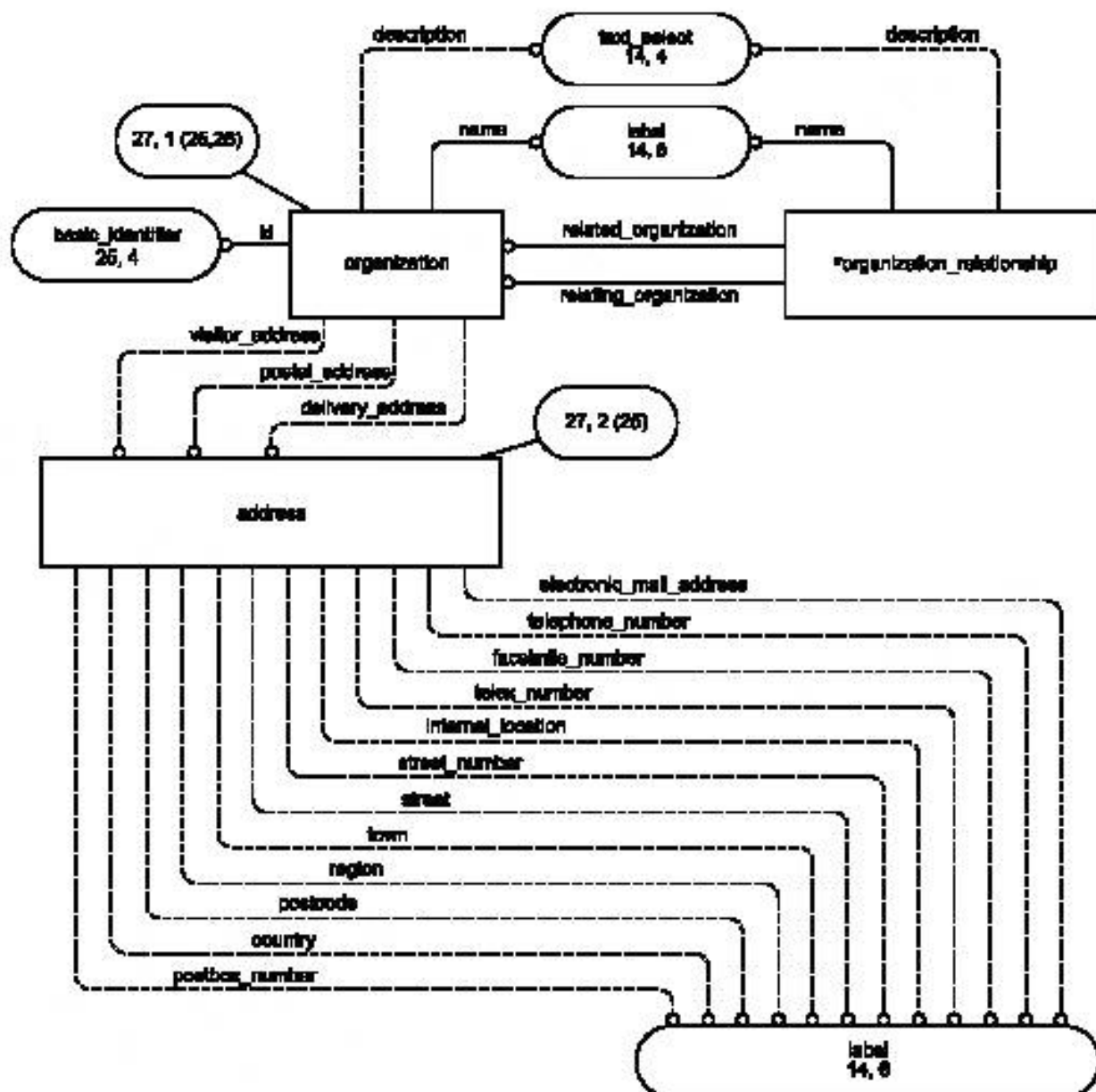
Рисунок E.28 — Диаграмма ссылочной модели приложения на уровне сущности в нотации EXPRESS-G (27 из 41)
