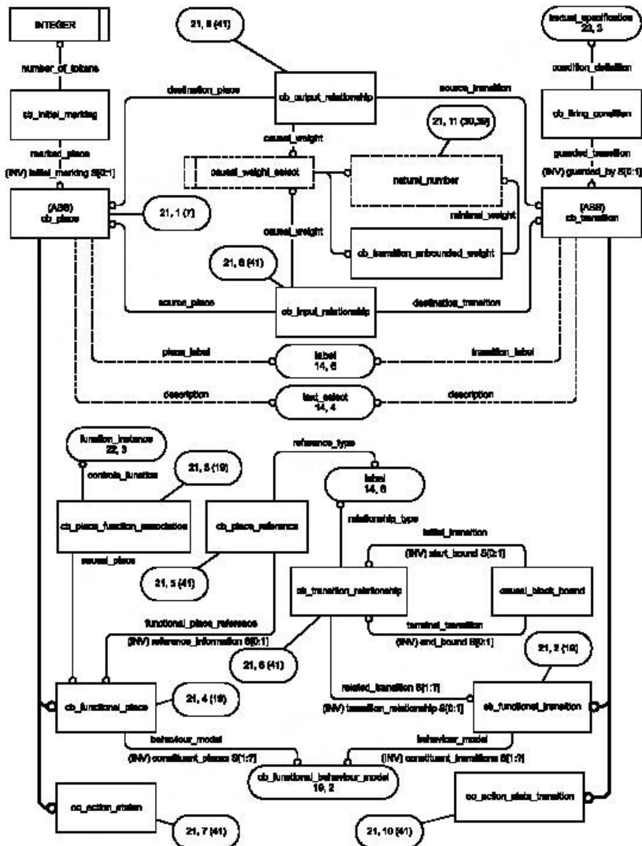
Рисунок Е.22 — Диаграмма ссылочной модели приложения на уровне сущности в нотации EXPRESS-G (21 из 41)
