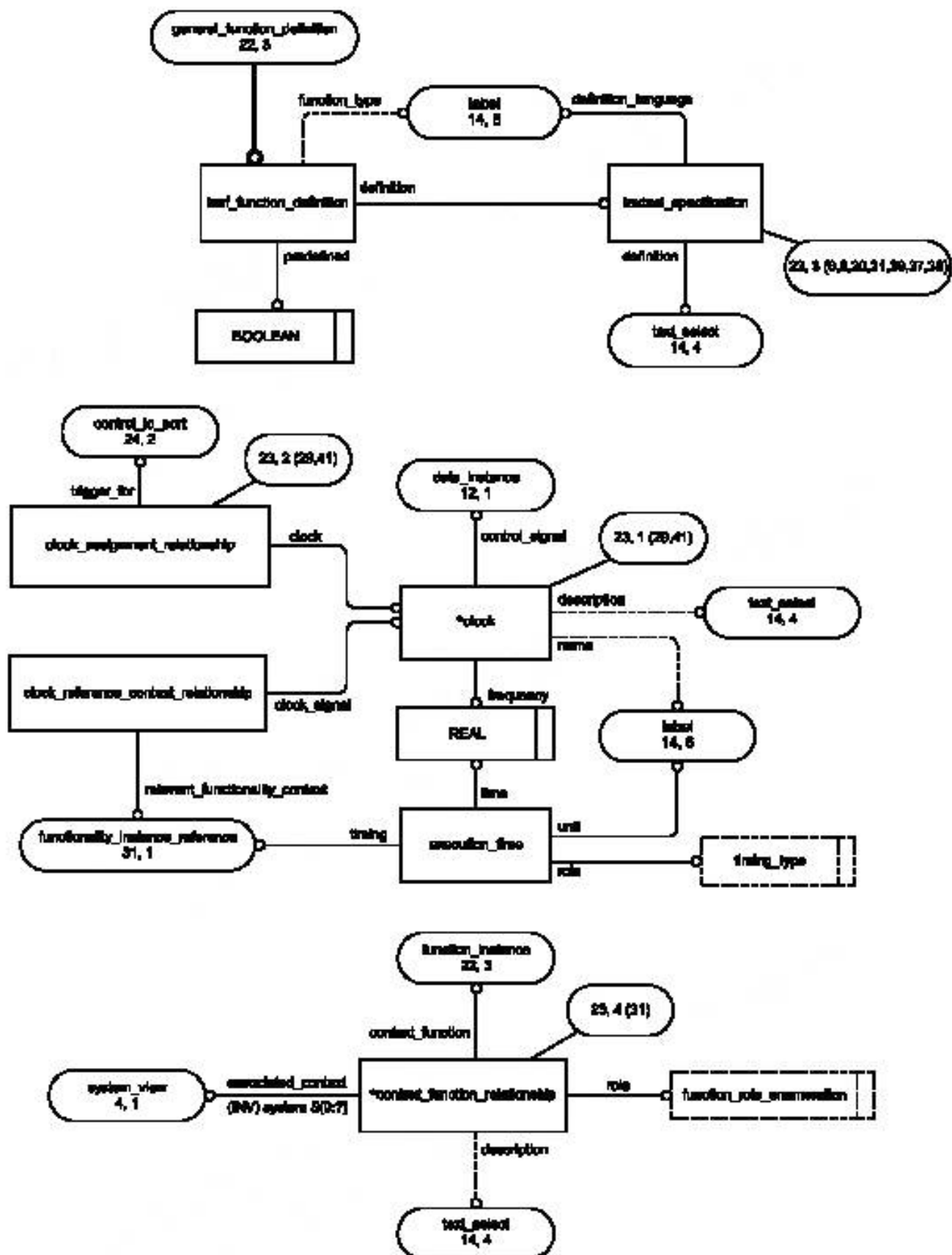
Рисунок Е.24 — Диаграмма ссылочной модели приложения на уровне сущности в нотации EXPRESS-G (23 из 41)
