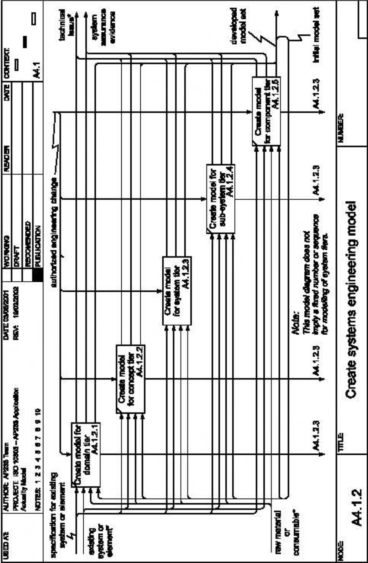
D.6–A4.1.2 Процесс разработки инженерной модели системы
