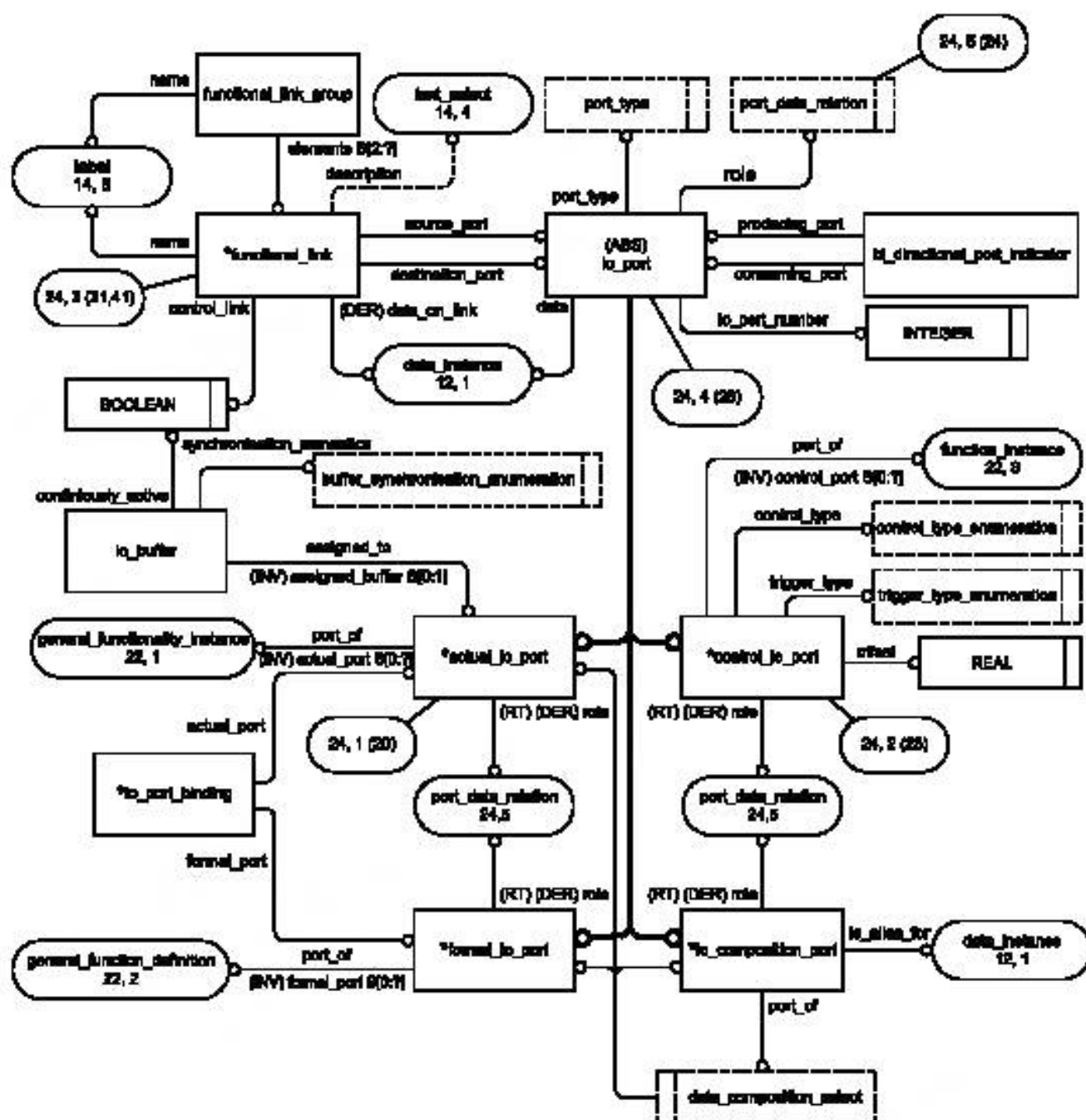
Рисунок E.25 — Диаграмма ссылочной модели приложения на уровне сущности в нотации EXPRESS-G (24 из 41)
