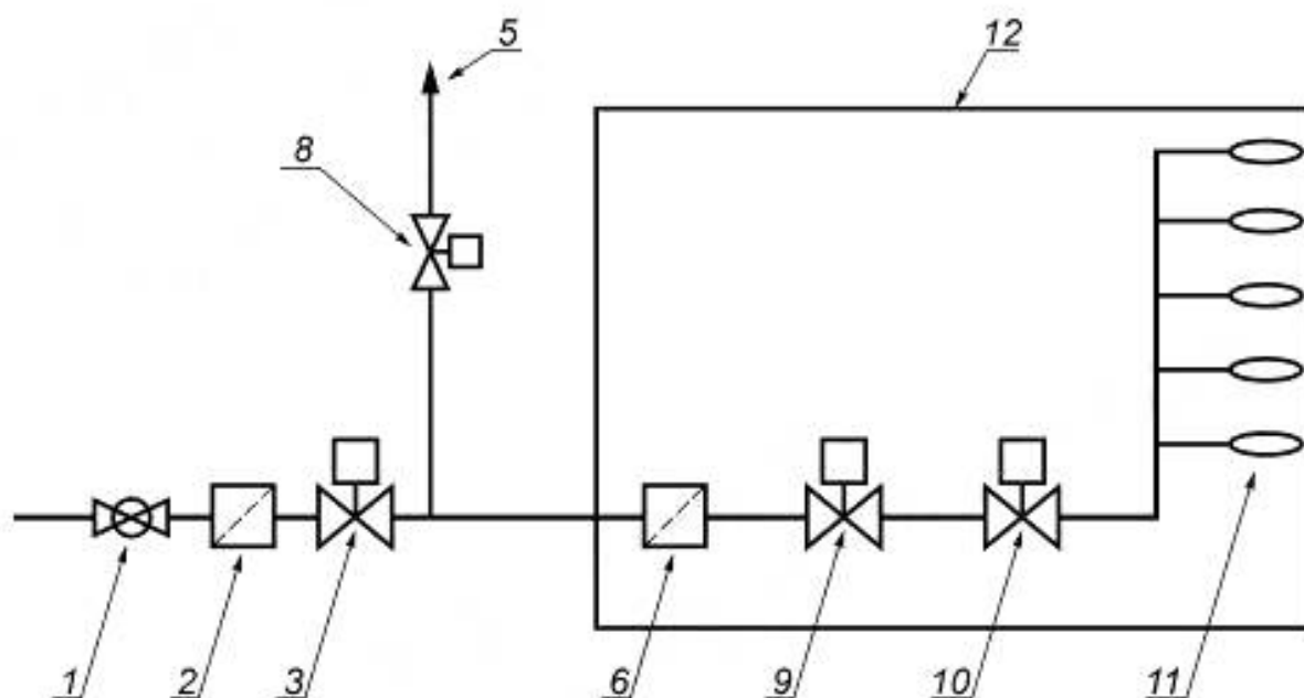
а) Схема с минимальной комплектацией
