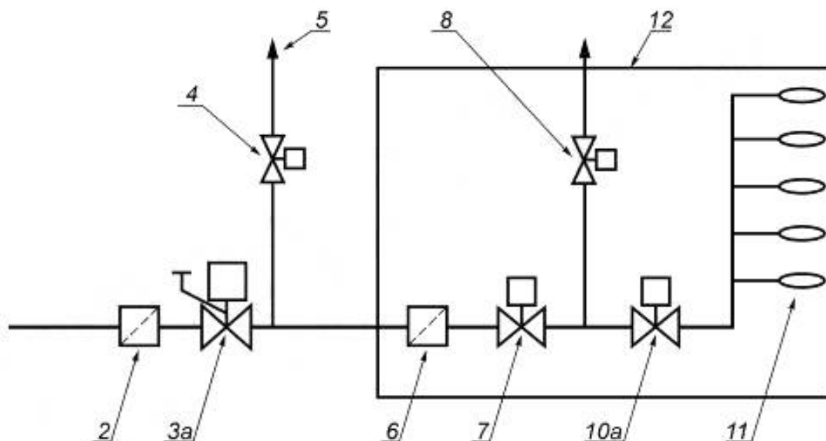
в) Типичная альтернативная схема
