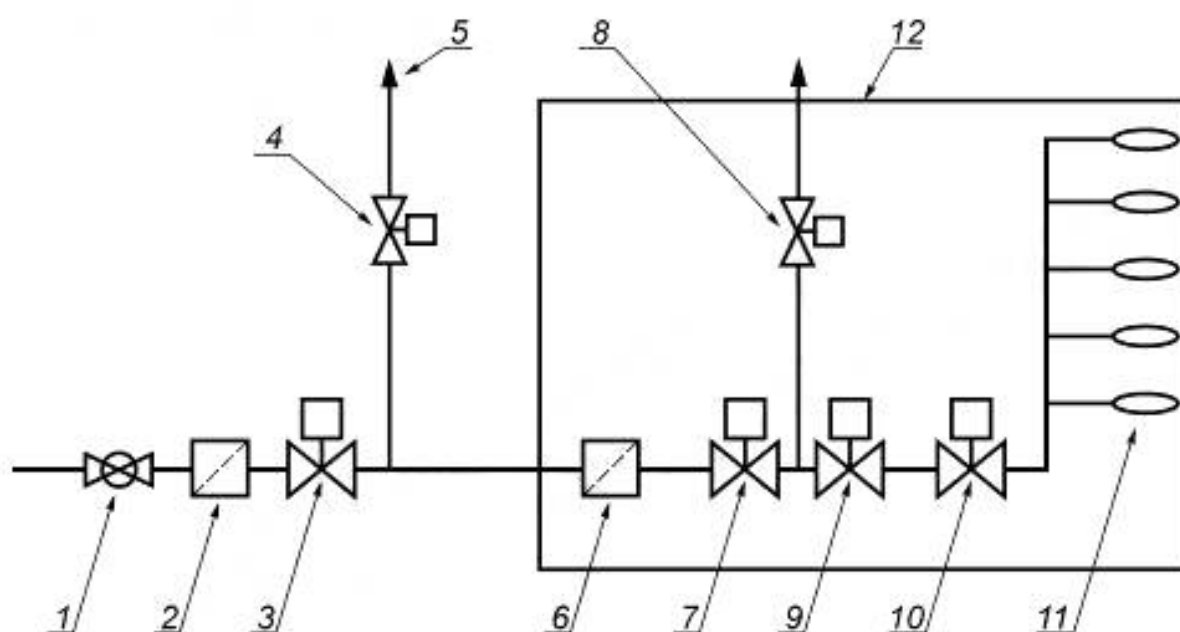
б) Типичная альтернативная схема
