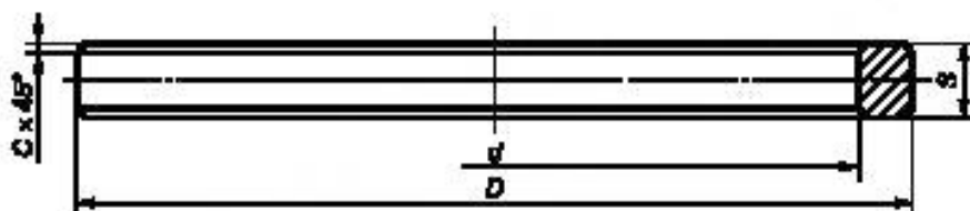
Рисунок 4 — Упорное кольцо
