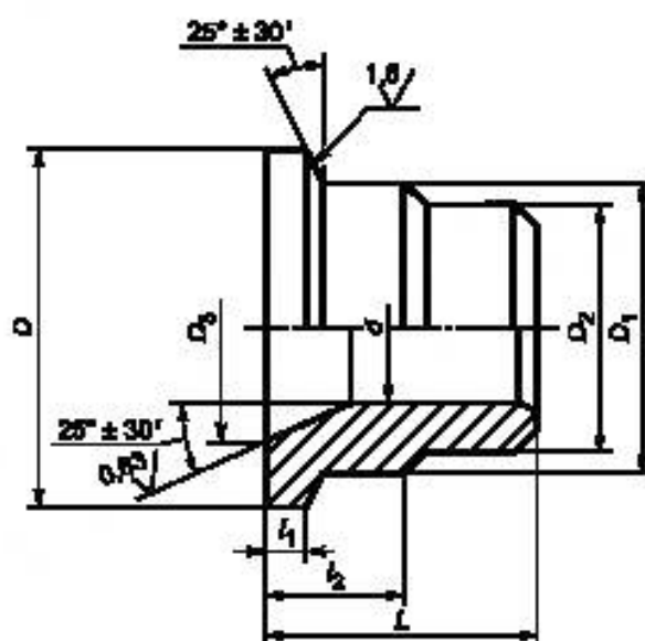
Рисунок 5 — Приварной ниппель
