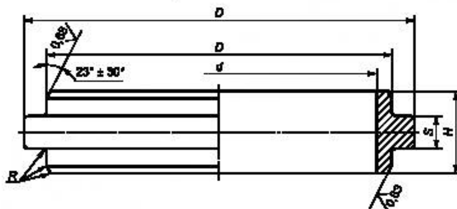
Рисунок 3 — Уплотнительное кольцо
