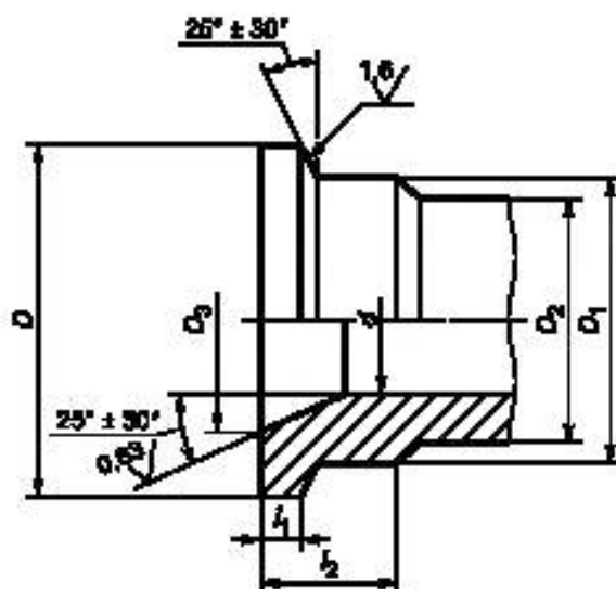
Рисунок 6 — Ниппель неприварной
