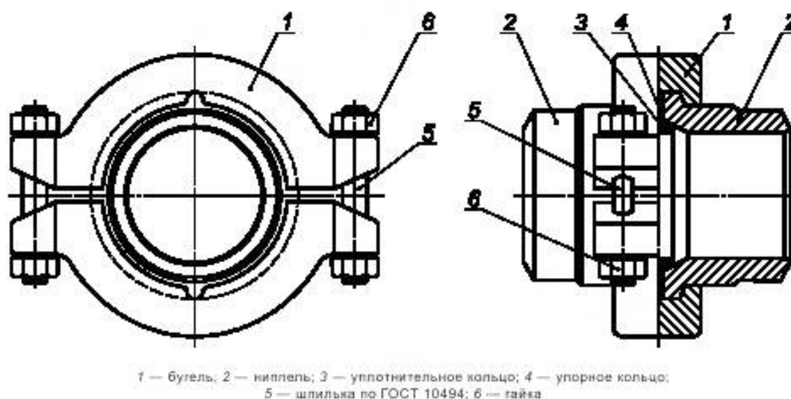
Рисунок 1 — Бугельное разъемное соединение
