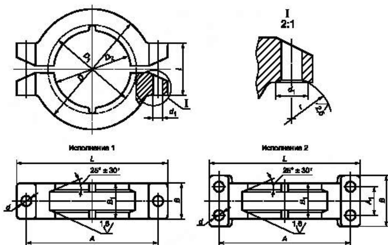
Рисунок 2 — Бугель
