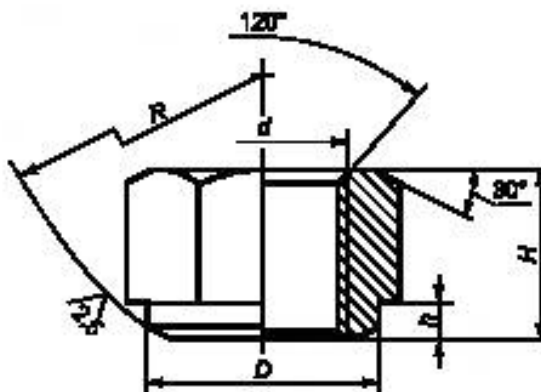
Рисунок 7 — Гайка бугельного разъемного соединения
