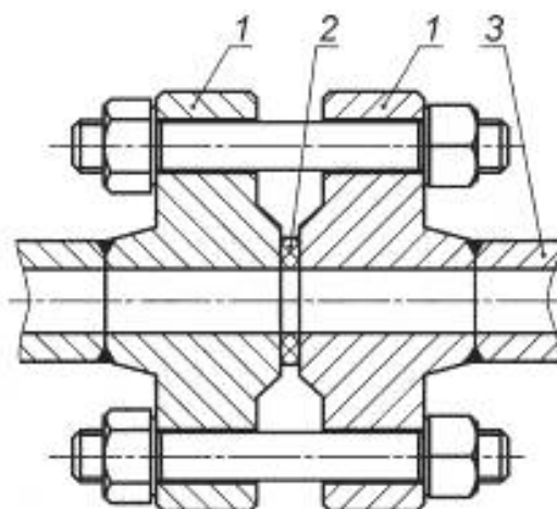
Рисунок 1 — Фланцевое РС с приварными фланцами
