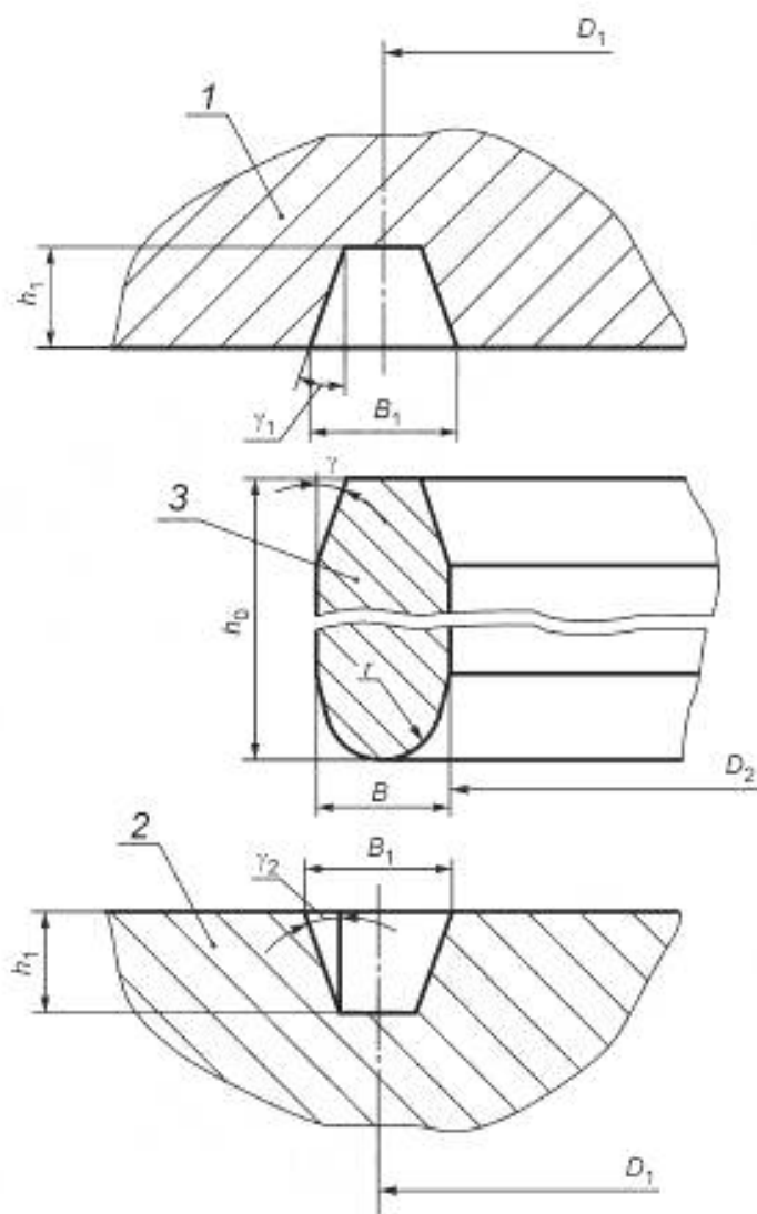
1 — фланец 1; 2 — фланец 2; 3 — прокладка восьмиугольного (овального) сечения
