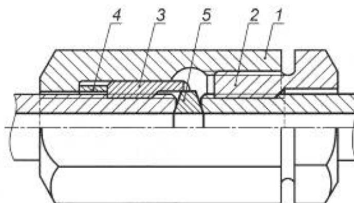
Рисунок 2 — Фланцевое РС с резьбовыми фланцами
