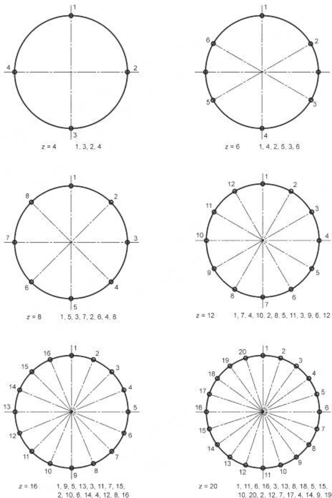
Рисунок М.2 — Схемы перестановки ключа при затяжке шпилек разъемных соединений с различным количеством шпилек z
