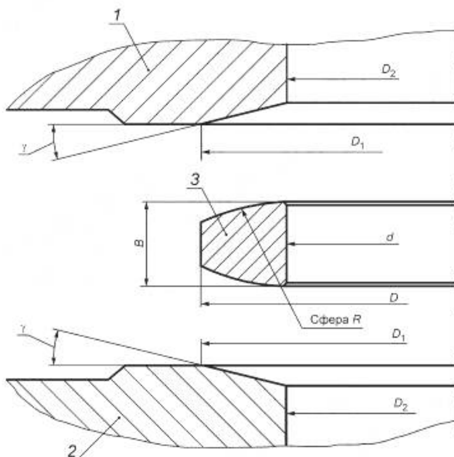
1 — фланец 1; 2 — фланец 2; 3 — сферическая линза
