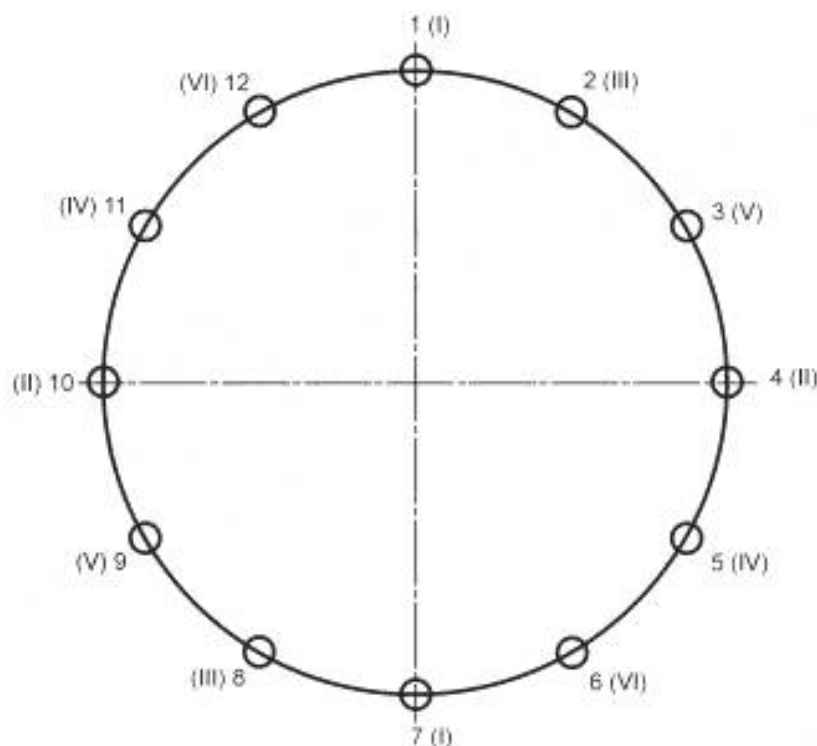
Рисунок М.1 — Схема перестановки ключа (обход)
