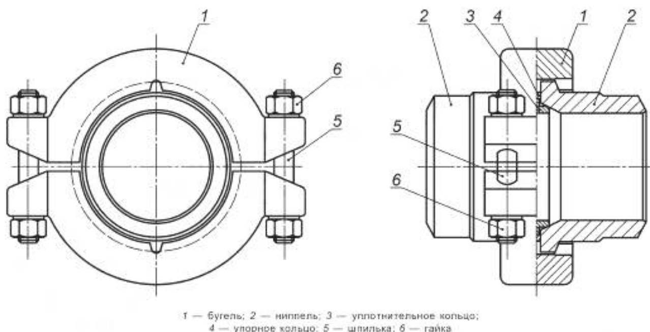
Рисунок 4 — Бугельное РС (ГОСТ Р 55429)
