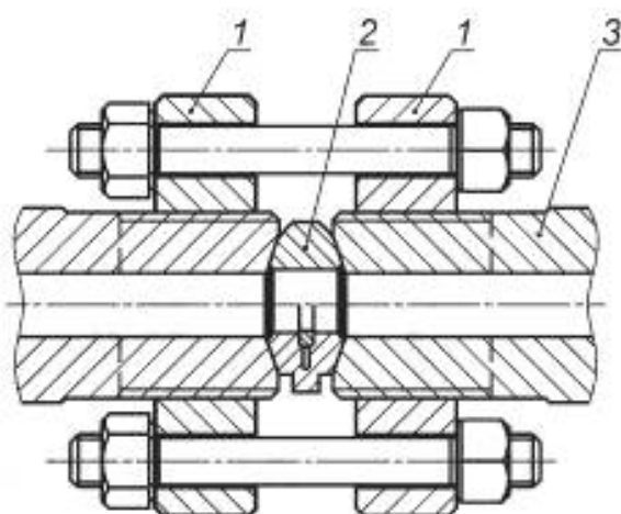
Рисунок 1 — Фланцевое РС с приварными фланцами
