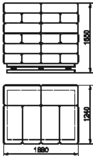
Рисунок 6 — Пакет груза в мешках на поддоне
