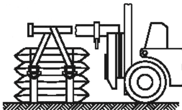
Рисунок 10 — Транспортировка груза погрузчиком со штыревым захватом
