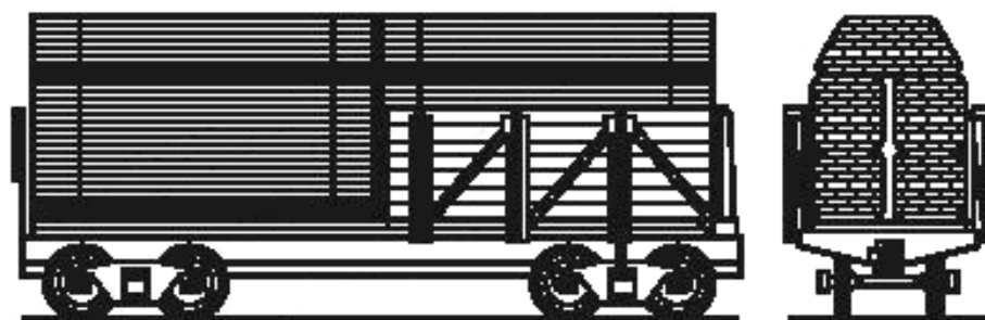
Рисунок 11 — Схема размещения груза в полувагоне
