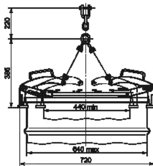
Рисунок 4 — Пример изображения грузозахватного приспособления
