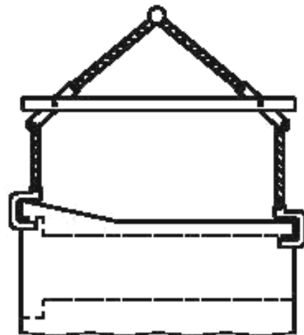
Рисунок 8 — Схема строповки железобетонной трубы
