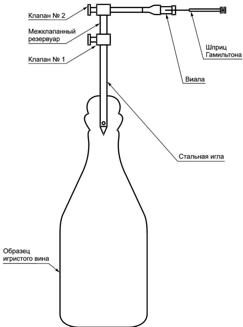
Рисунок А.1 — Схема приспособления для отбора проб
