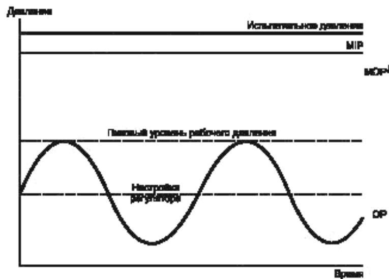
Рисунок 1 — Соотношение давлений
