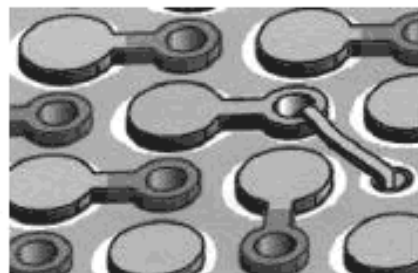
Рисунок 44 б – Установка медной перемычки из фольги в тefлоновую трубку и металлизированное отверстие
