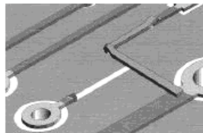
Рисунок 19 d – Перегиб широкого проводника
