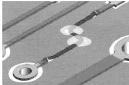
Рисунок 21 e – Приклеивание провода к поверхности платы клеем
