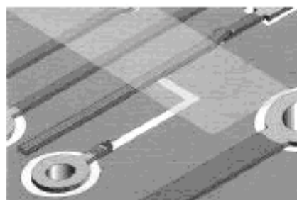
Рисунок 19 b – Установка перемычки из фольги, фиксация положения липкой лентой
