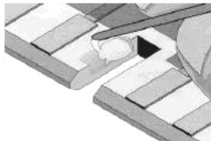
Рисунок 14 б – Нанесение эпоксидного состава на кромки прорези
