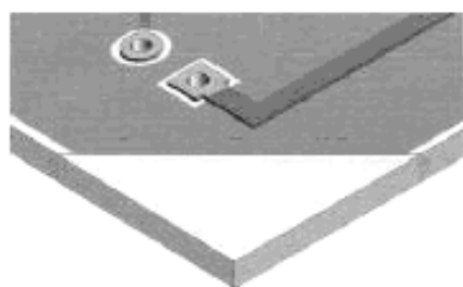
Рисунок 11 с – Фрезерование уступа в кромке имплантанта
