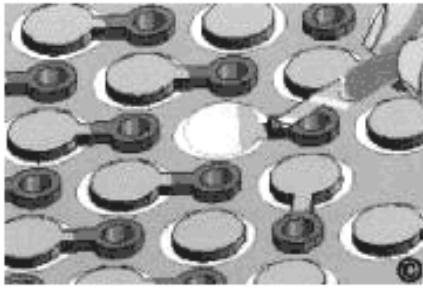
Рисунок 42 а – Удаление поврежденной контактной площадки
