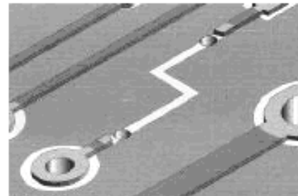
Рисунок 22 b – Сверление сквозных отверстий рядом с проводником
