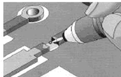
Рисунок 26 б – Пропил для размыкания печатного проводника
