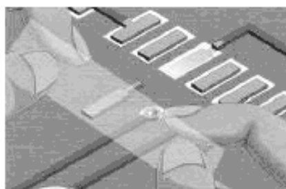
Рисунок 38 e – Установка новой контактной площадки с помощью липкой ленты
