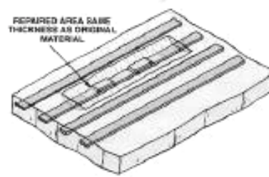
Рисунок 24 х – Герметизация отреставрированного участка
