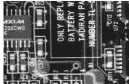
Рисунок 45 d – Приклеивание провода кусочками липкой ленты
