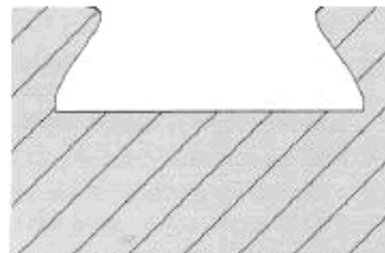
Рисунок 9 б – Подрез для увеличения механической прочности
