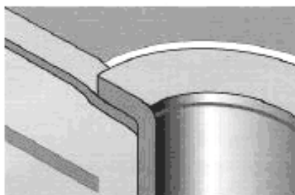
Рисунок 39 а – Зажатие фланцем пистона нового печатного проводника
