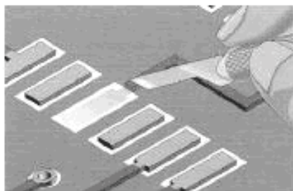
Рисунок 37 а – Удаление площадки
