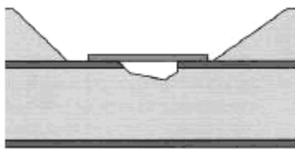
Рисунок 25 с – Перемычка из фольги, установленная по месту
