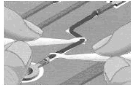
Рисунок 21 d – Припаивание второго конца провода по месту
