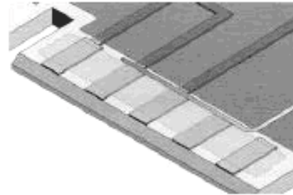
Рисунок 36 д – Припаивание провода по кромке металлизированных концевых контактов
