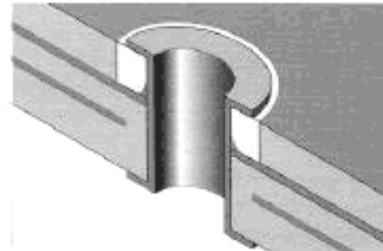
Рисунок 41 d – пистона, расклепанная вровень с поверхностью платы
