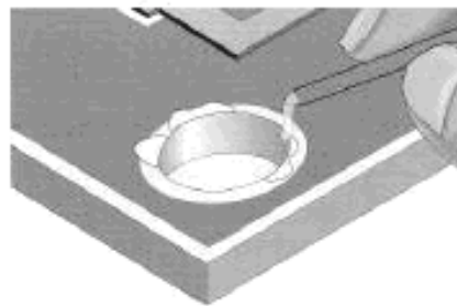
Рисунок 13 б – Введение эпоксидного состава заостренной деревянной палочкой
