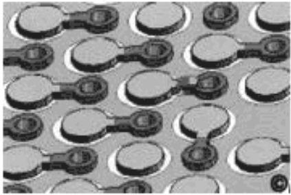
Рисунок 42 с – Удаление припоя с присоединяемого проводника
