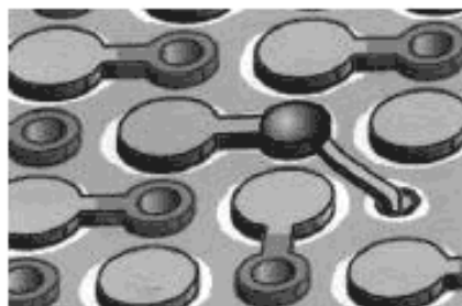
Рисунок 44 с – Припайвание перемычки из фольги к металлизированному отверстию, соединенному площадкой BGA
