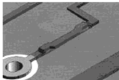
Рисунок 20 ф – Завершенный ремонт
