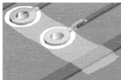
Рисунок 33 д – Установка новой контактной площадки с помощью липкой ленты
