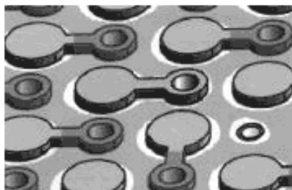
Рисунок 44 а – Фрезерование в плате сквозных отверстий и установка тefлоновой трубки
