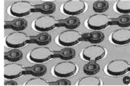
Рисунок 42 д – Покрытие паяных соединений эпоксидным составом
