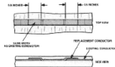
Рисунок 24 ф – Технические данные по замене
