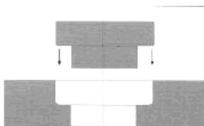
Рисунок 10 с – Создание уступа в кромке печатной платы
