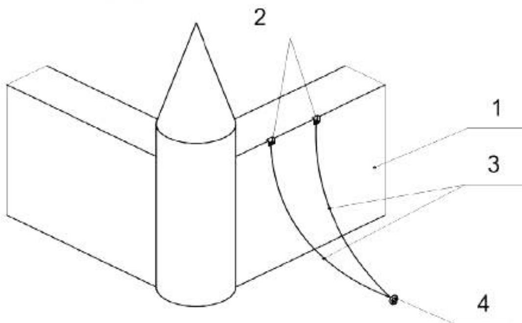
1 — сторона батута; 2 — узлы крепления; 3 — швартовочные элементы (условно показаны с провисом); 4 — один стержень или одна точка балластной системы
