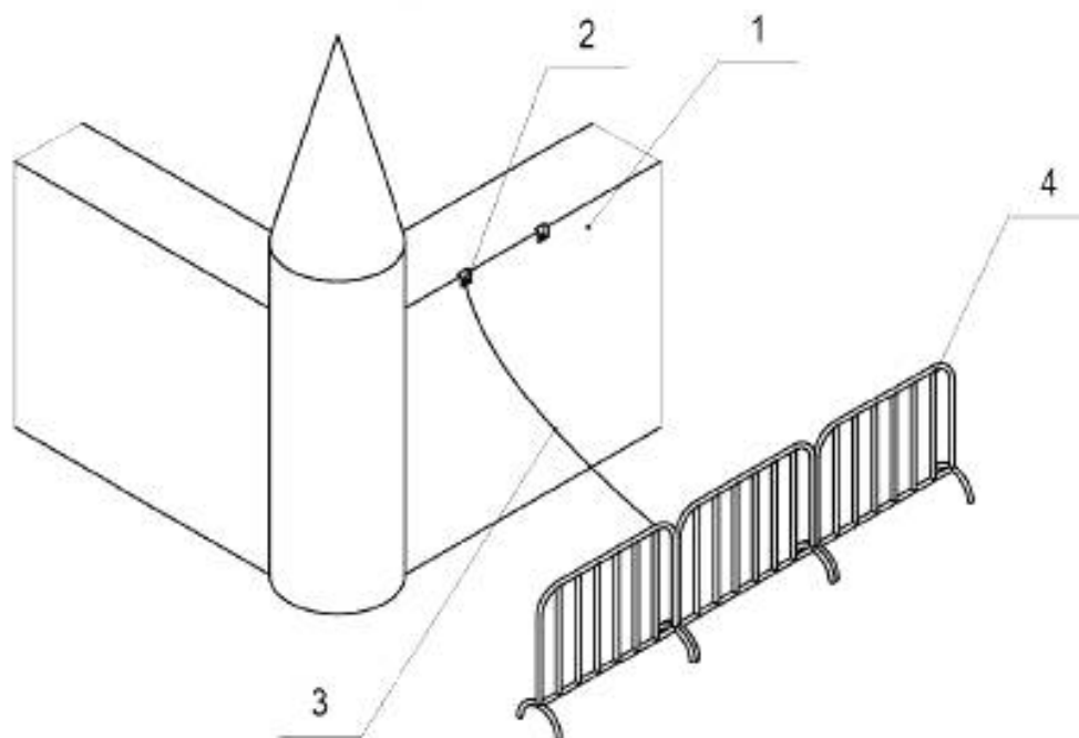
1 — сторона батута; 2 — узел крепления; 3 — швартовочный элемент (условно показан с провисом); 4 — система ограничения доступа
