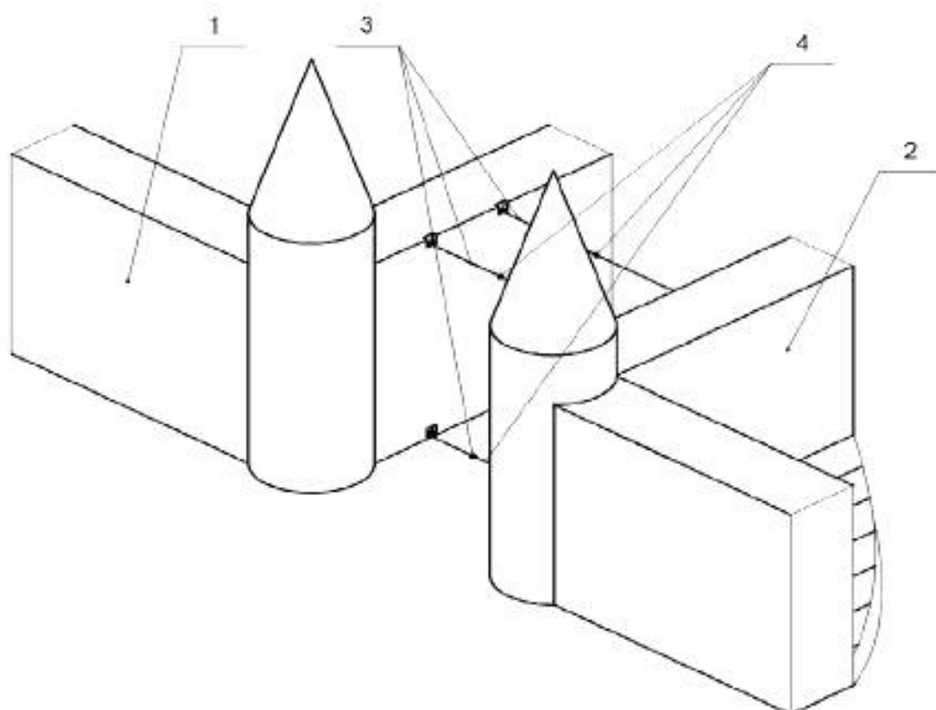
1 — первый батут; 2 — второй батут; 3 — швартовочные элементы первого батута; 4 — швартовочные элементы второго батута
