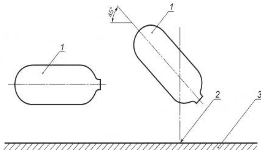
1 — испытываемый баллон; 2 — точка соударения; 3 — испытательная плита
