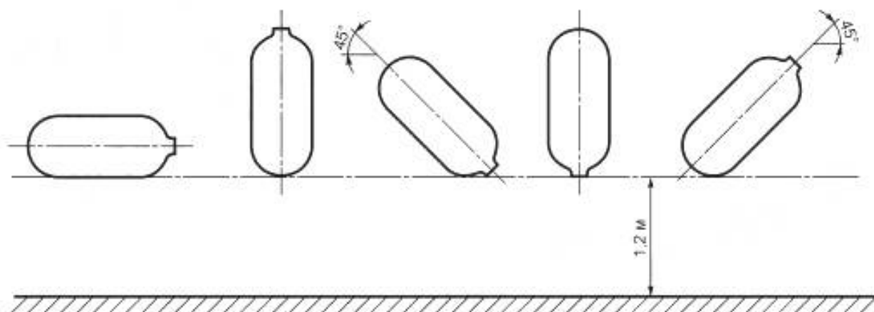
Рисунок 5 — Ориентация баллона при испытании
