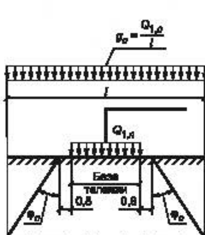
б) Схема распределения нагрузки вдоль грузового причала от ноги крана
