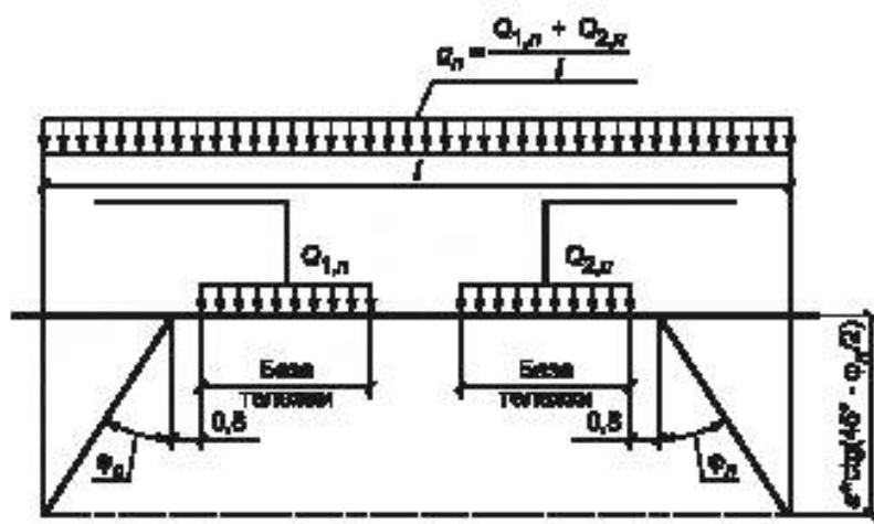
в) Схема распределения нагрузок вдоль грузового причала от двух ног максимально сближенных кранов (размеры в метрах)
