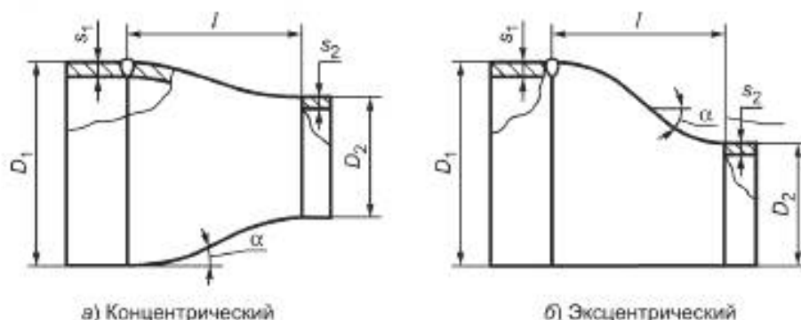
Рисунок 7.2 — Переходы
