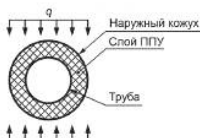
Рисунок 12.1 — К определению жесткости поперечного сечения на изгиб
