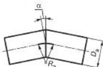
Рисунок 8.8 — Косой стык
