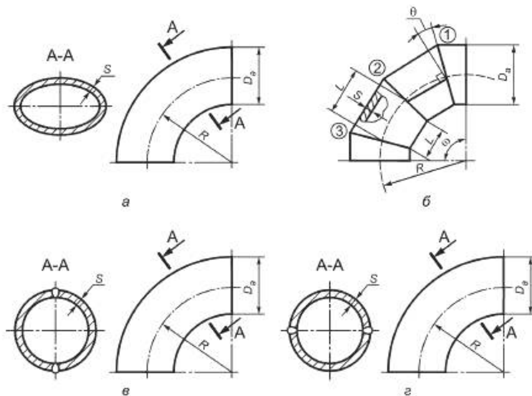
а — глухой; б — секторный с тремя косыми стыками ( n = 3 ); в, г — штампованной
