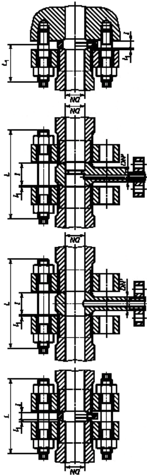
Рисунок Е.1 — Длина шпилек фланцевых соединений
