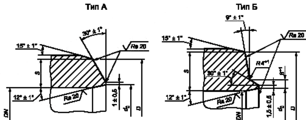
Рисунок Д.1 — Разделка концов труб и деталей трубопроводов под сварку
