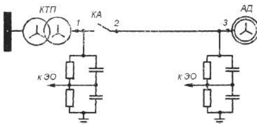
Схема коммутации низкого напряжения
