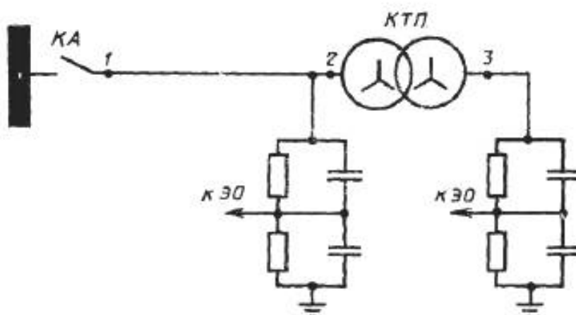
Схема коммутации низкого напряжения
