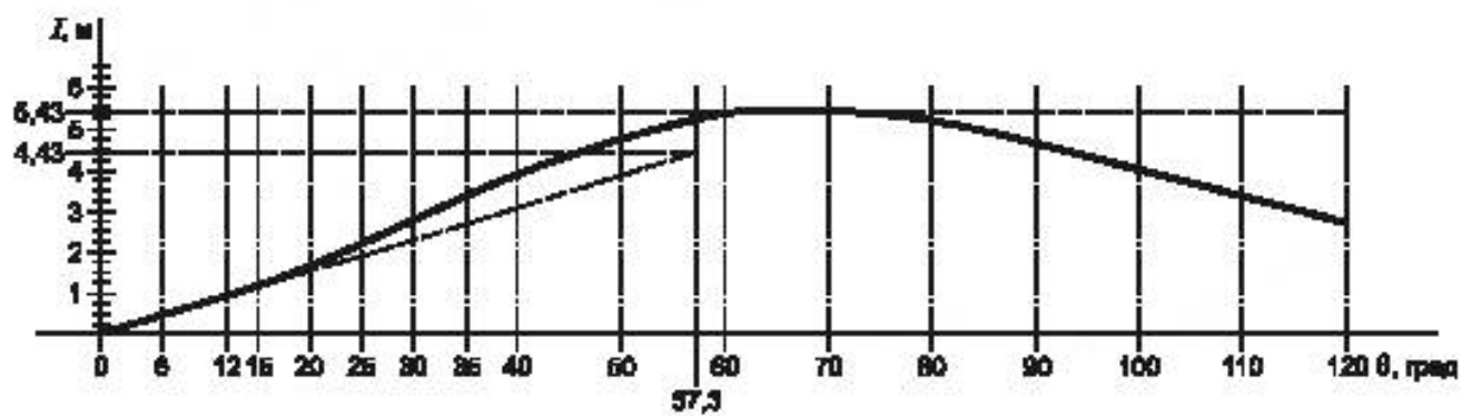
Рисунок К.12 — Диаграмма статической остойчивости
