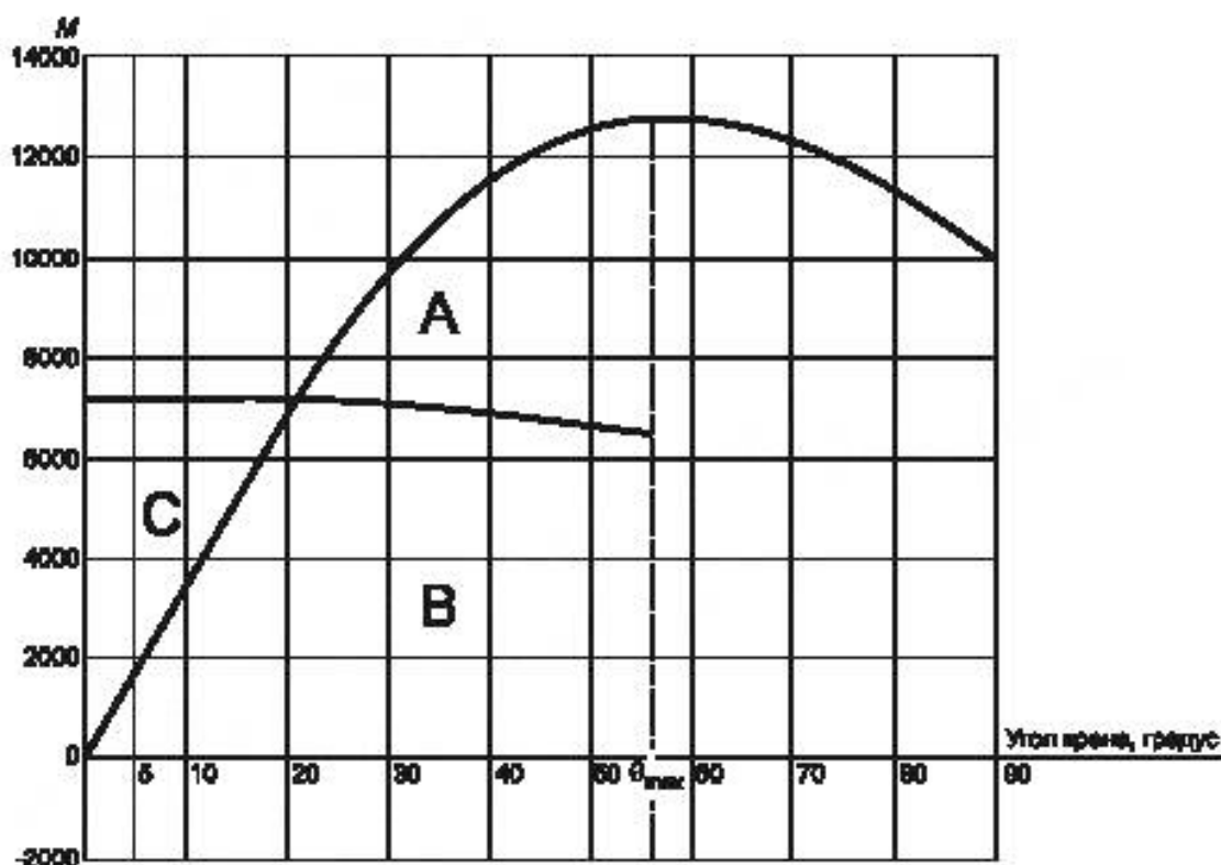
Рисунок 1 — Диаграмма статической устойчивости
